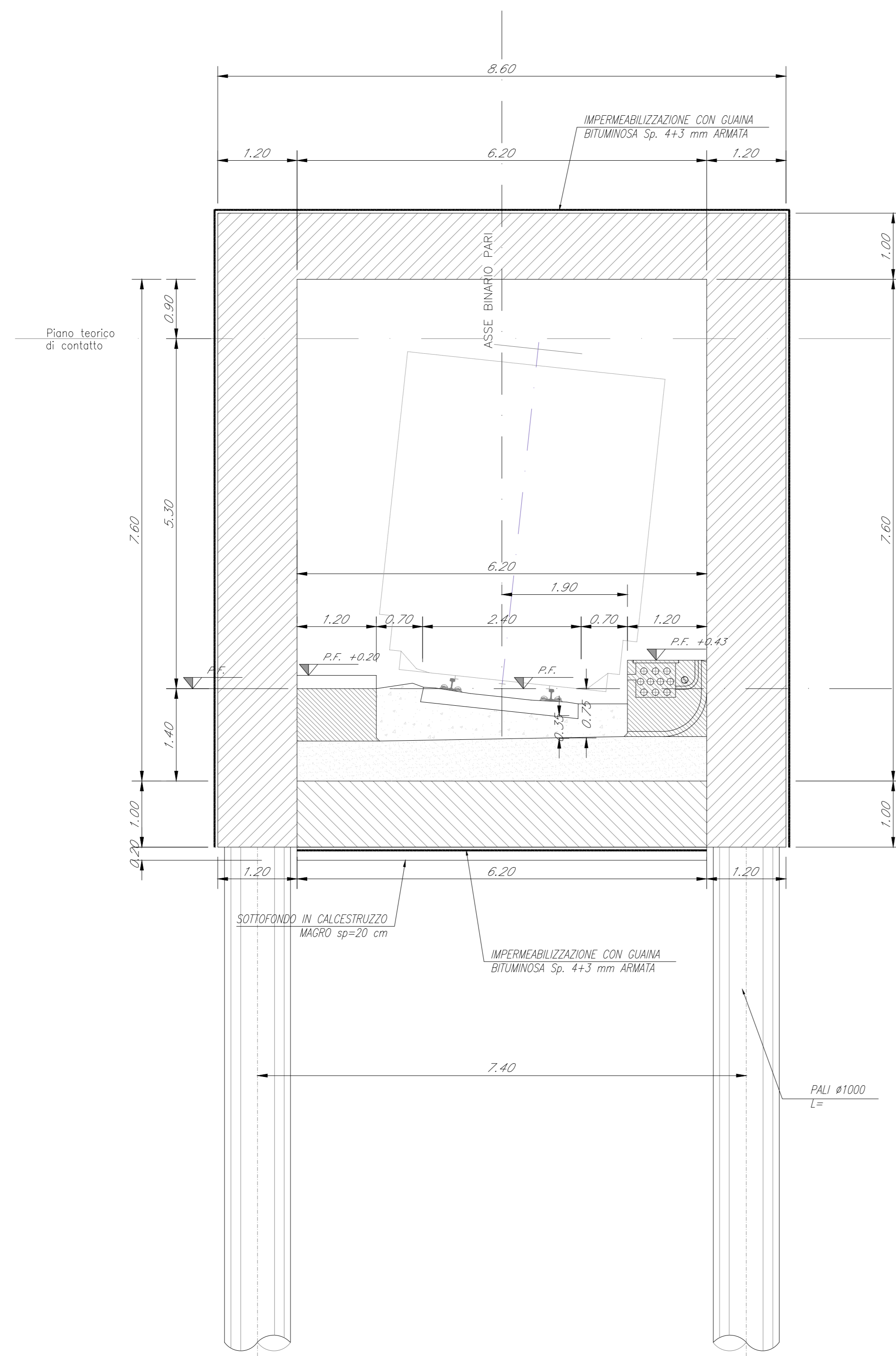
SEZIONE TIPO GALLERIA ARTIFICIALE IMBOCCO scala 1:50
