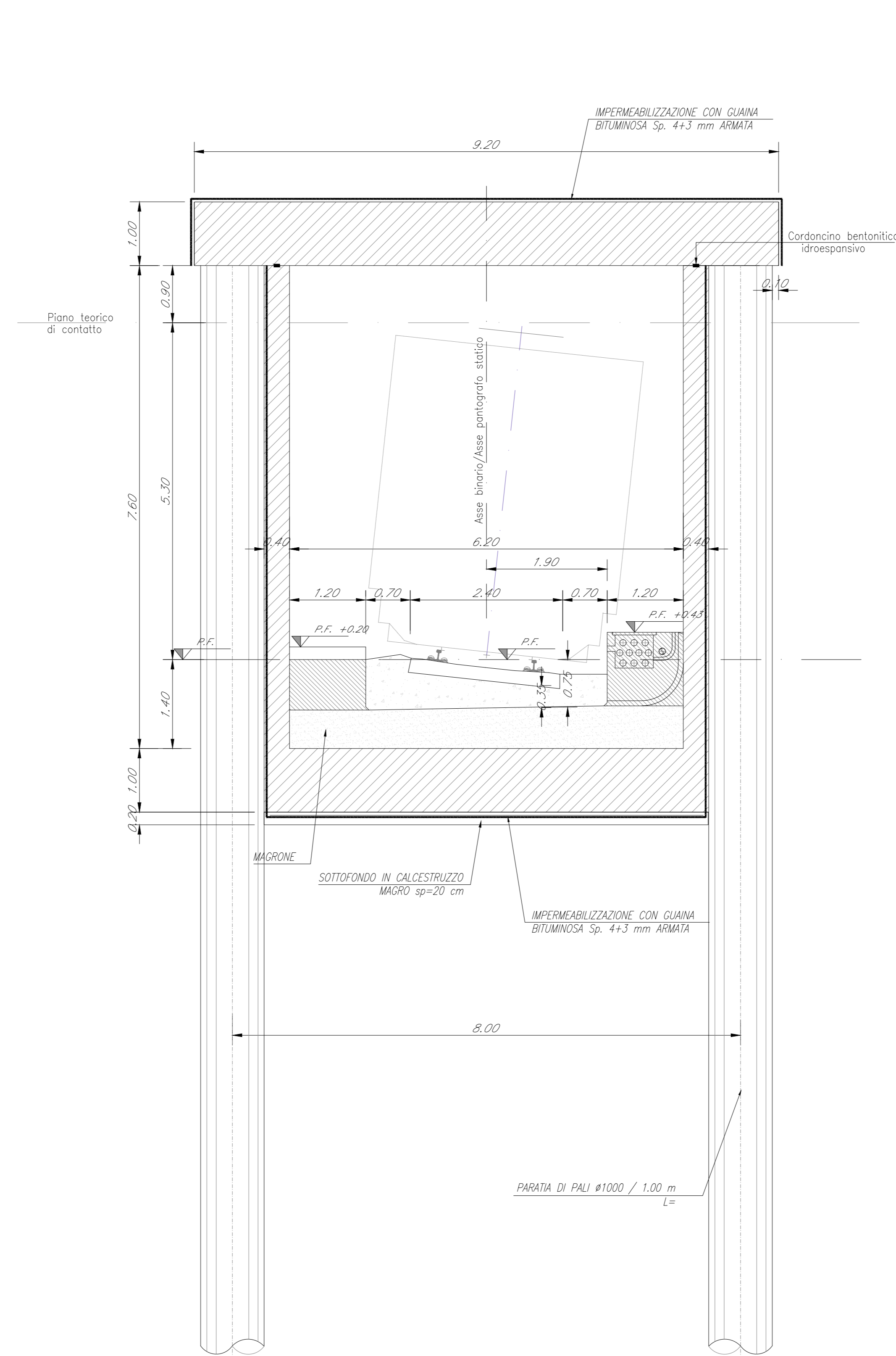
SEZIONE TIPO GALLERIA ARTIFICIALE CON PALI scala 1:50
