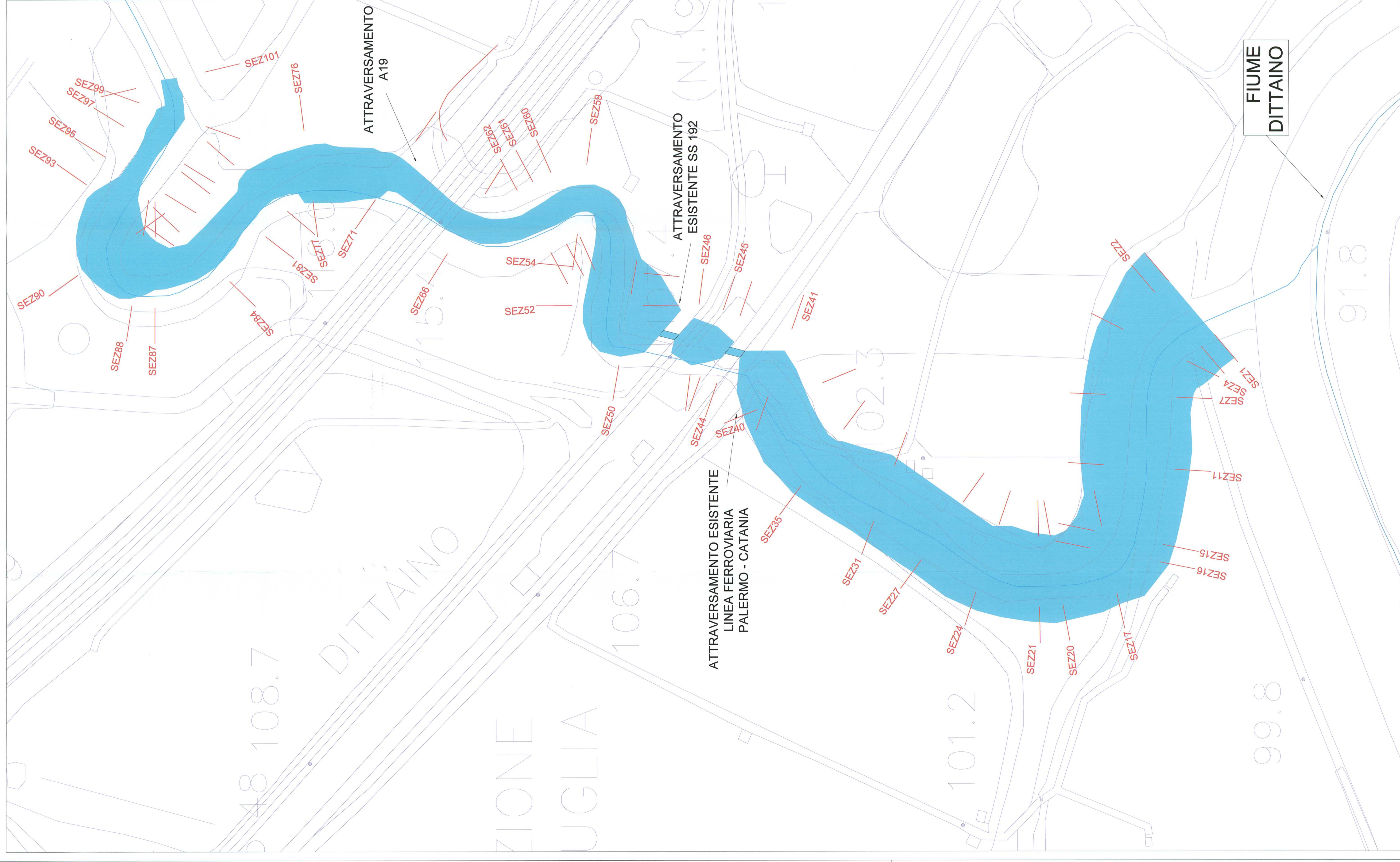
VALLONE ARANCIARO ANTE OPERAM Scala 1:1'000
