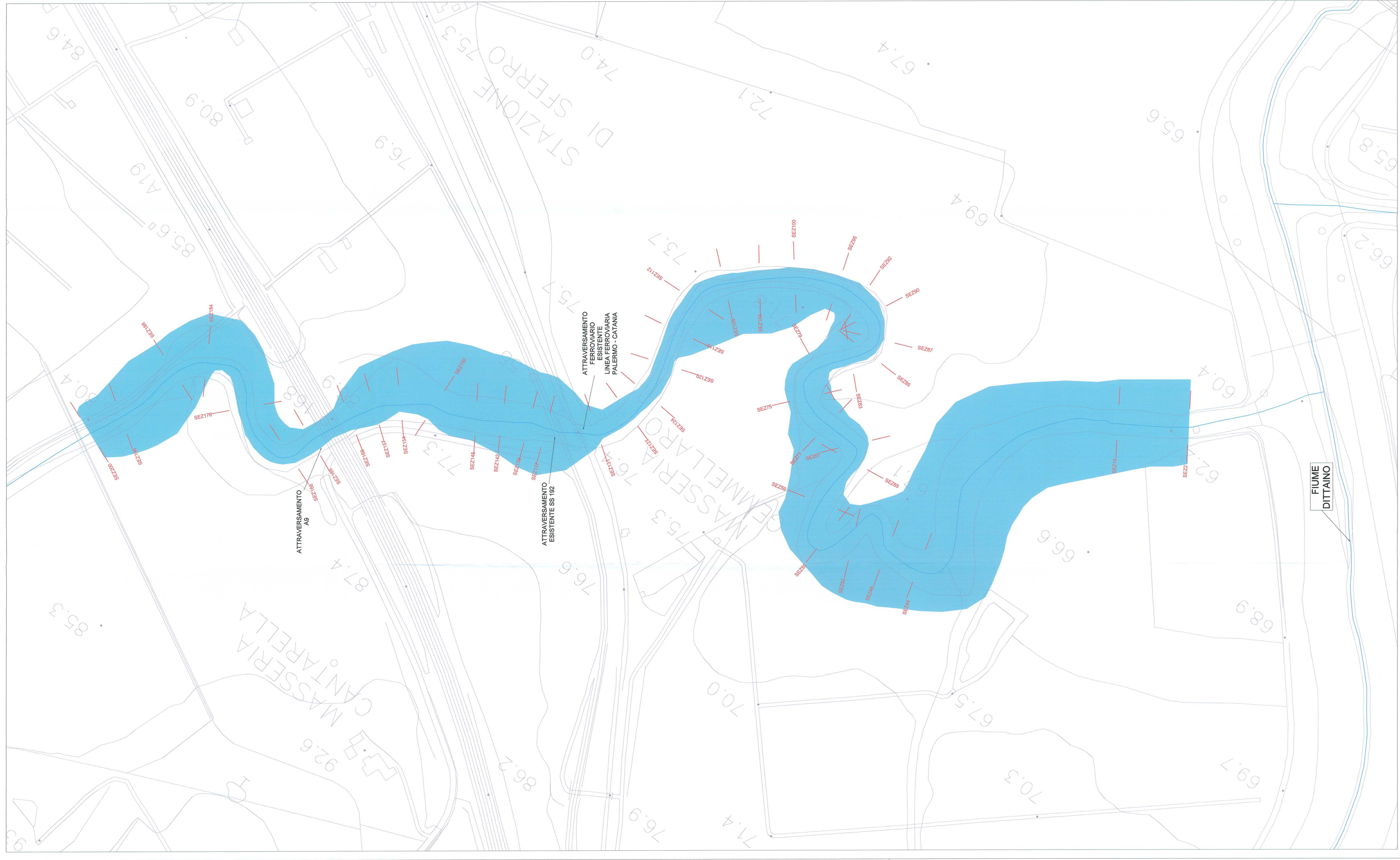
VALLONE SFERRO ANTE OPERAM Scala 1:2000
