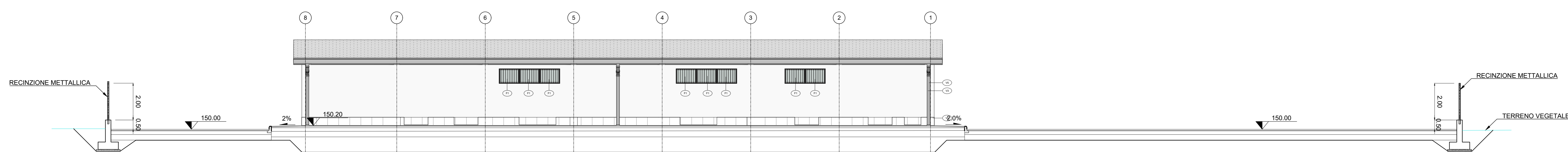
SEZIONE A-A PIAZZALE scala 1:100
