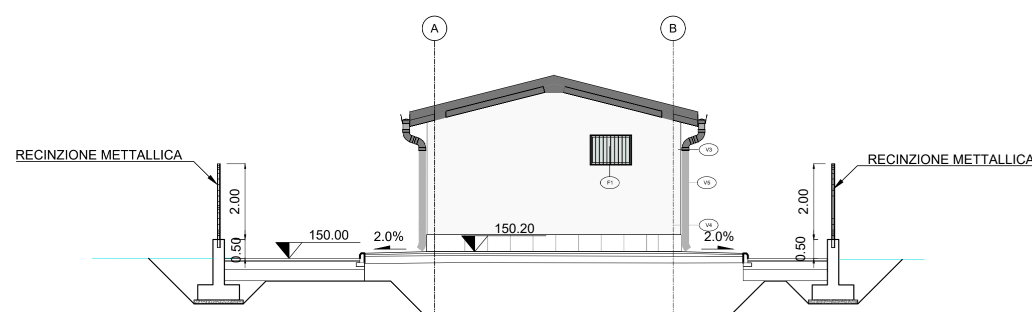
SEZIONE B-B PIAZZALE scala 1:100
