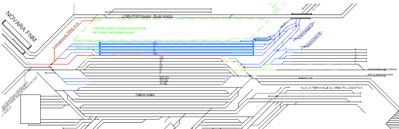
FIGURA 17 MACROFASE 3 - INTERVENTI NELLO SCALO DI NOVARA BOSCHETTO (NUOVO FASCIO HUCKEPACK)
