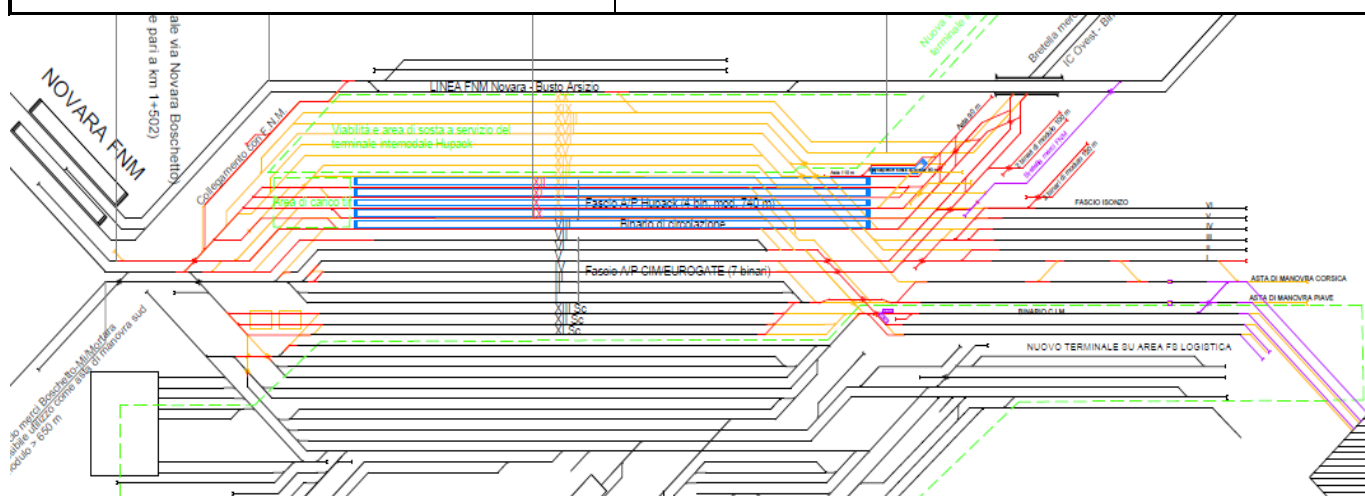
FIGURA 8 SCHEMATICO DI PROGETTO DELLO SCALO DI NOVARA BOSCHETTO
