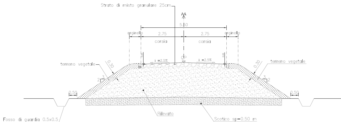
FIGURA 27 VIABILITÀ NV05 - SEZIONE TIPO IN RILEVATO
