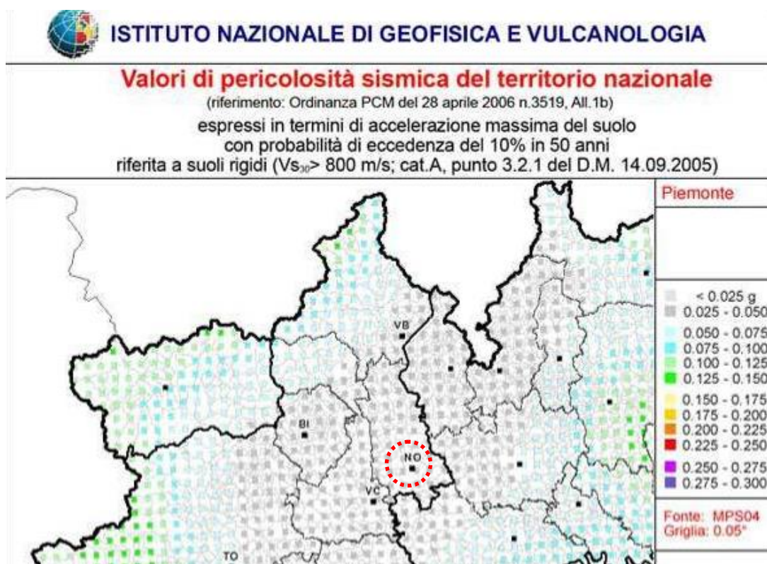
Figura 8-2. Mappa di pericolosità sismica espressa in termini di accelerazione massima del suolo ( a_{max} ) con probabilità di eccedenza del 10% in 50 anni riferita a suoli molto rigidi ( V_{s,30} > 800 m/s) – da INGV.
