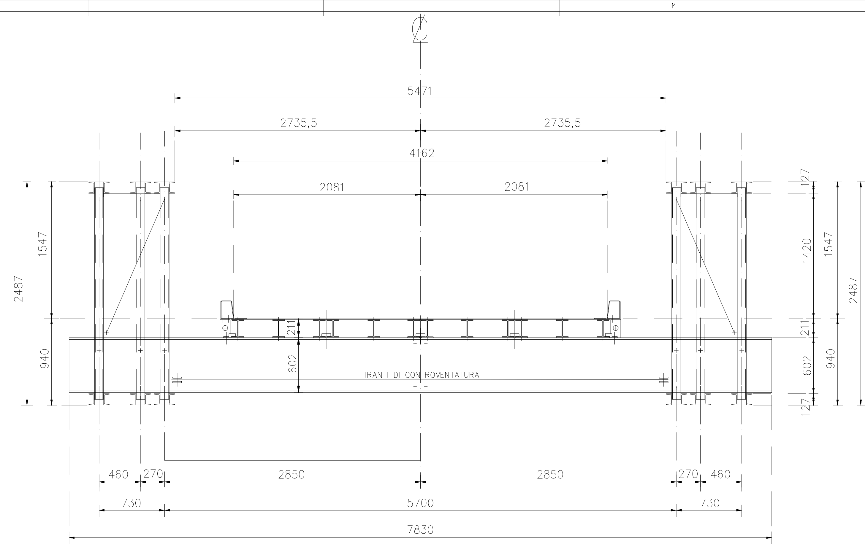
SEZIONE TRASVERSALE IN ZONA CENTRALE
