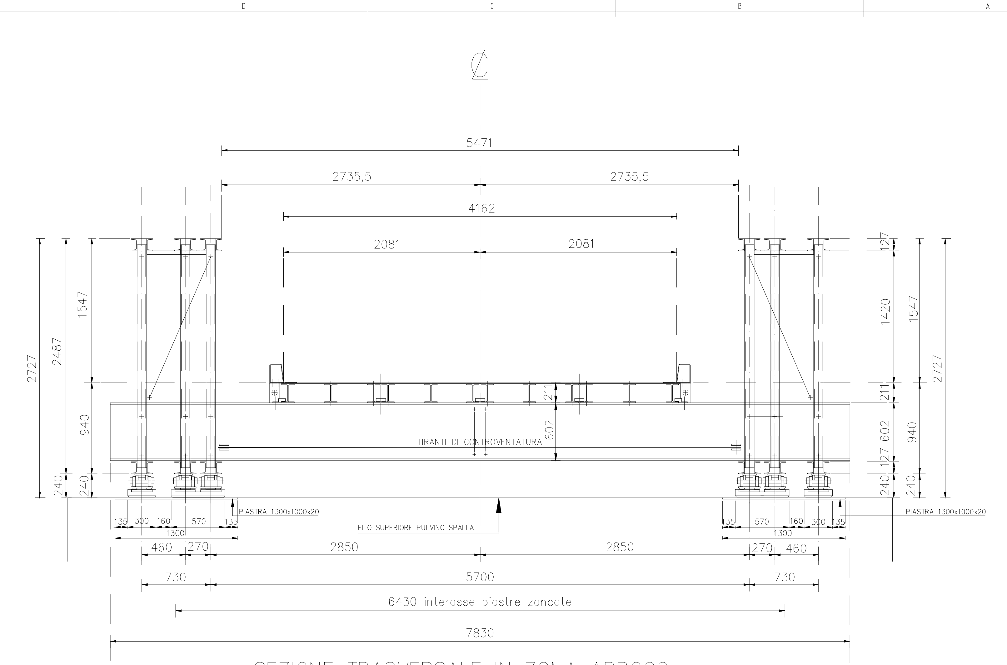
SEZIONE TRASVERSALE IN ZONA APPOGGI
