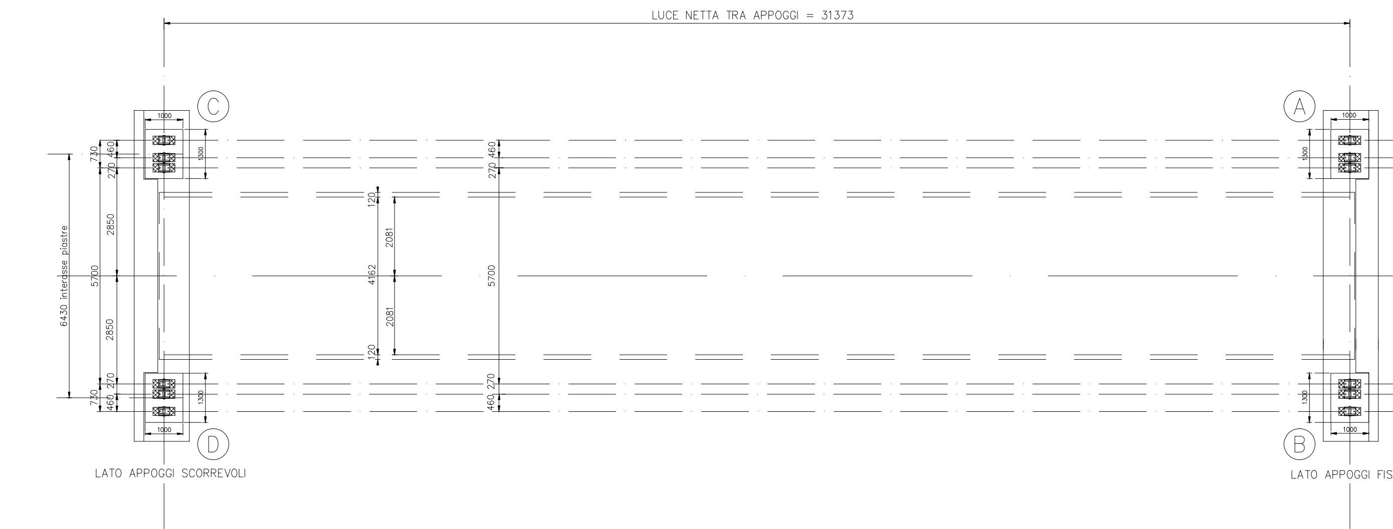
PIANTA CON AZIONI SULLE FONDAZIONI
