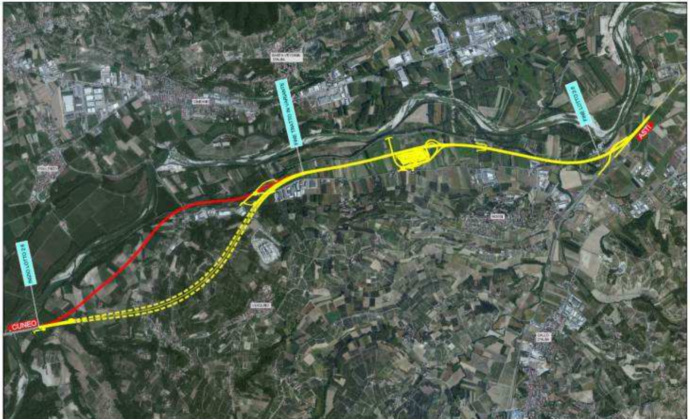
COMPLETAMENTO AUTOSTRADA A33 Confronto Tracciato all’aperto - Tracciato in galleria
