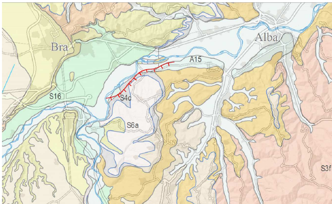
Fig.3. Carta geologica del Piemonte (fonte ARPA Piemonte) con sovrapposto in rosso il tracciato del lotto 2.6a
