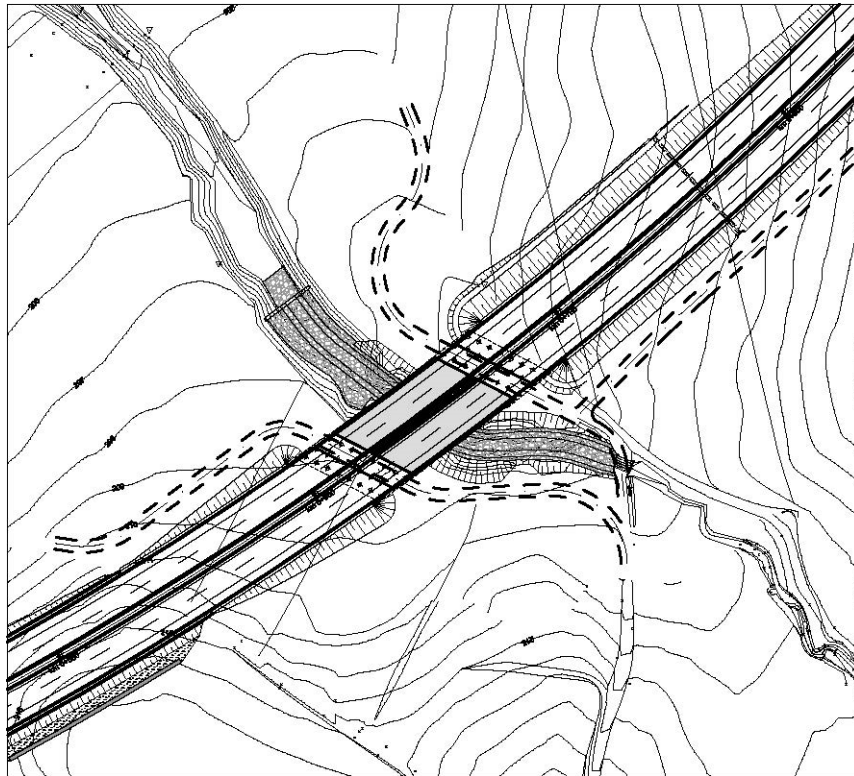
Fig.6. Attraversamento del Rio San Giacomo nel PFTE
