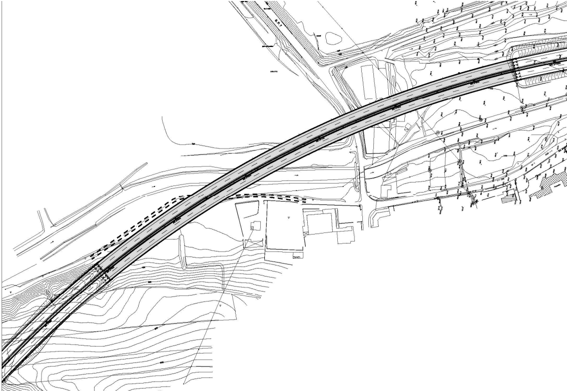
Fig.8. Viadotto Verduno nel PFTE
