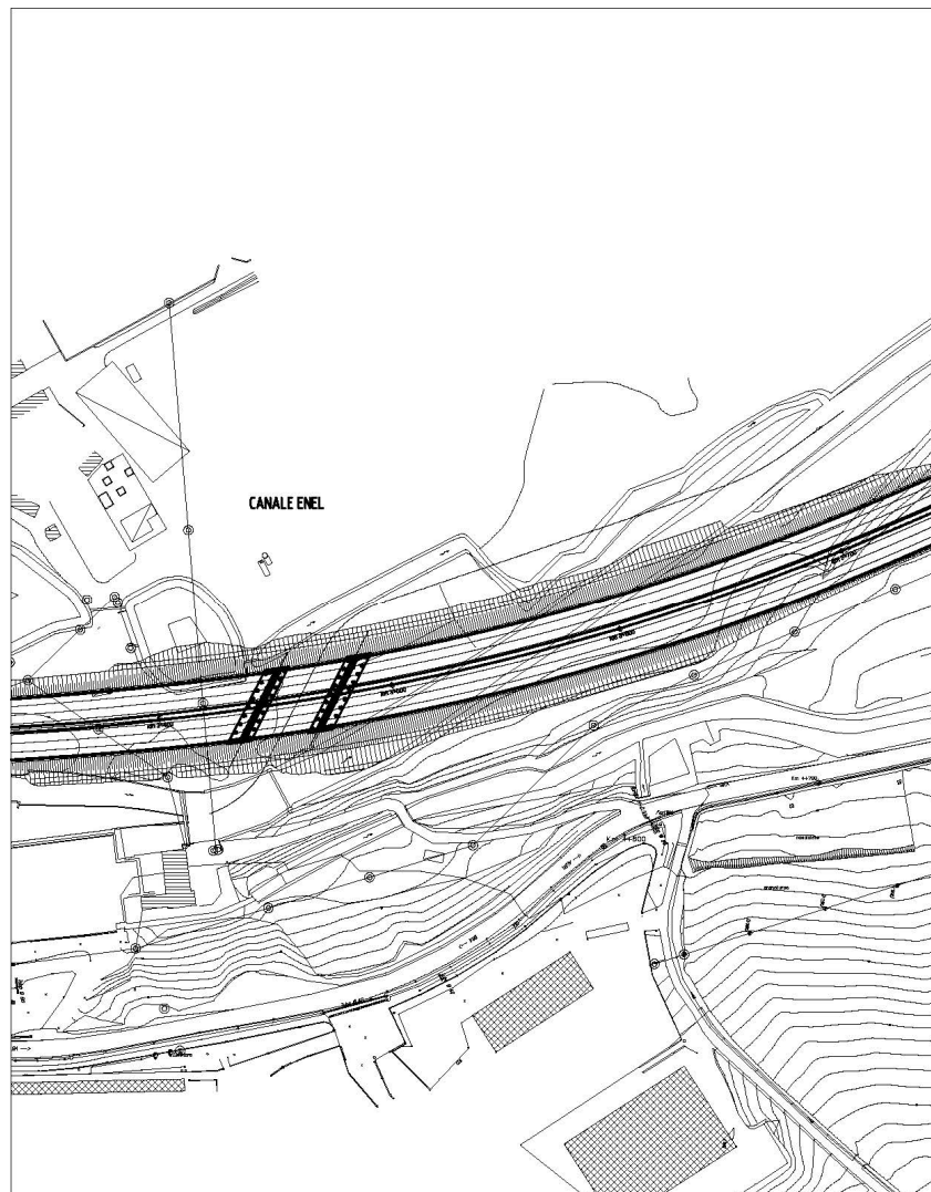
Fig.5. Attraversamento del canale Enel nel PD
