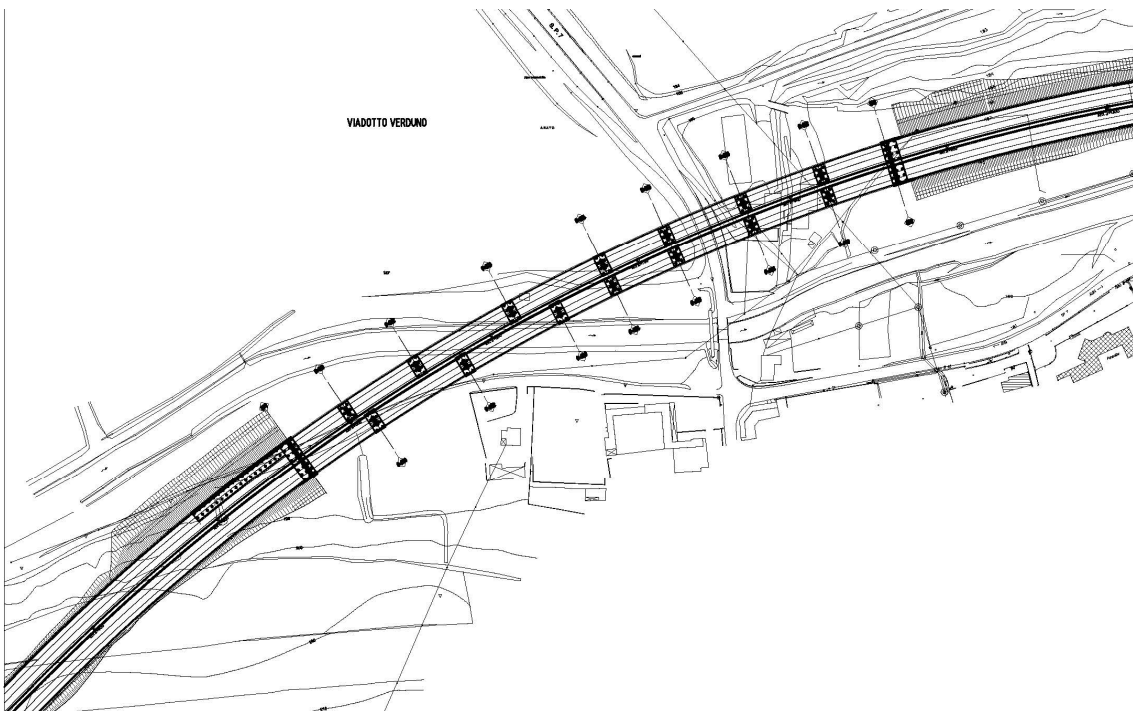
Fig.9. Viadotto Verduno nel PD
