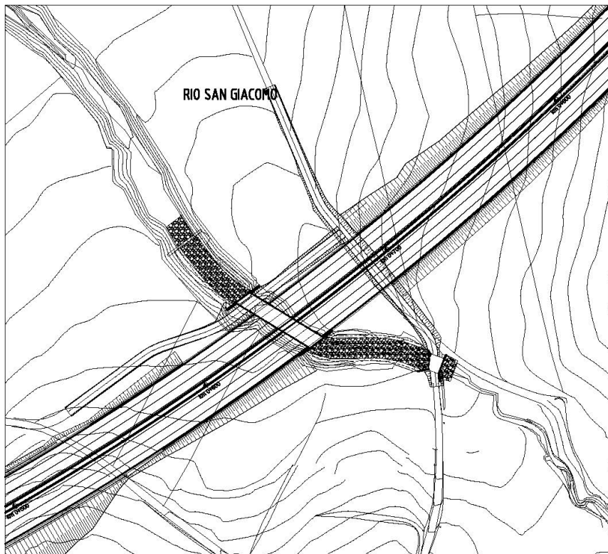
Fig.7. Attraversamento del Rio San Giacomo nel PD
