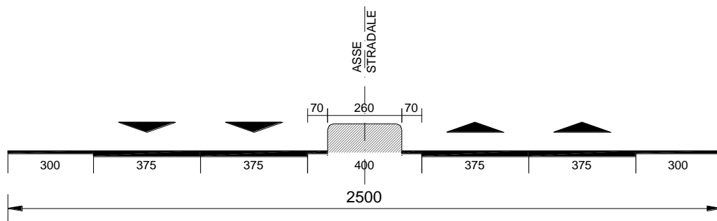
Figura 8-8 Sezione trasversale schematica
