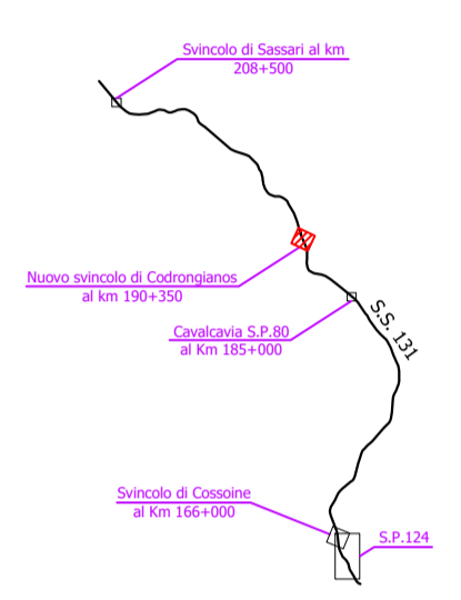
KEY MAP
