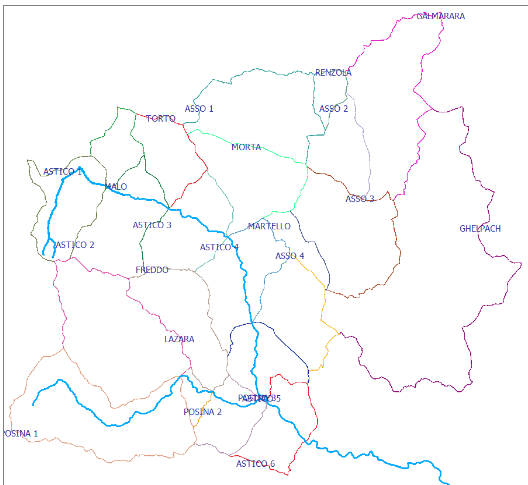
Figura 4: Rappresentazione della suddivisione in 22 sottobacini del bacino del fiume Astico con evidenziati i corsi d'acqua dell'Astico e del Posina.
