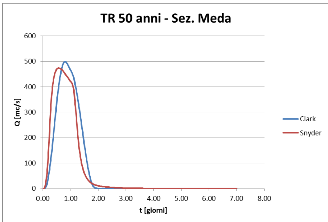
Figura 12: portata alla sezione di chiusura per un TR di 50 anni
