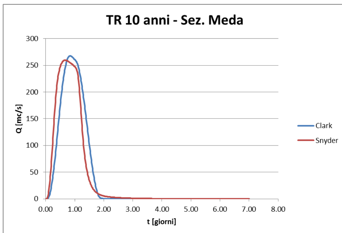
Figura 10: portata alla sezione di chiusura per un TR di 10 anni
