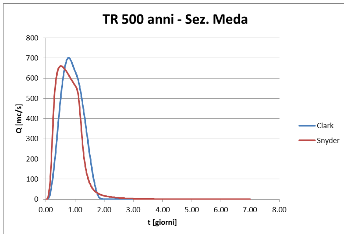
Figura 15: portata alla sezione di chiusura per un TR di 500 anni
