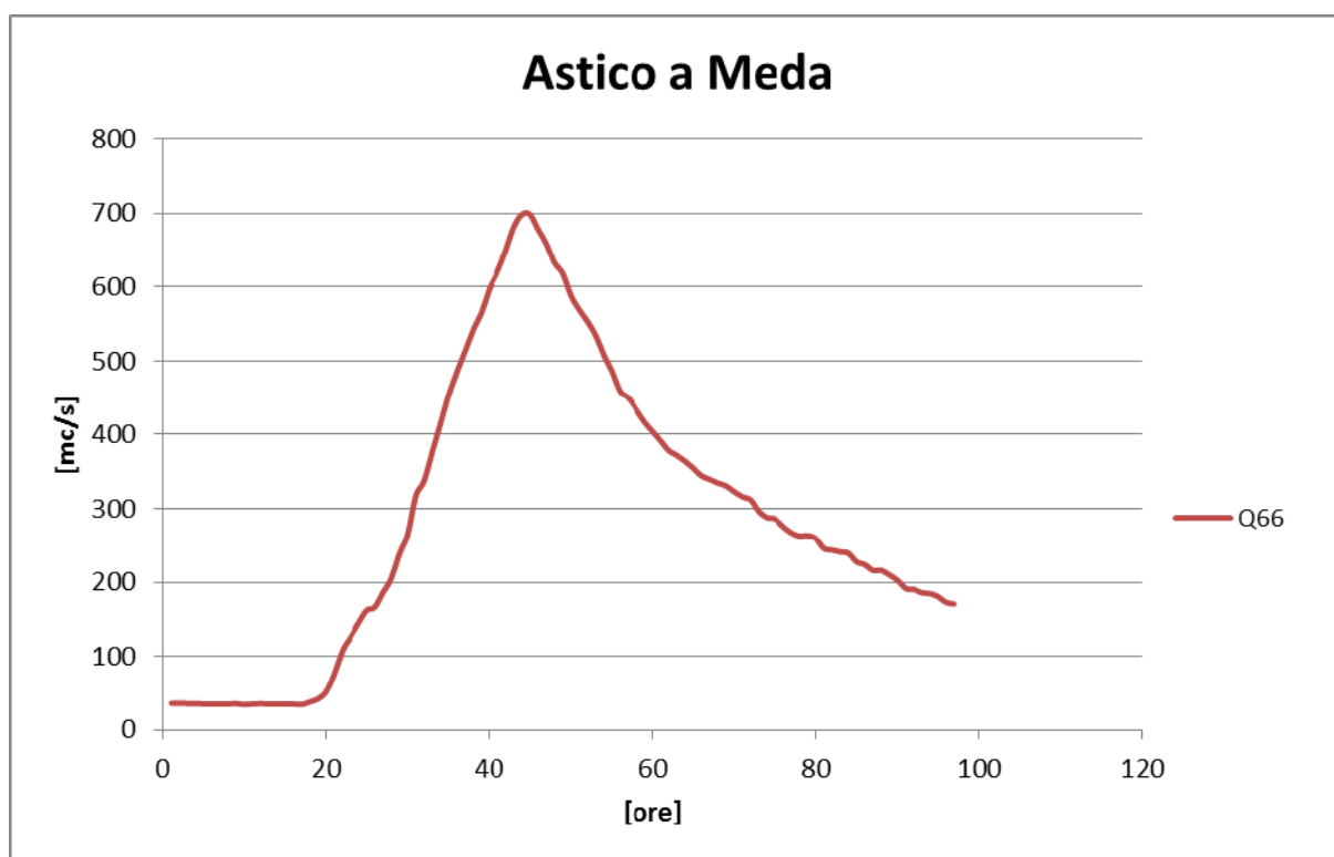
Figura 9: idrogramma dell'evento del 1966 fornito dall'Autorità di Bacino
