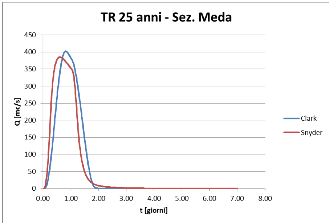
Figura 11: portata alla sezione di chiusura per un TR di 25 anni
