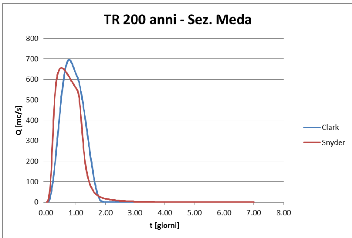
Figura 14: portata alla sezione di chiusura per un TR di 200 anni
