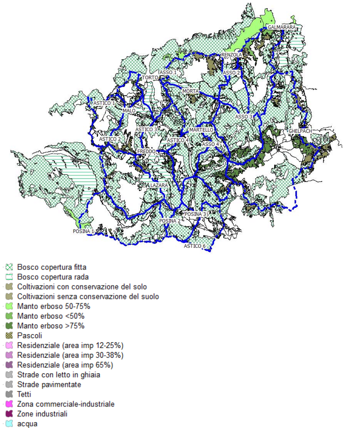
Figura 5: carta di utilizzo del suolo all'interno del bacino imbrifero dell'Astico
