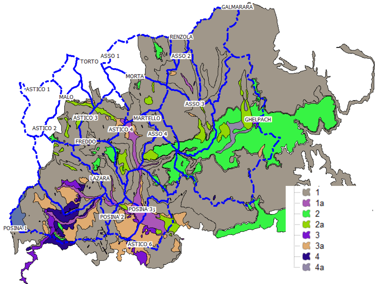
Figura 6: carta della permeabilità del suolo nel bacino imbrifero dell'Astico, dove: 1 rocce molto permeabili con fessurazione e carsismo; 2 rocce mediamente permeabili per fessurazione; 3 rocce poco permeabili per fessurazione; 4 rocce praticamente impermeabili; 1a depositi molto permeabili per porosità; 2a depositi mediamente permeabili per porosità; 3a depositi poco permeabili per porosità; 4a depositi praticamente impermeabili.
