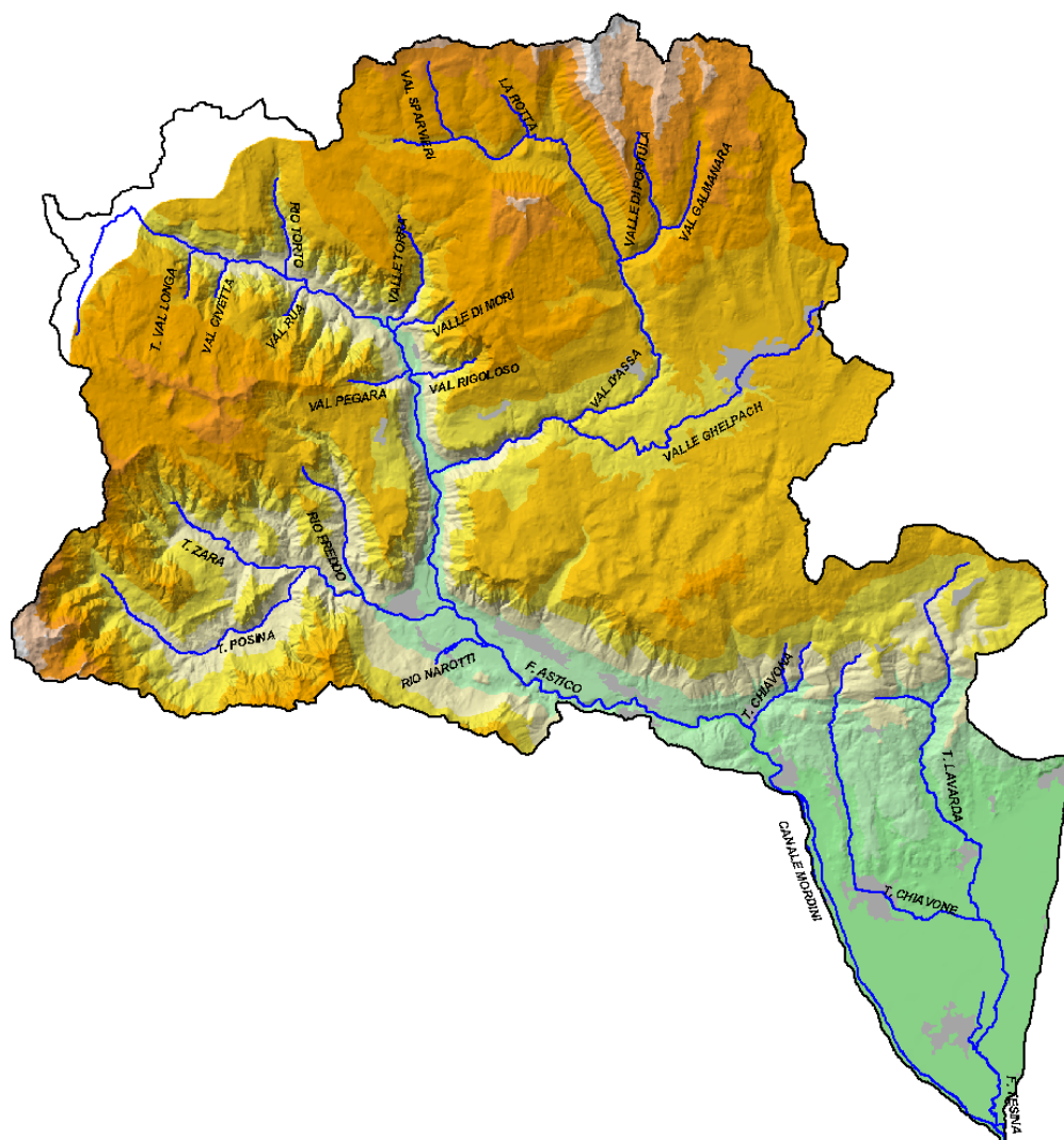
Figura 2: bacino imbrifero del torrente Astico
