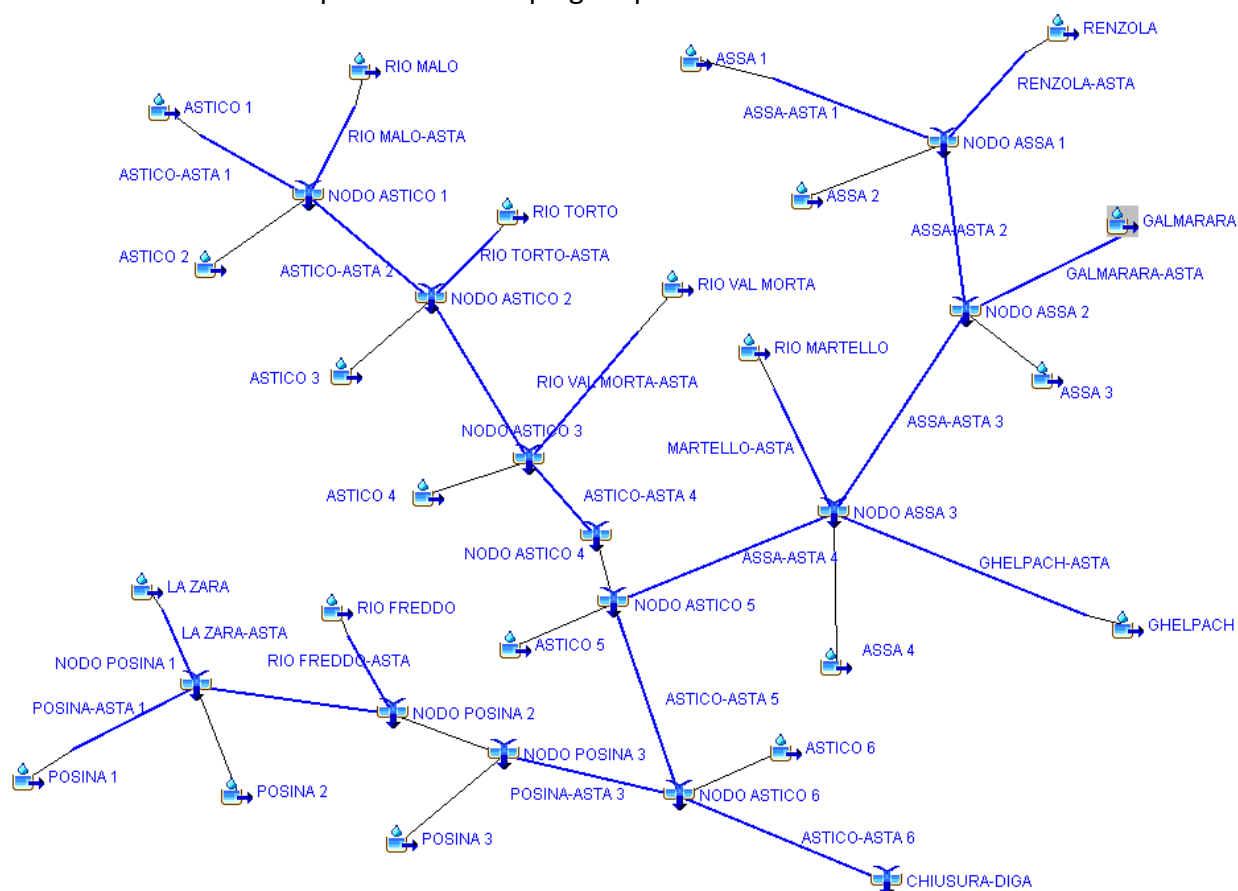
Figura 8: schema dei sottobacini costituenti il bacino imbrifero del Torrente Astico in HEC HMS
