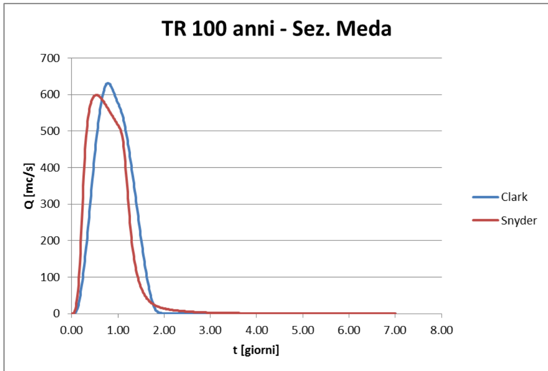
Figura 13: portata alla sezione di chiusura per un TR di 100 anni
