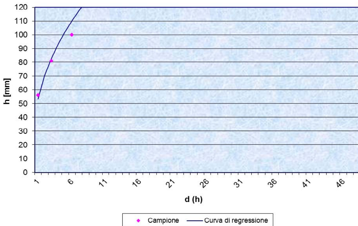
Curva di possibilità climatica -TR 25 anni
