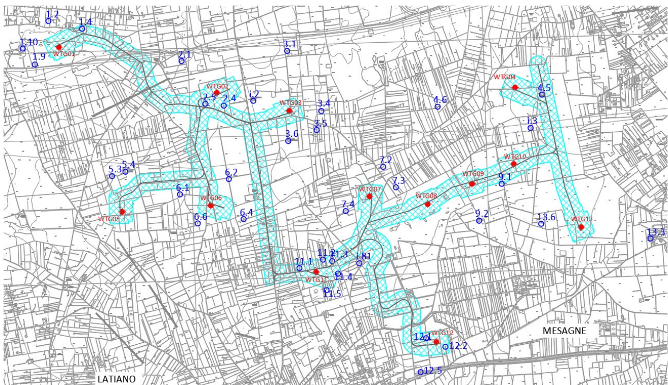
Figura1: In ciano, fascia di 100 metri dalla viabilità di impianto. In blu i ricettori ed in rosso le WTG
