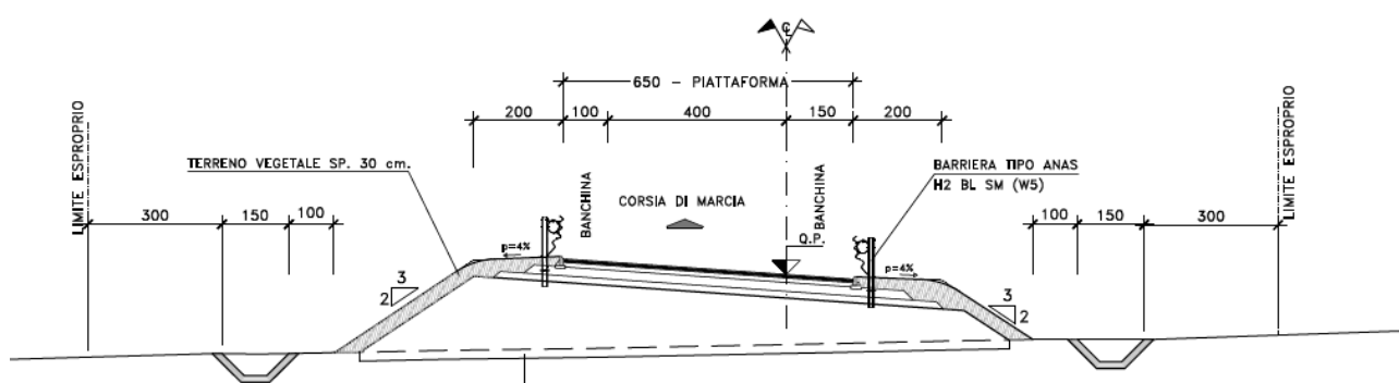
Figura 2 Sezione tipo Svincolo
