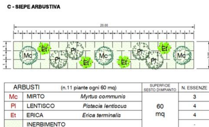
Figura 9 Sesto di impianto della tipologia C
