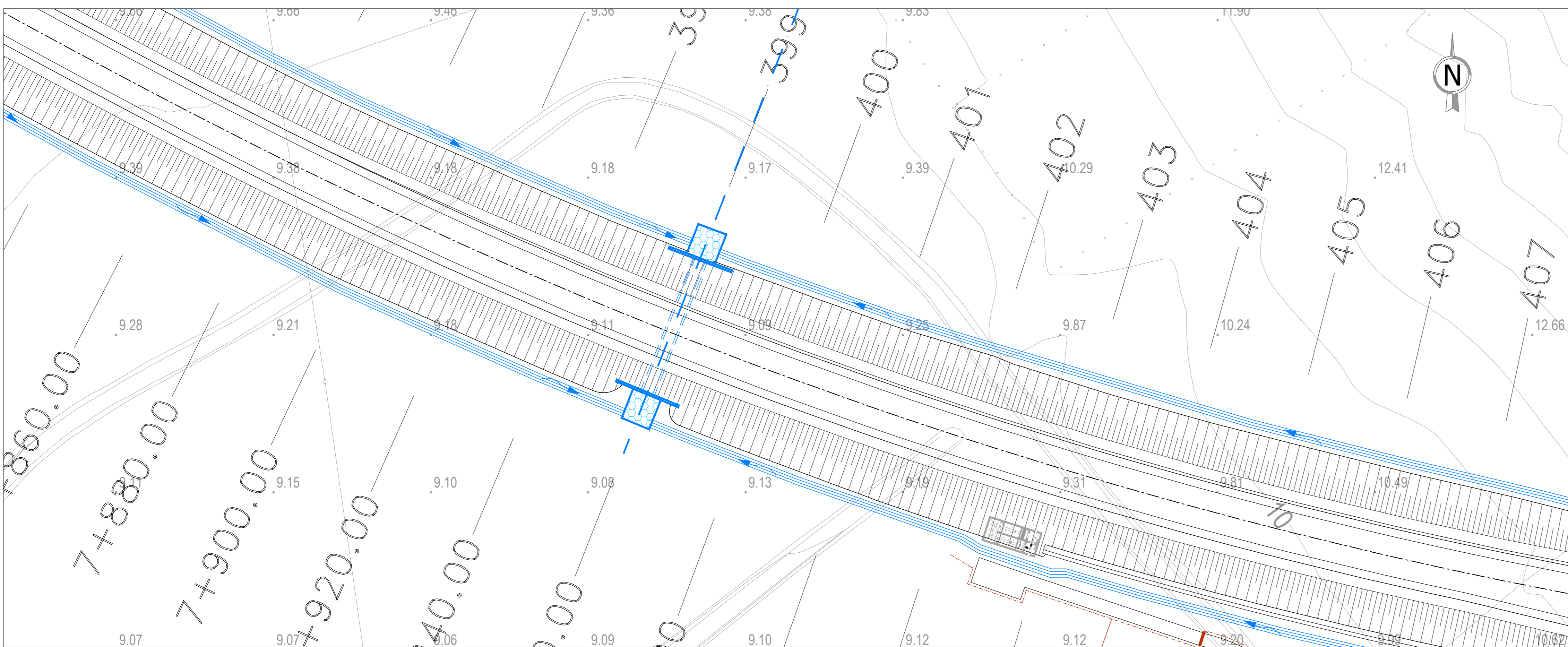
TOMBINO TM 11bis (2.00 x 2.00 m) - pk 7+960,00 - STRALCIO PLANIMETRICO
