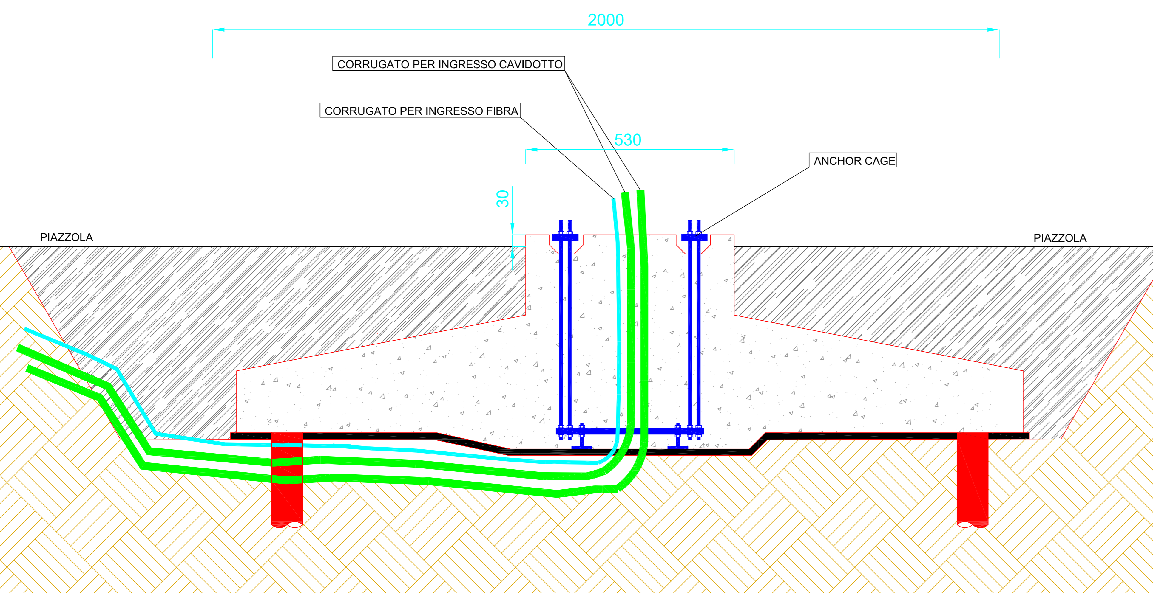
SEZIONE PLINTO DI FONDAZIONE SU PALI
