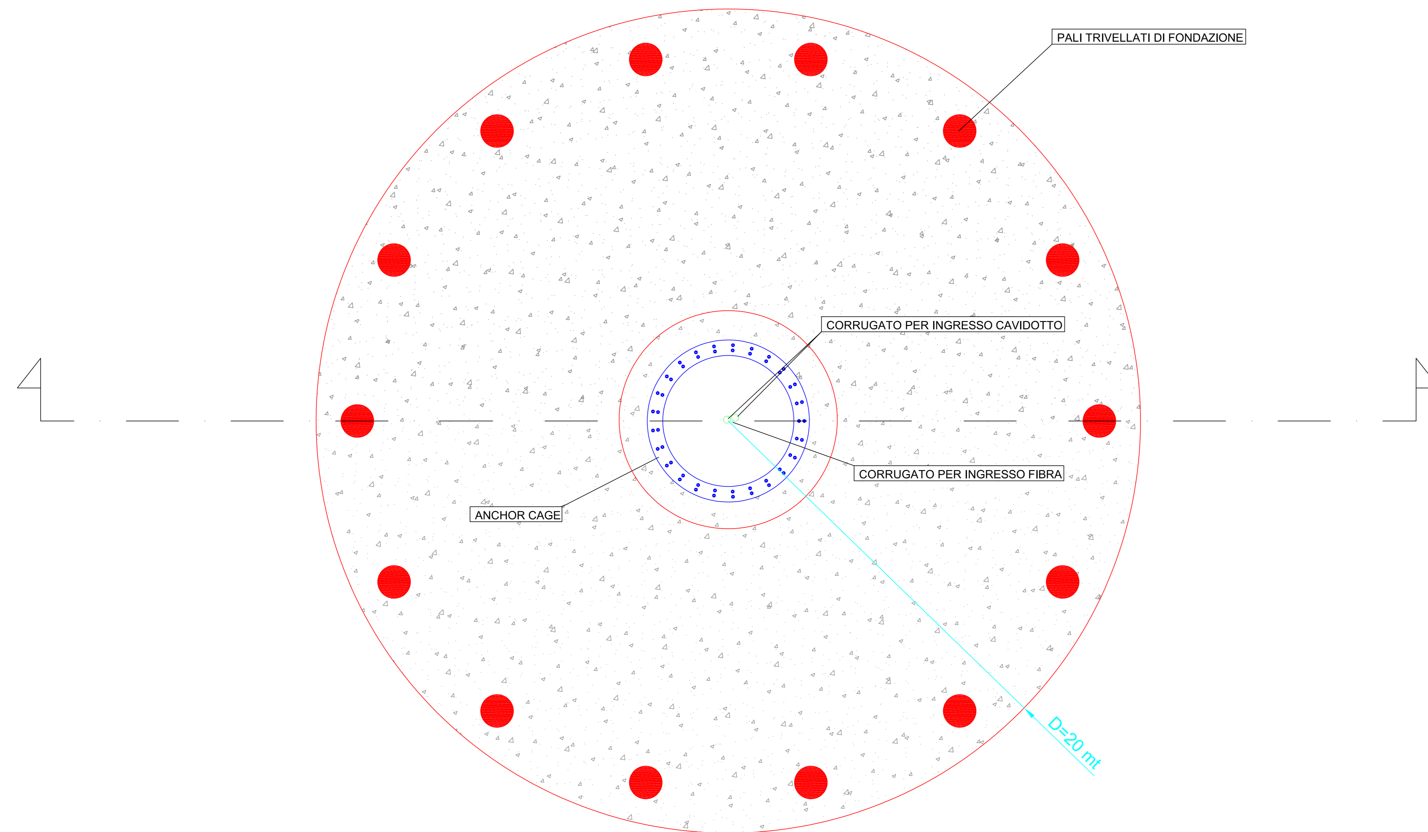
SEZIONE PLINTO DI FONDAZIONE SU PALI
