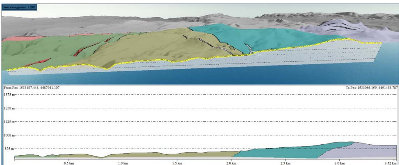
Traccia sulla carta geolitologica della sezione interpolante le posizioni delle WTG da BT05 a BT09 e BT11 e sua rappresentazione sul rilievo 3d
