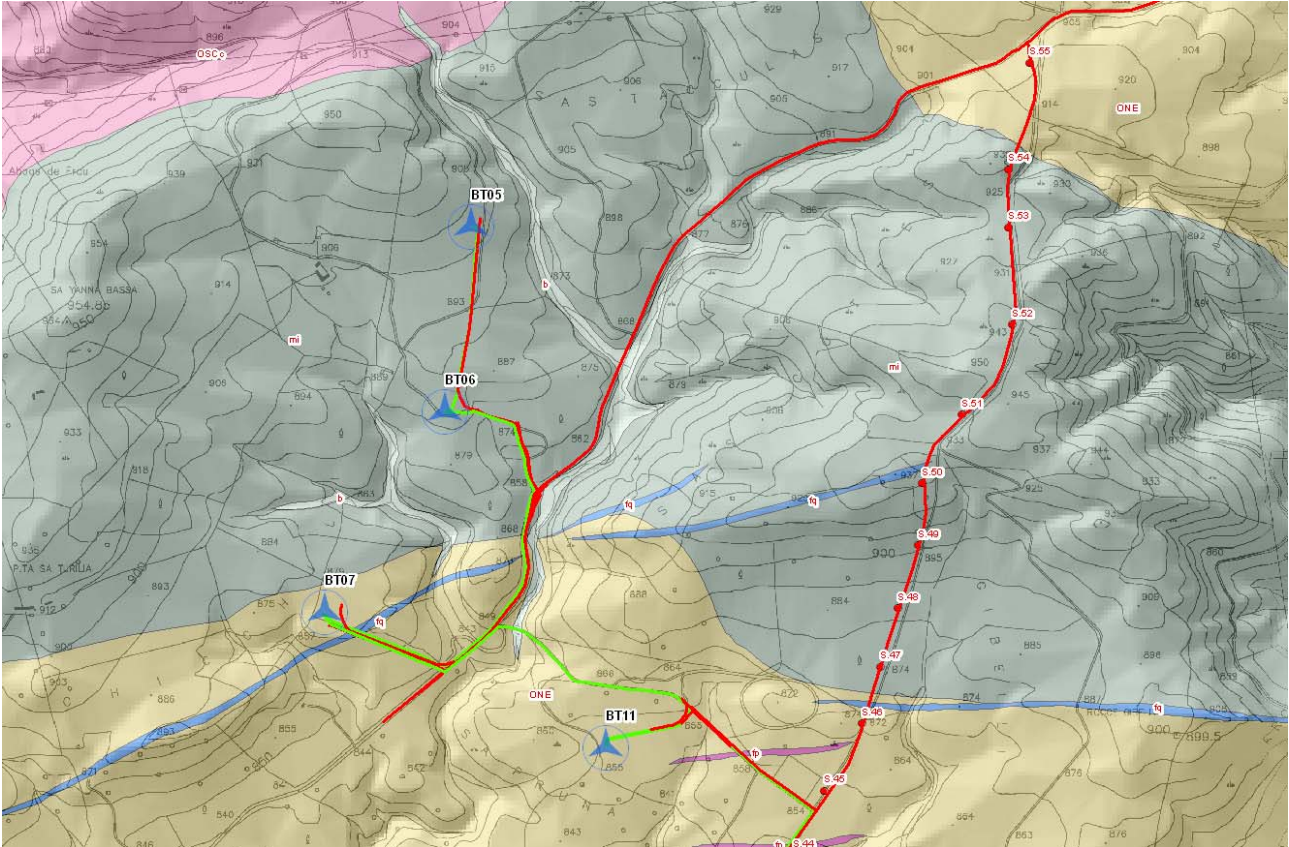
Mapa – Geolitologia, WTG e sondaggi di riferimento per i micascisti (mi)
