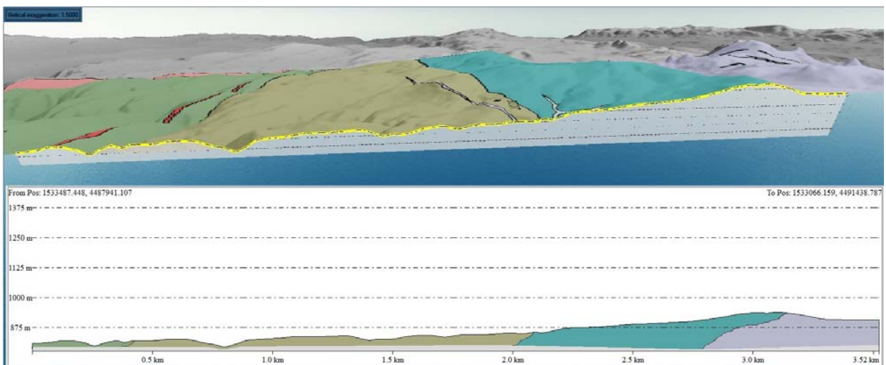
Sezione schematica dei rapporti tra le formazioni presenti nell'area degli aerogeneratori
