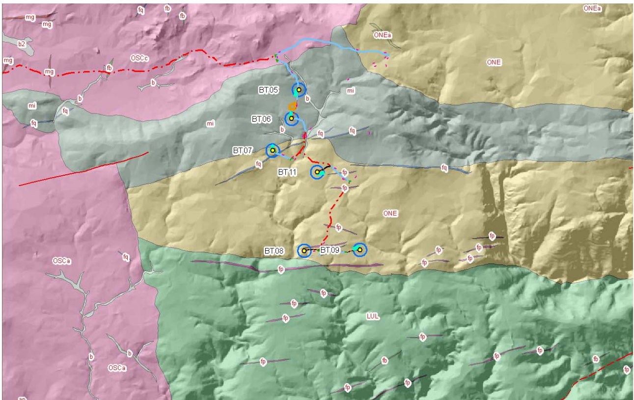
Lineazioni strutturali dell'area ristretta del Parco eolico su DTM hill shaded
