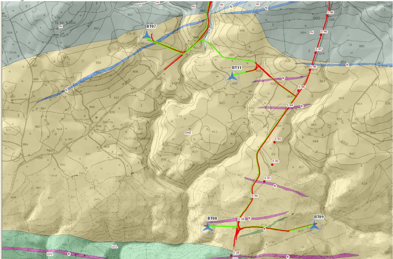
Mappa – Geolitologia, WTG e sondaggi di riferimento sugli Ortogneiss di Mamone (ONE)
