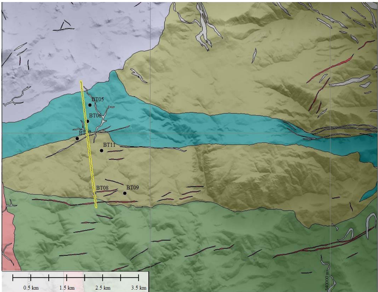
Traccia sulla carta geolitologica della sezione interpolante le posizioni delle WTG da BT05 a BT09 e BT11 e sua rappresentazione sul rilievo 3d
