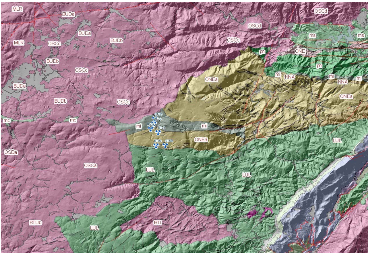
Mappa - La geologia dell'area con le quattro formazioni principali che interessano il sedime di progetto dei 6 aerogeneratori
