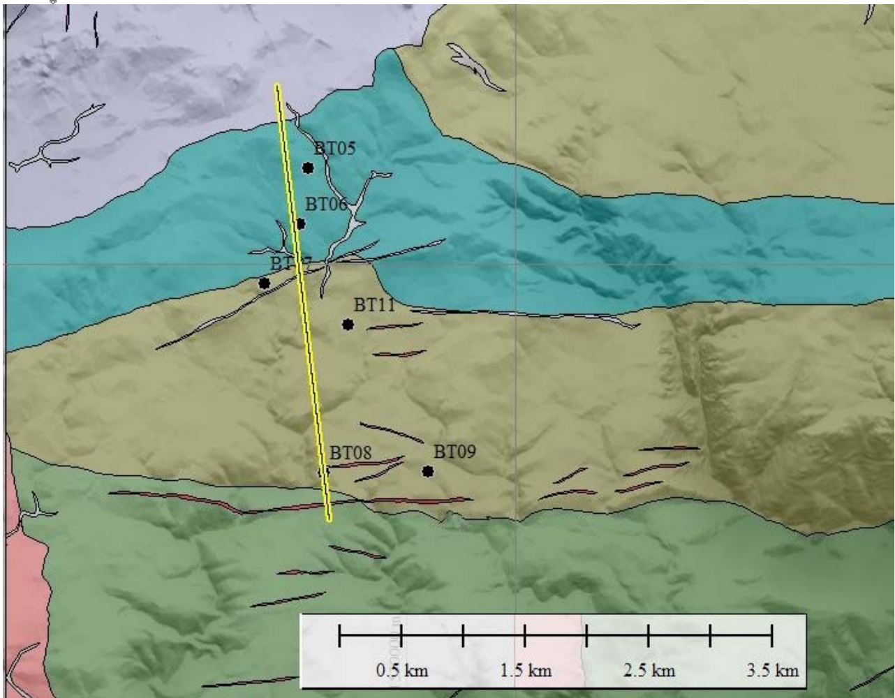
Traccia del profilo su cartografia geologica
