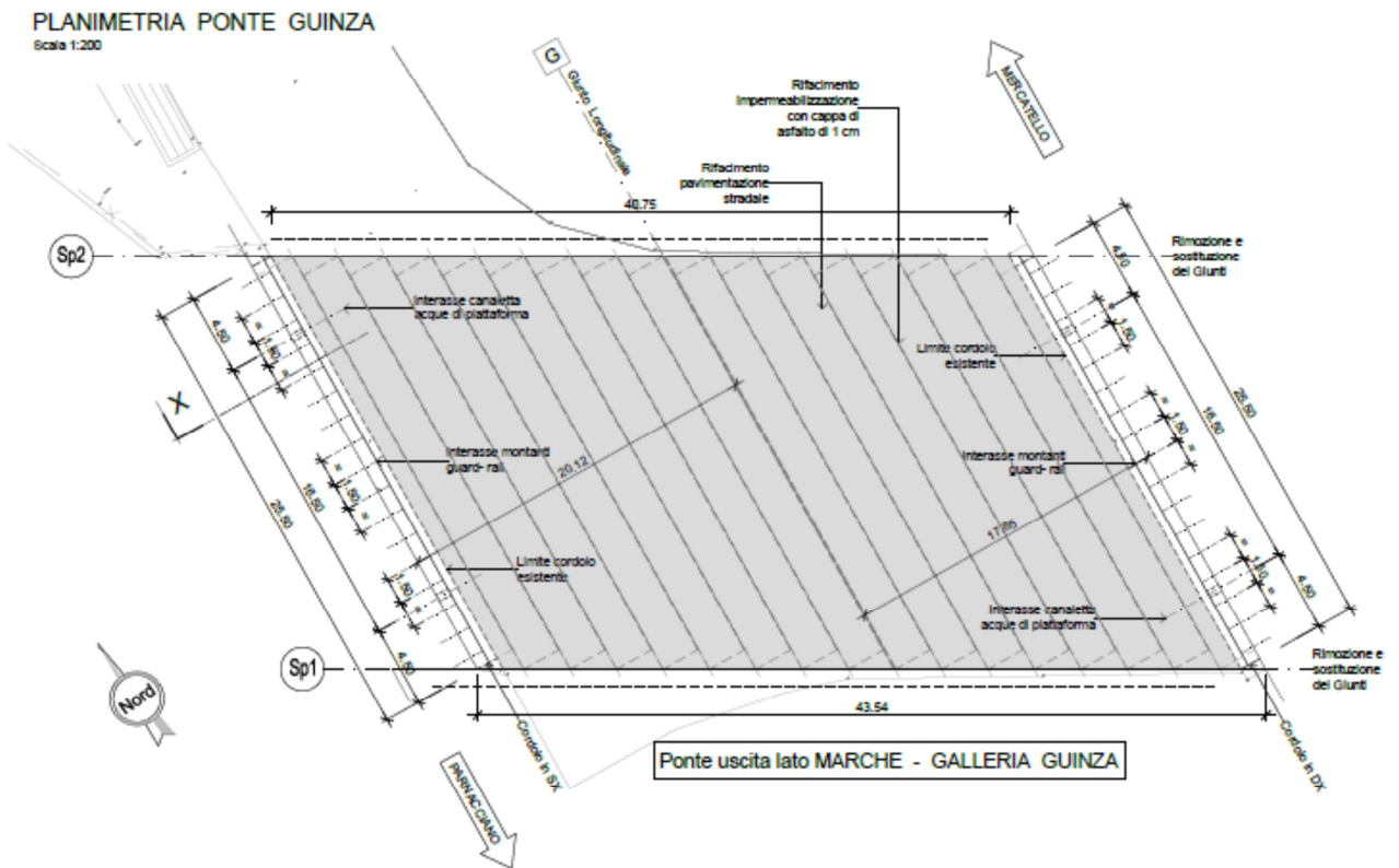
Figura 26 - planimetria del ponte
