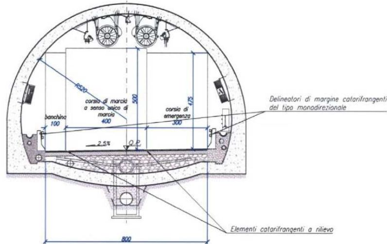
Figura 1 - sezione tipo in galleria in configurazione a senso unico direzione Umbria
