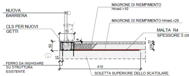
Figura 33 - intervento di sistemazione del sottovia
