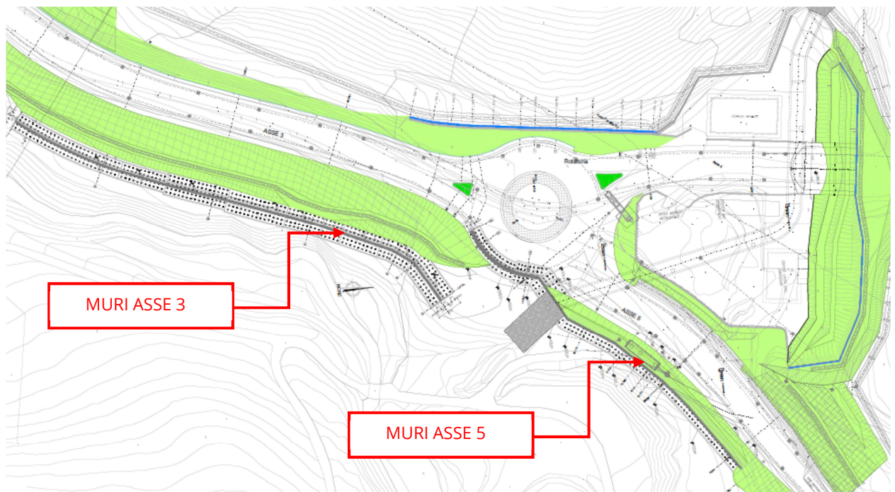
Figura 7 – Stralcio planimetrico muri Asse 3 e Asse 5.
