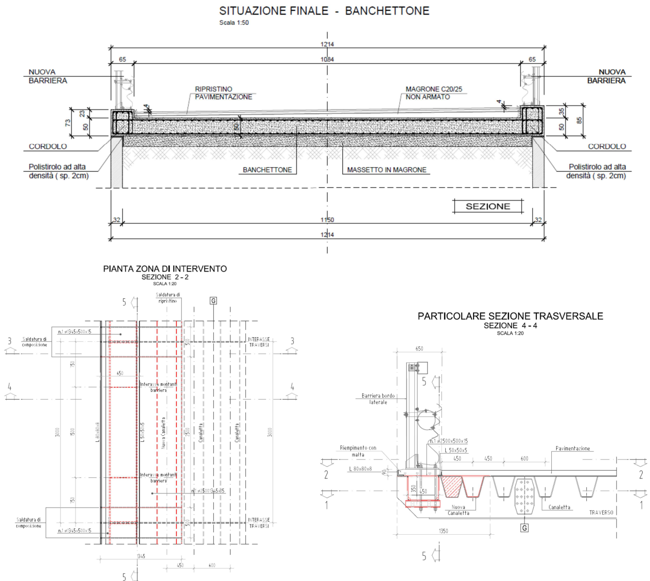
Figura 28 - interventi di sistemazione del cordolo
