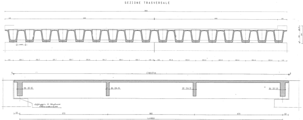
Figura 25 - sezioni longitudinale e trasversale del ponte
