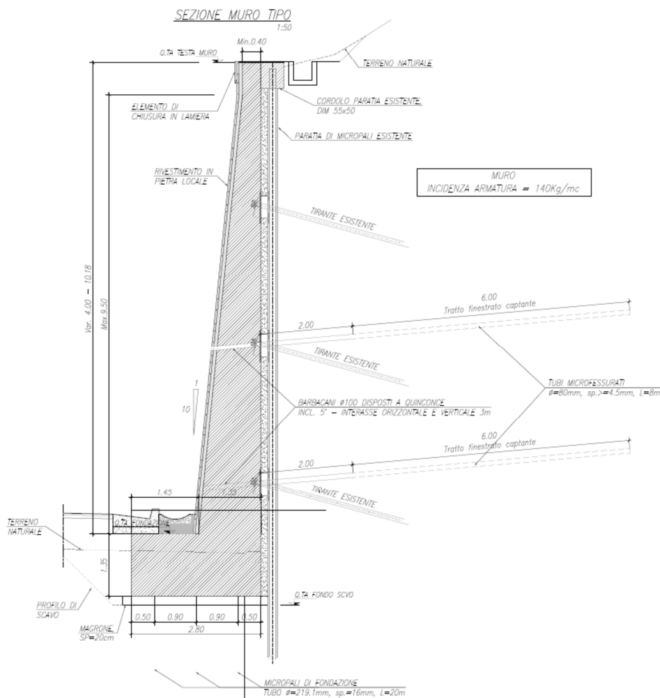
Figura 10 - Muro di consolidamento della berlinese esistente: sezione tipologica.
