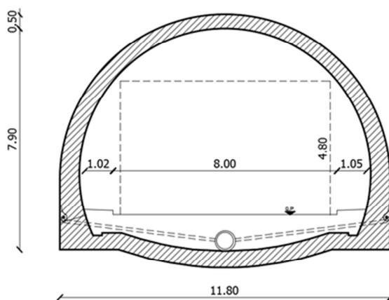
Galleria Guinza - Stato attuale
