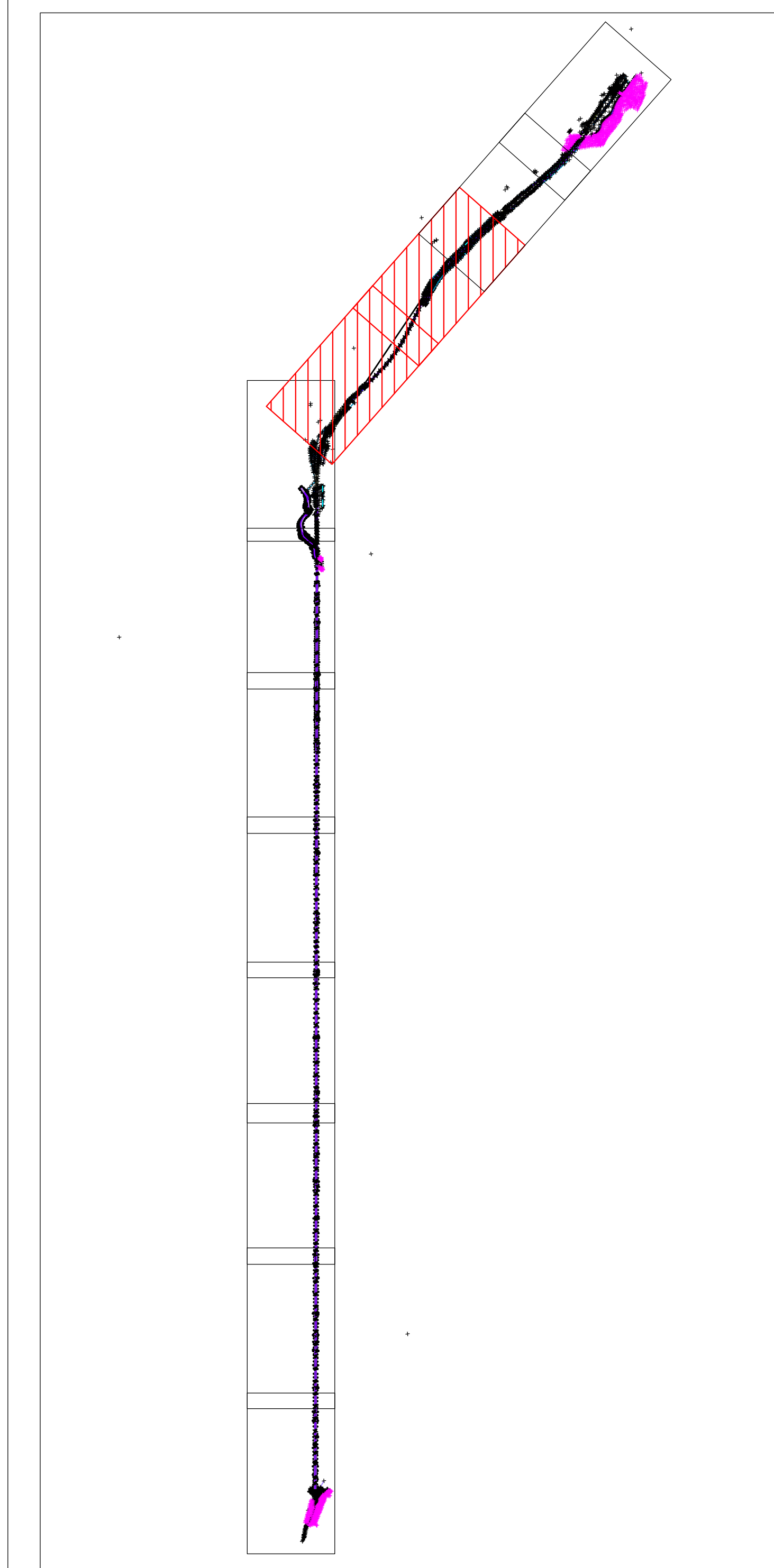
PLANIMETRIA DEI RILIEVI COMPLESSIVA scala 1:1.000
