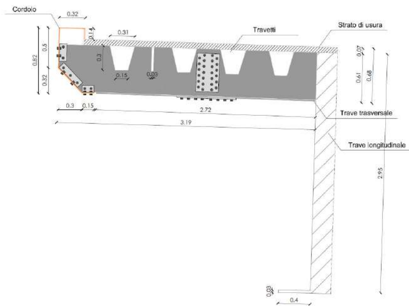
Figura 9 – Planimetria soletta a sbalzo del viadotto.
