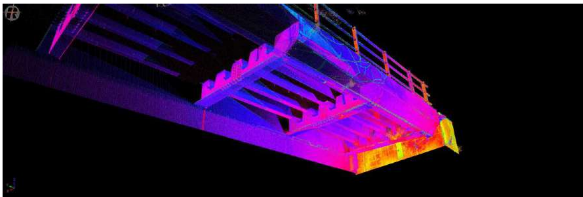
Figura 3 – Nuvola di punti tridimensionali della soletta a sbalzo del viadotto.
