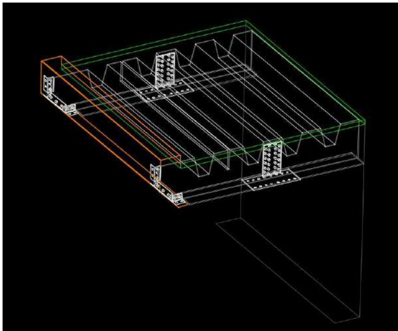
Figura 7 – Modellino 3D della soletta a sbalzo del viadotto.
