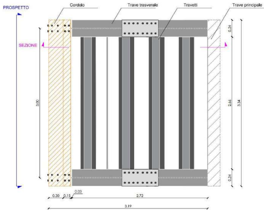
Figura 8 – Planimetria soletta a sbalzo del viadotto.
