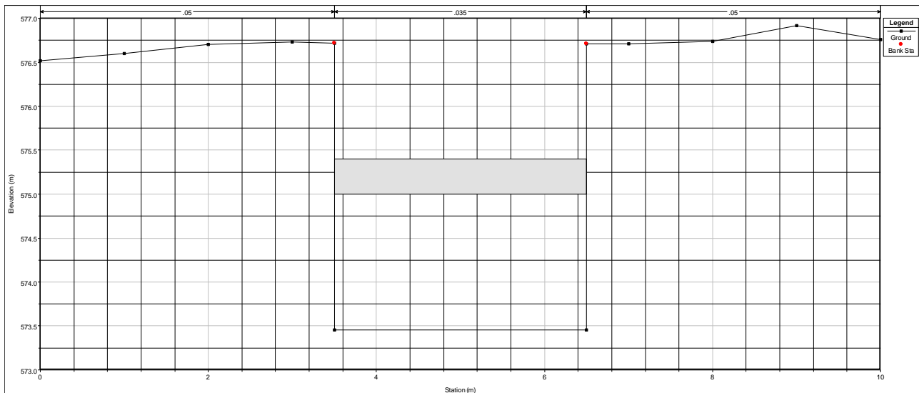
Figura 12 - Sezione tipo Tombino 3x2m
