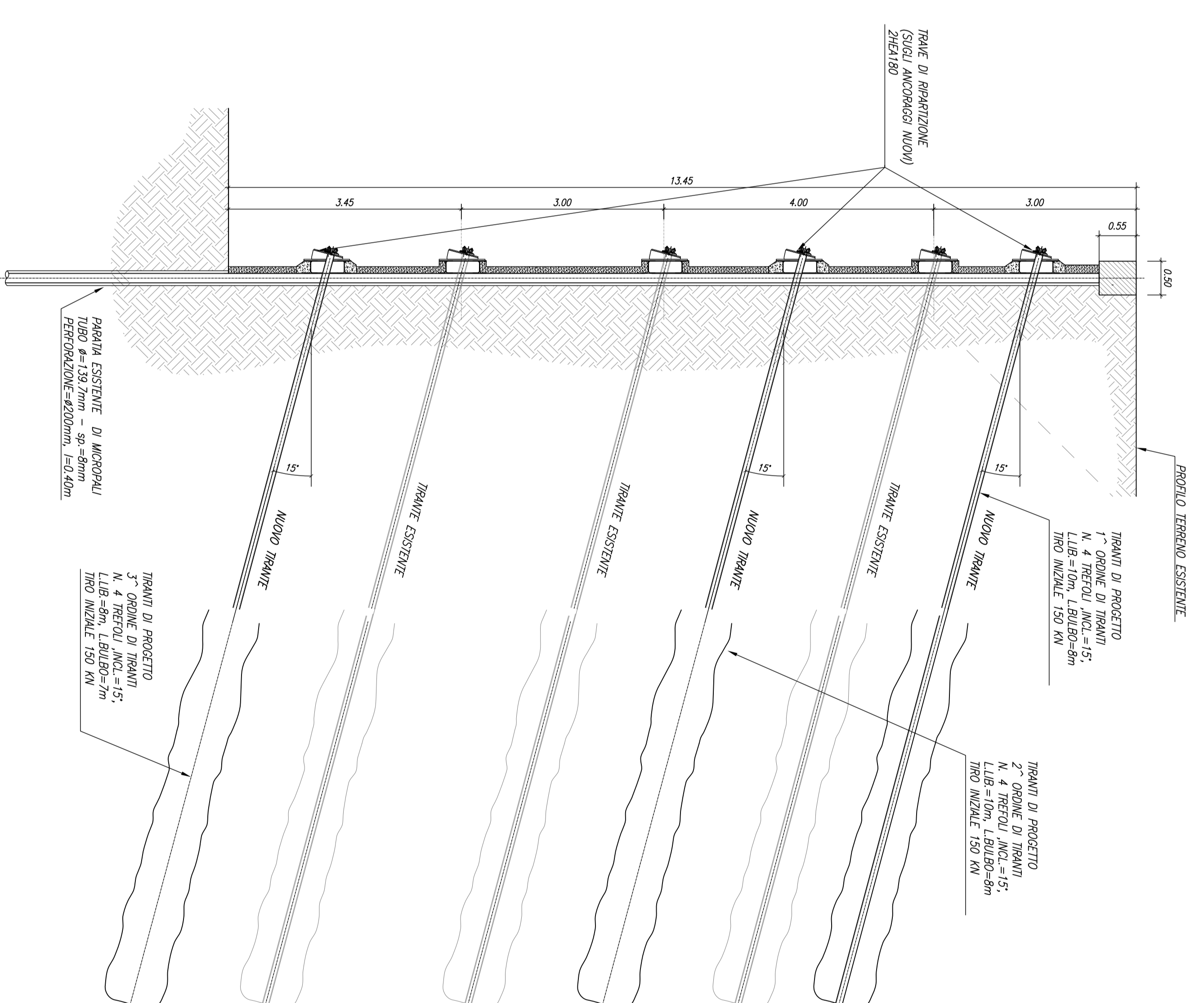
SEZIONE TIPO A-A 1:50
