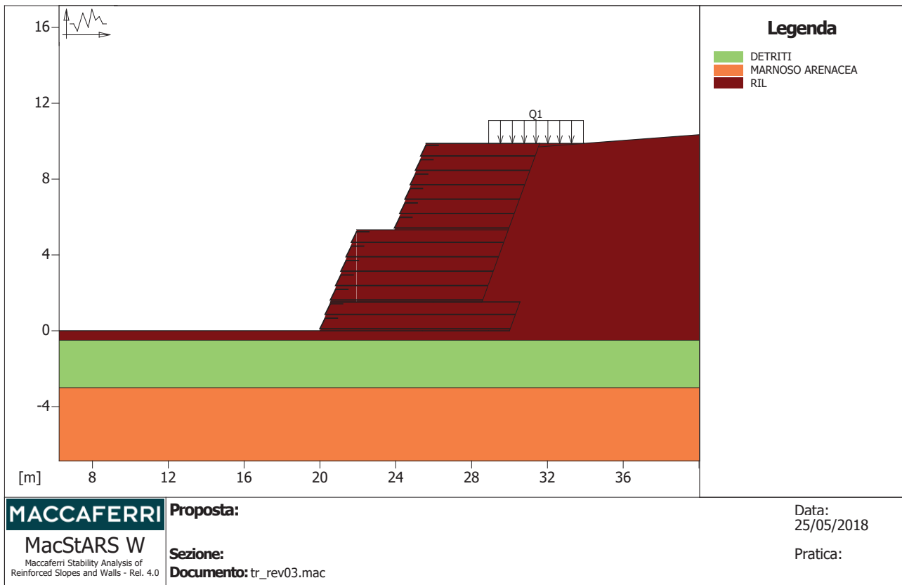
Figura 4.5 – Stratigrafia di progetto.
