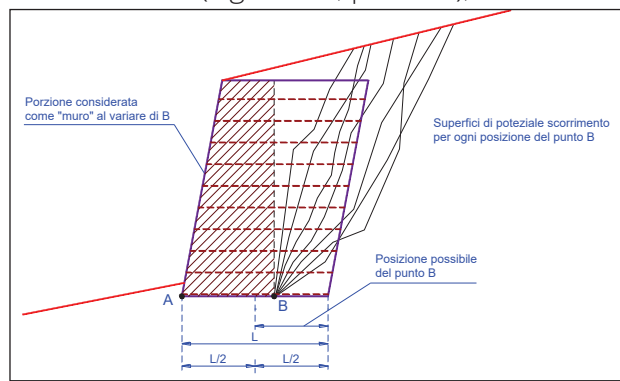
Figura 4.3 – Macstars: verifiche a scorrimento.
