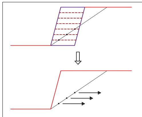
Figura 4.1 – Macstars: implementazione dei rinforzi.
