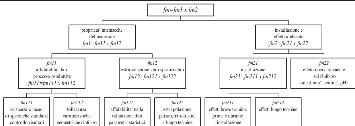
Figura 4.6 – Definizione del fattore di sicurezza per il calcolo della resistenza di lavoro.
