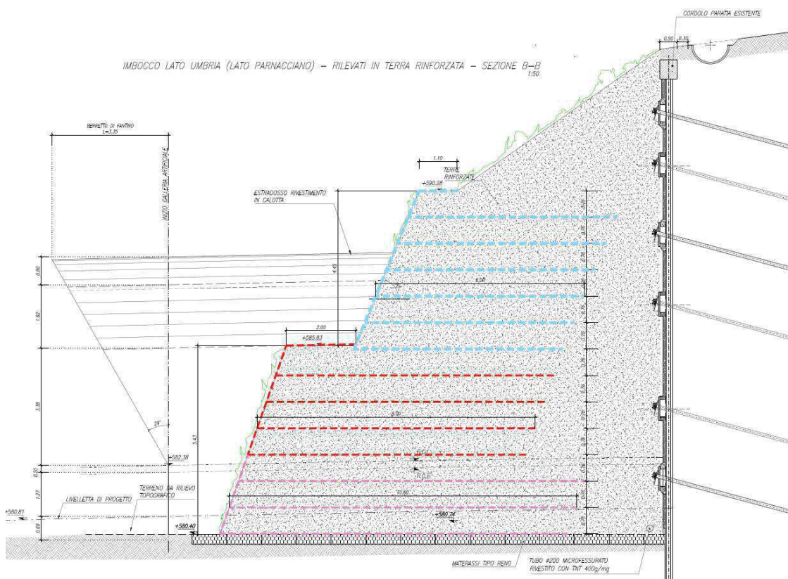
Figura 3.3 - Sezione tipologica B-B.
