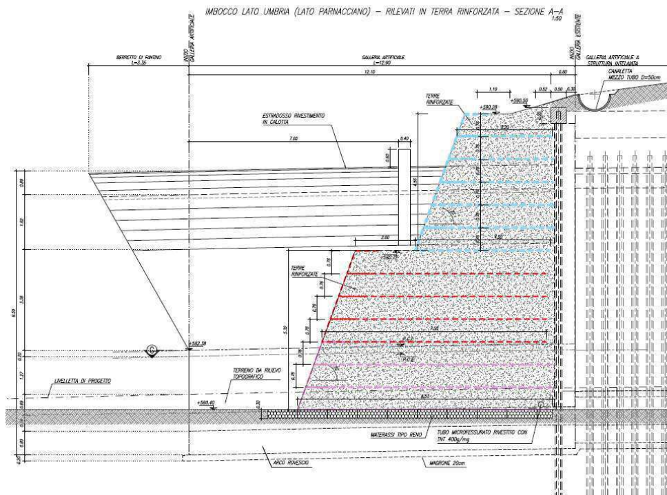
Figura 3.2 – Sezione tipologica A-A.
