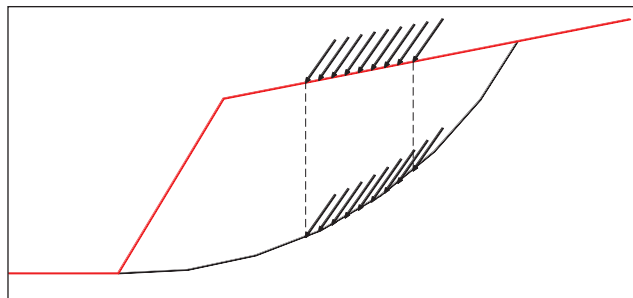
Figura 4.2 – Macstars: implementazione dei carichi superficiali.
