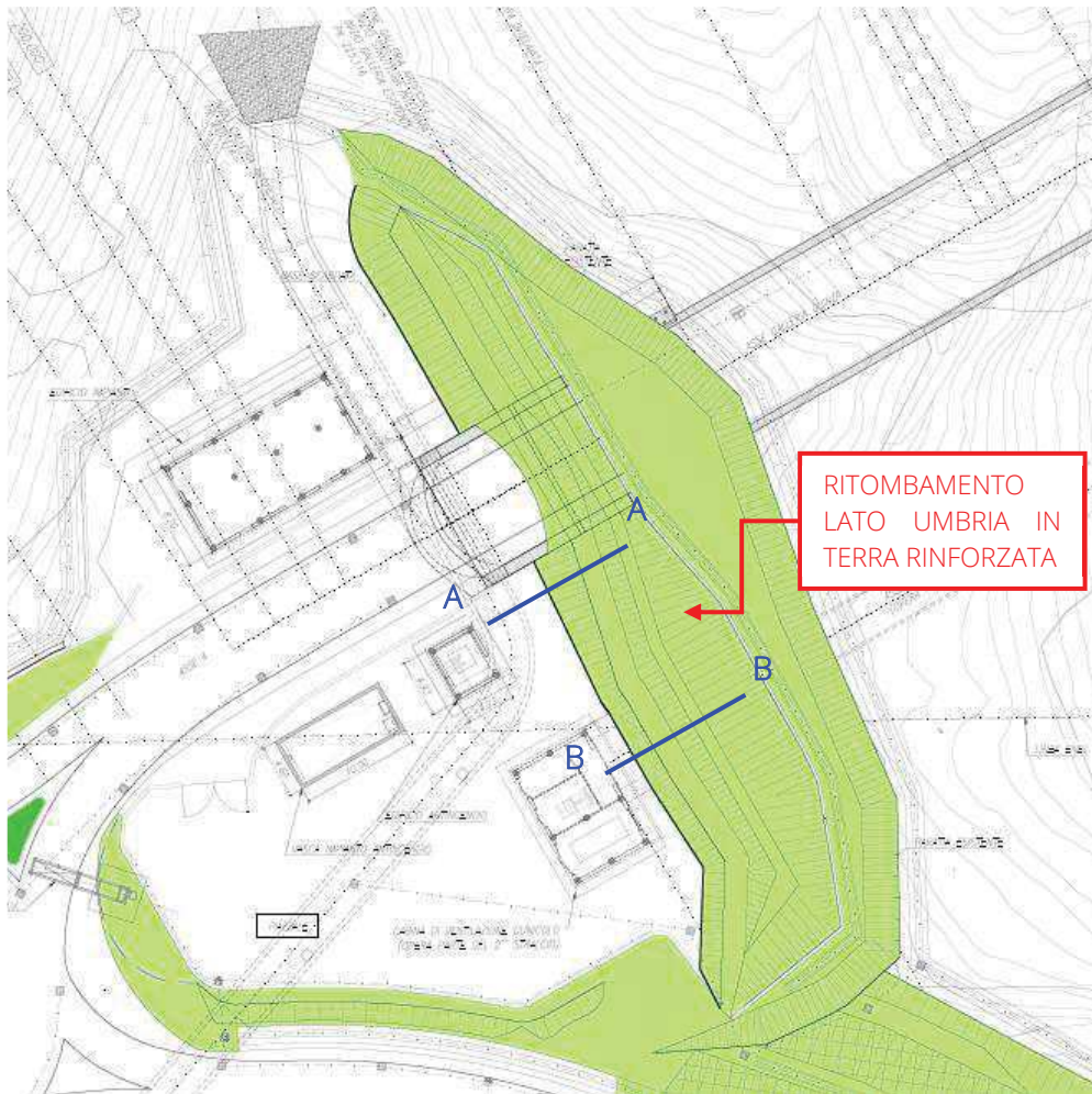
Figura 3.1 - Stralcio planimetrico dell'intervento.
