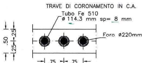
Figura 7.2 - Disegni contabili: particolari paratia esistente in prossimità della rotatoria.
