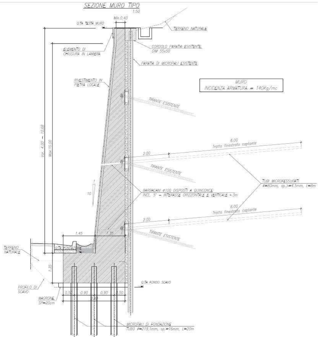
Figura 4.2 - Muro di consolidamento della berlinese esistente: sezione tipologica.
