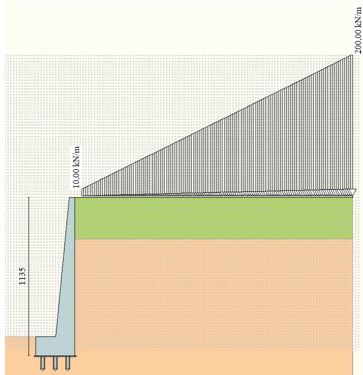
Figura 5.4 – Muro di consolidamento della berlinese provvisionale: sovraccarico che simula la scarpata.
