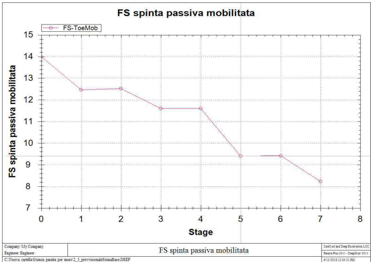
Figura 7.7 - FS spinta passiva/vera.
