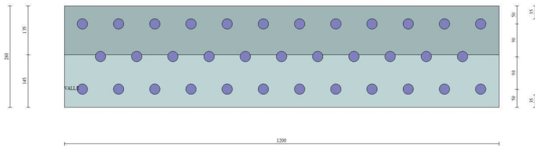
Figura 5.2 – Muro di consolidamento berlinese: disposizione dei micropali di fondazione.
