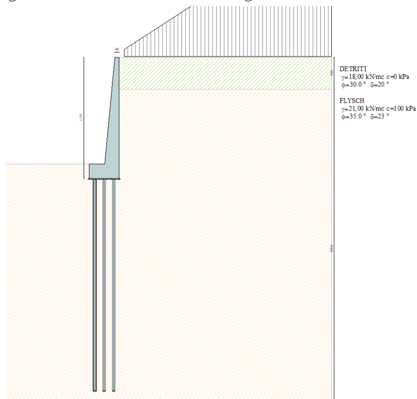
Figura 5.3 – Muro di consolidamento berlinese rotatoria: stratigrafia di progetto.
