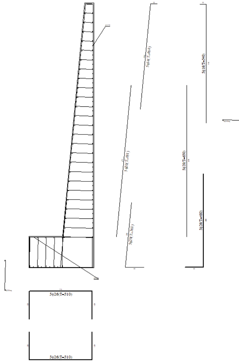
Figura 5.5 – Muro di consolidamento della berlinese esistente: distinta ferri.
