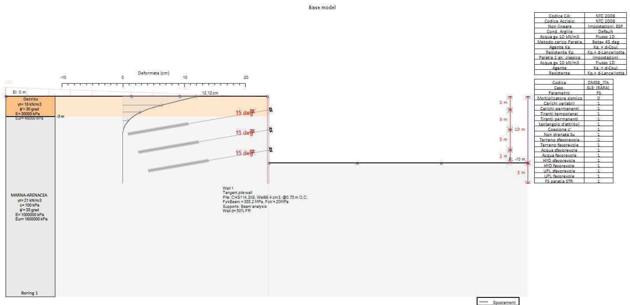
Figura 7.4 - SLE - diagramma involucro spostamenti.
