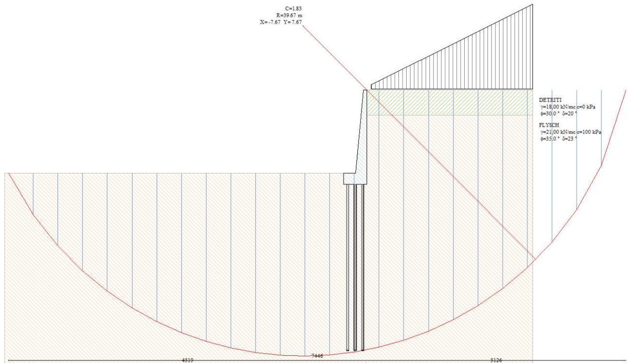
Figura 5.7 - Muro di consolidamento della berlinese esistente: verifica sismica SLV M2+R2.
