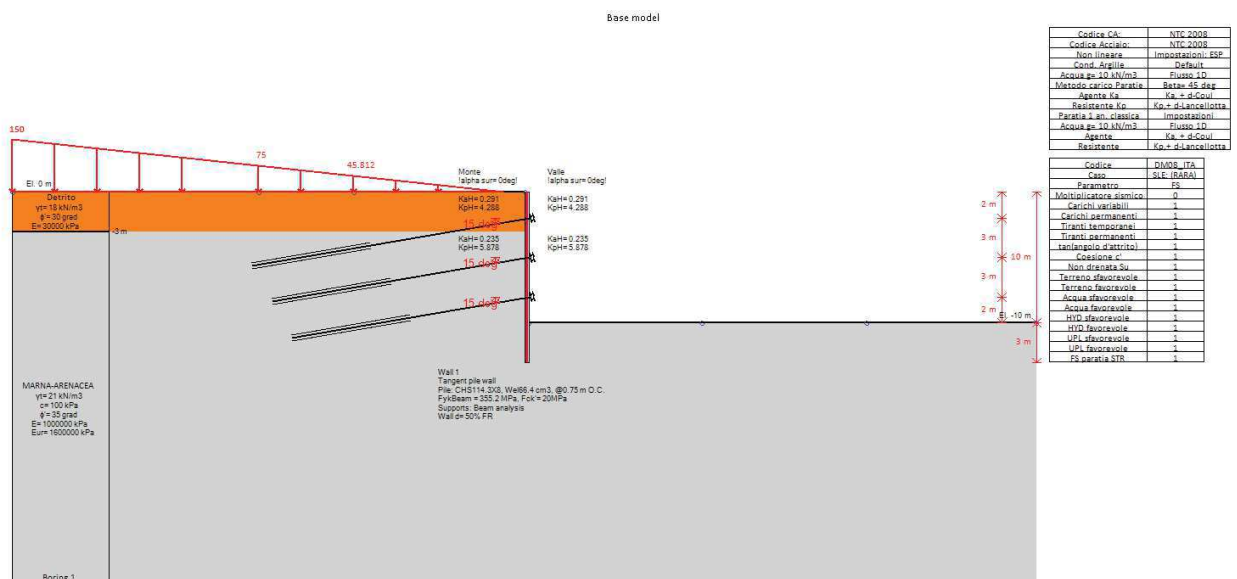
Figura 7.3 - Sezione di calcolo della paratia esistente in prossimità della rotatoria.
