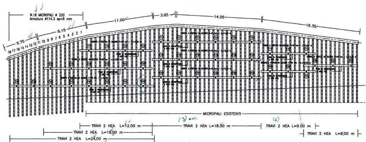
Figura 7.1 - Sviluppata paratia esistente in prossimità della rotatoria: disegni contabili
