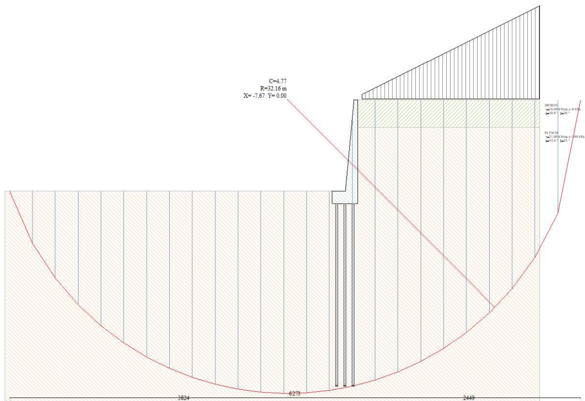
Figura 5.6 - Muri di consolidamento della berlinese esistente: verifica statica SLU A2+M2+R2.
