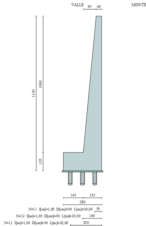
Figura 5.1 – Muro di consolidamento berlinese: geometria del muro di sostegno.
