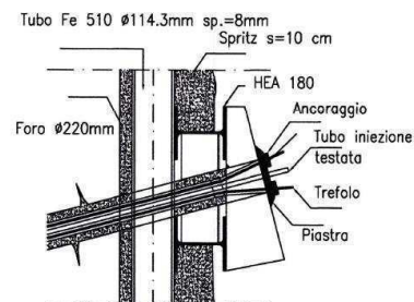
Figura 7.2 - Disegni contabili: particolari paratia esistente in prossimità della rotatoria.
