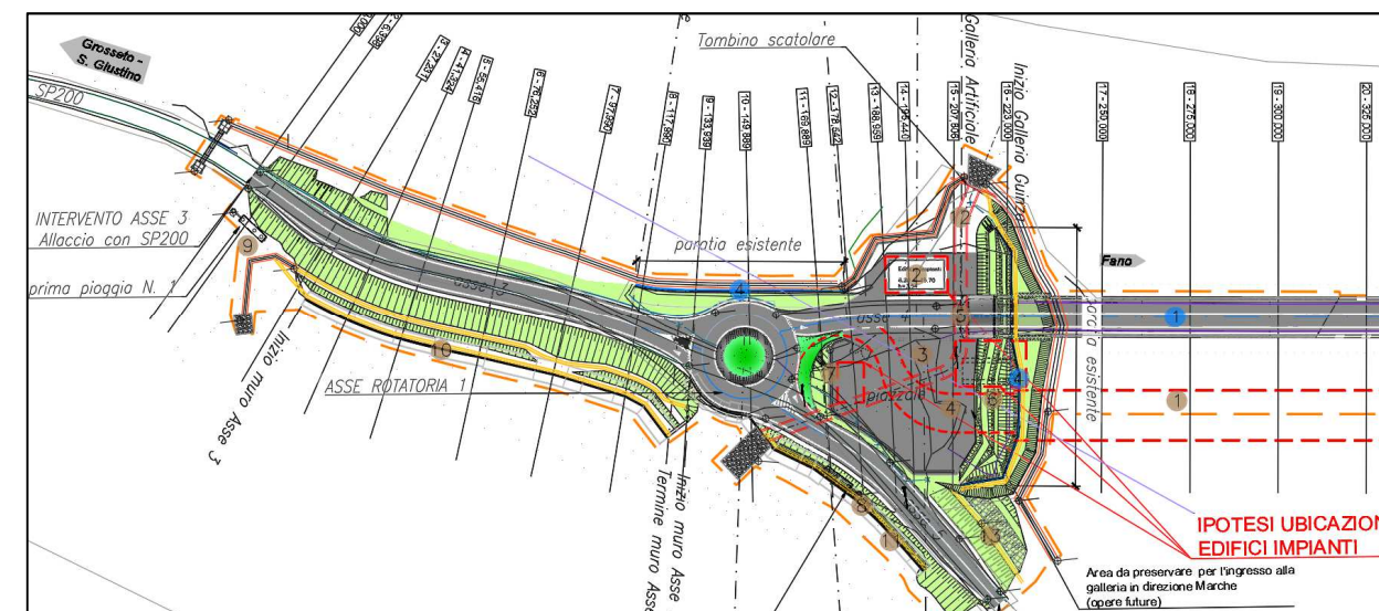
Figura 2: planimetria dell’intersezione sul lato umbro della Galleria della Guinza (Rotatoria 1)
