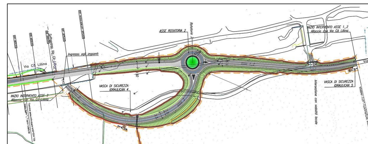
Figura 3: planimetria dell’intersezione sul lato marchigiano della galleria della Guinza (Rotatoria 2)
