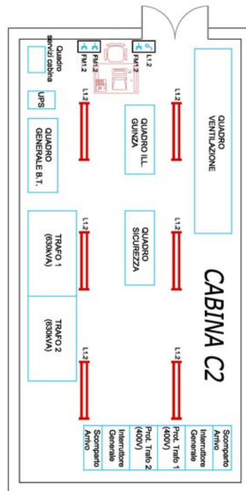
Fig.07 – lay-out cabina interna C2
