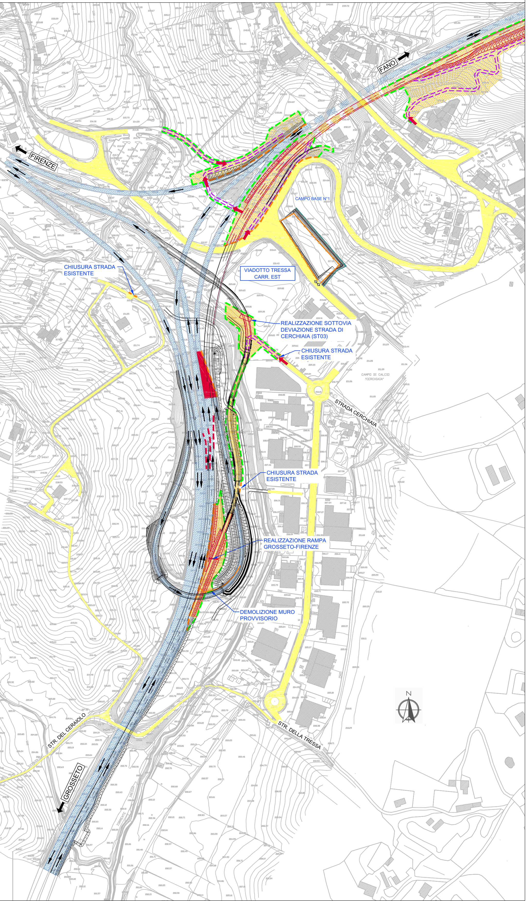
PLANIMETRIA FASE DI LAVORO 1 d
