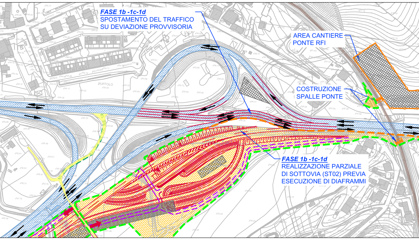
PLANIMETRIA FASE DI LAVORO 1b - 1c - 1d
