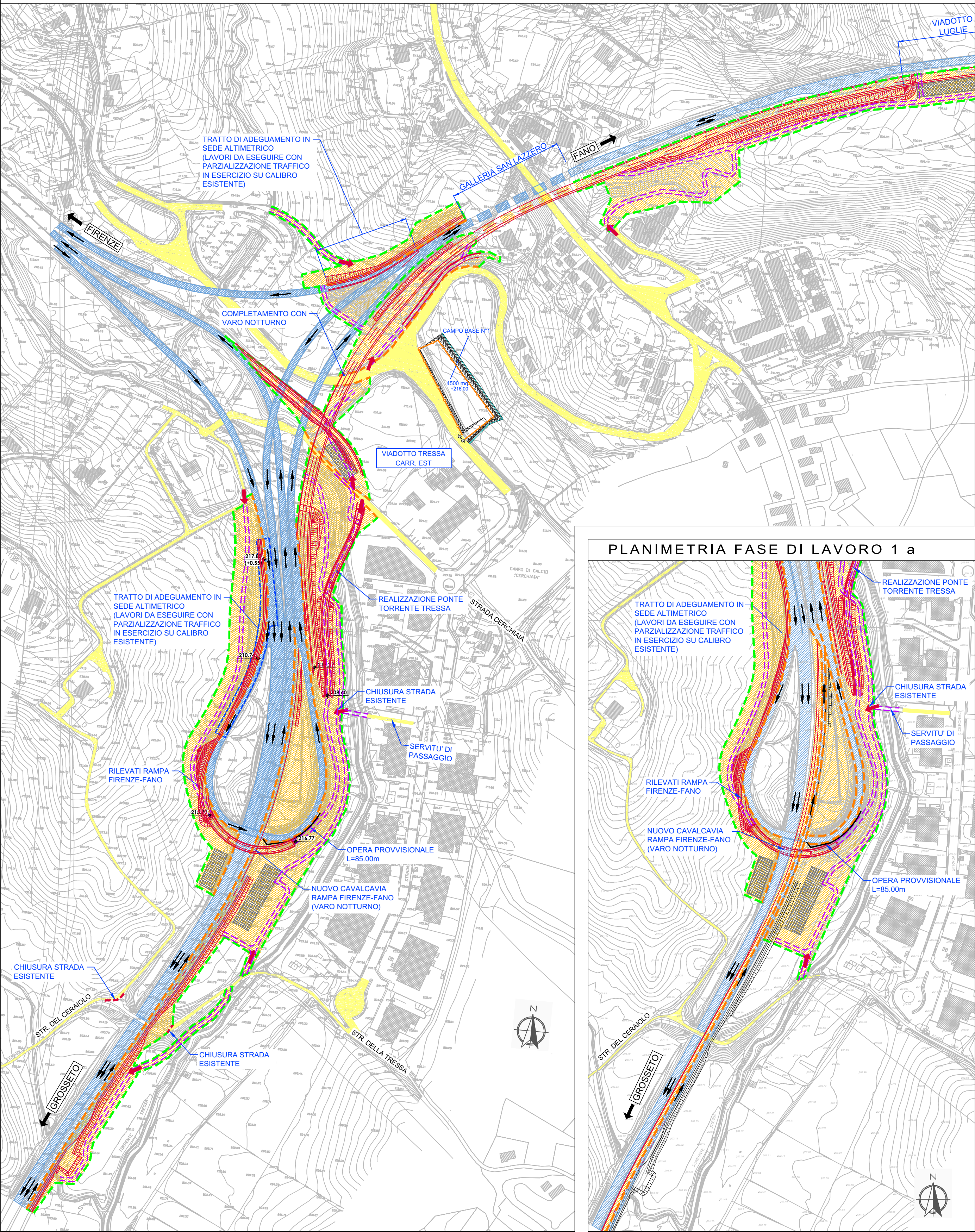
PLANIMETRIA FASE DI LAVORO 1 a
