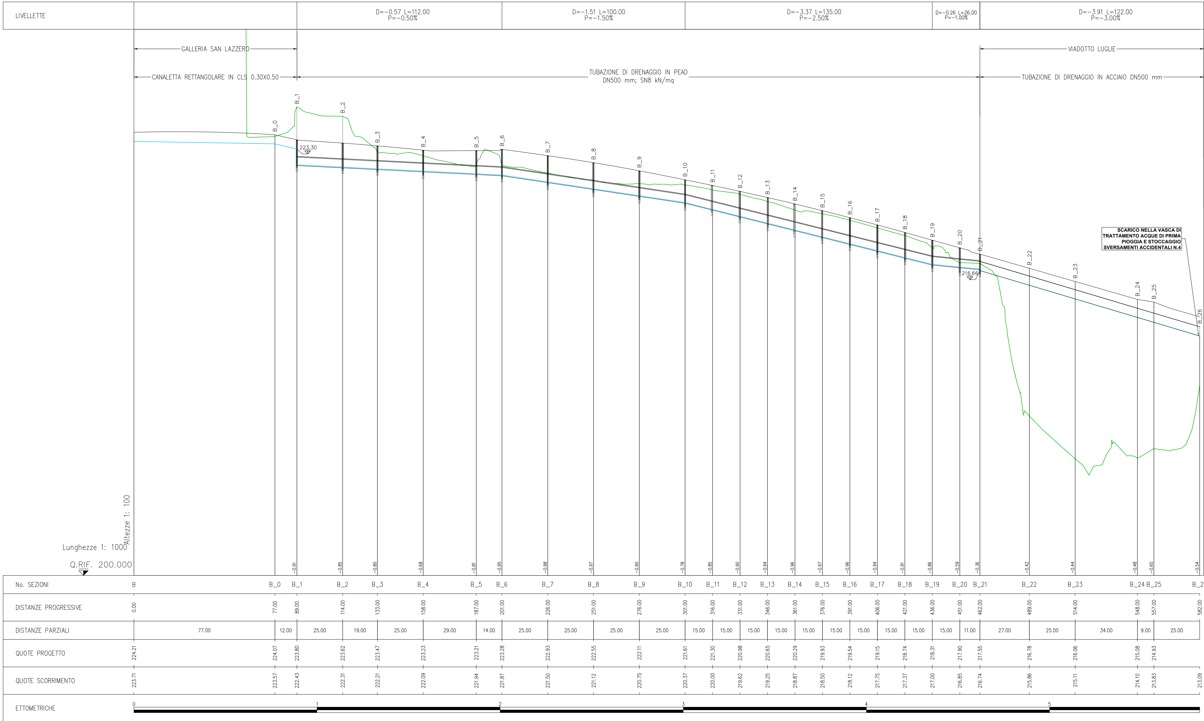
ASSE FANO-GROSSETO PROFILO LONGITUDINALE ASSE B
