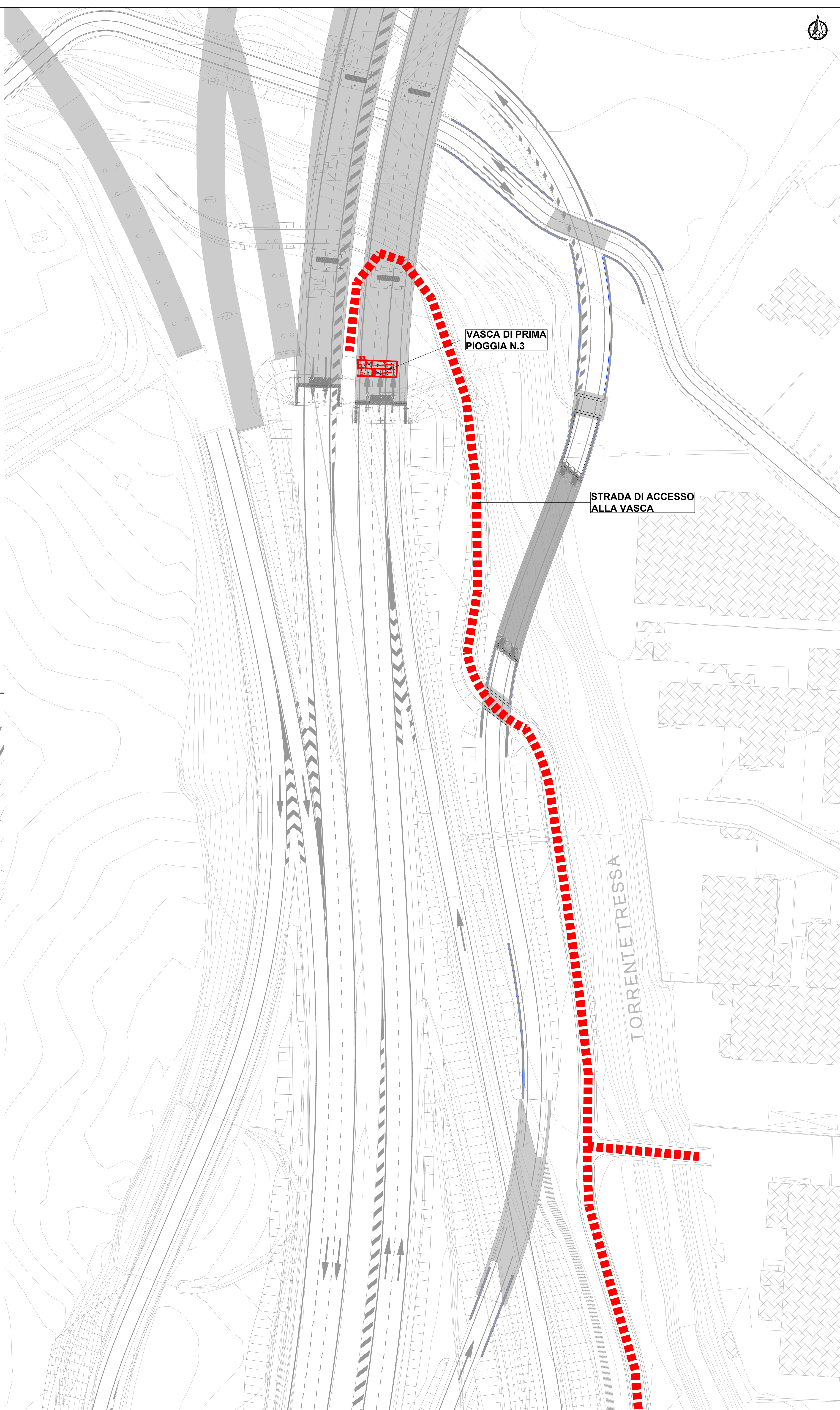
PARTICOLARE ACCESSO VASCA N.3 - SCALA 1:500
