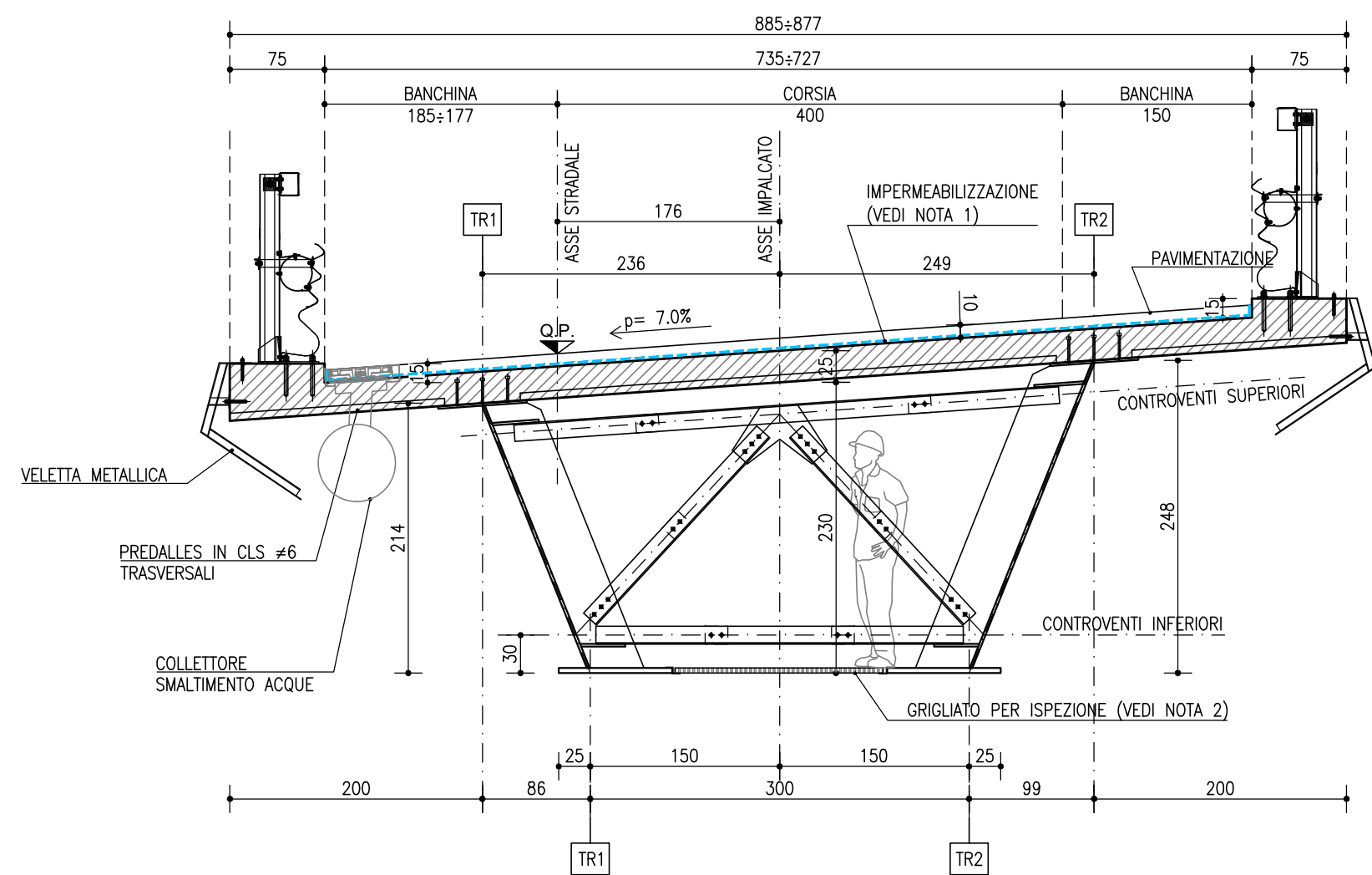
SEZIONE TIPO SCALA 1:50
