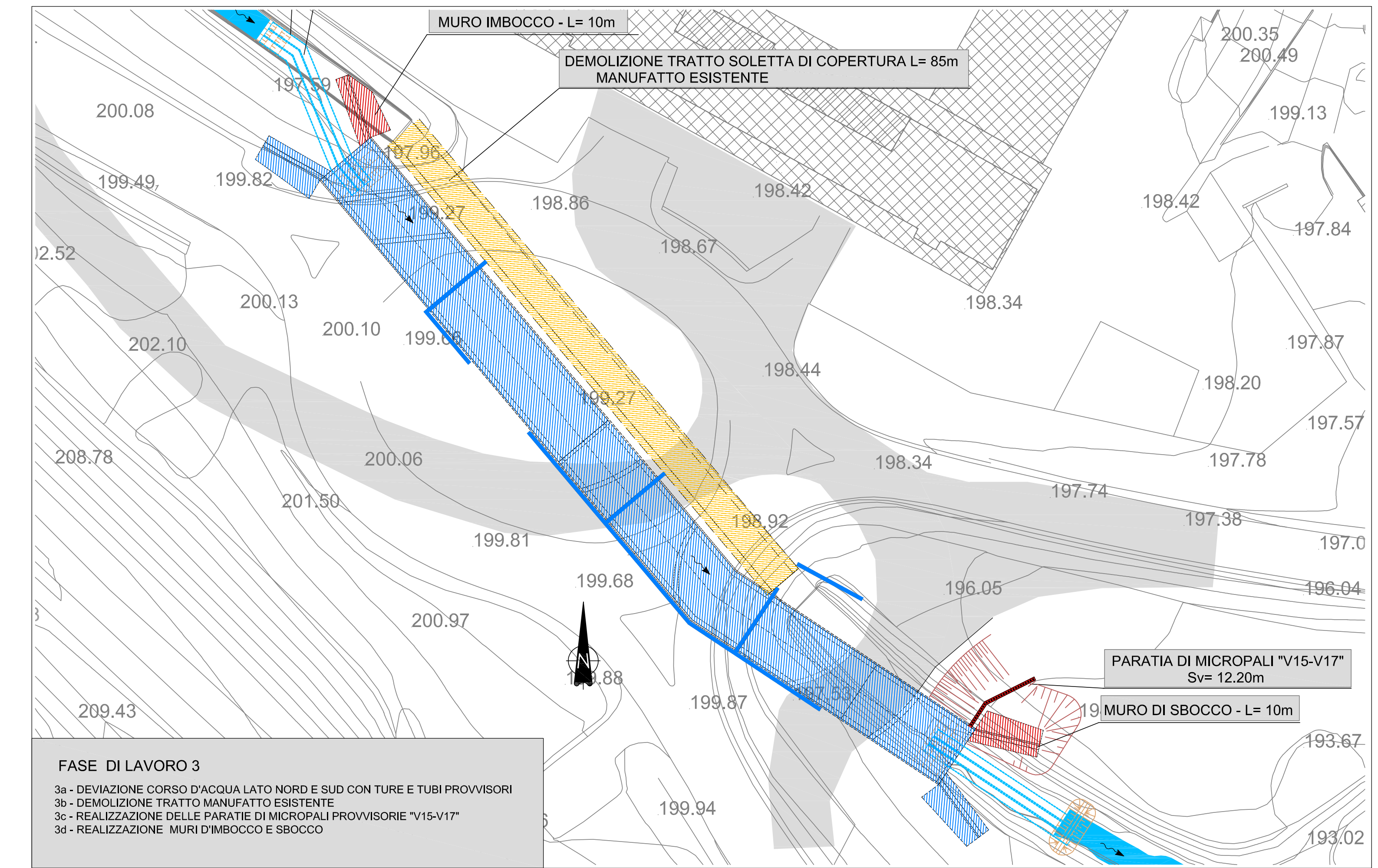
STRALCIO PLANIMETRICO FASE 3 SCALA 1:500
