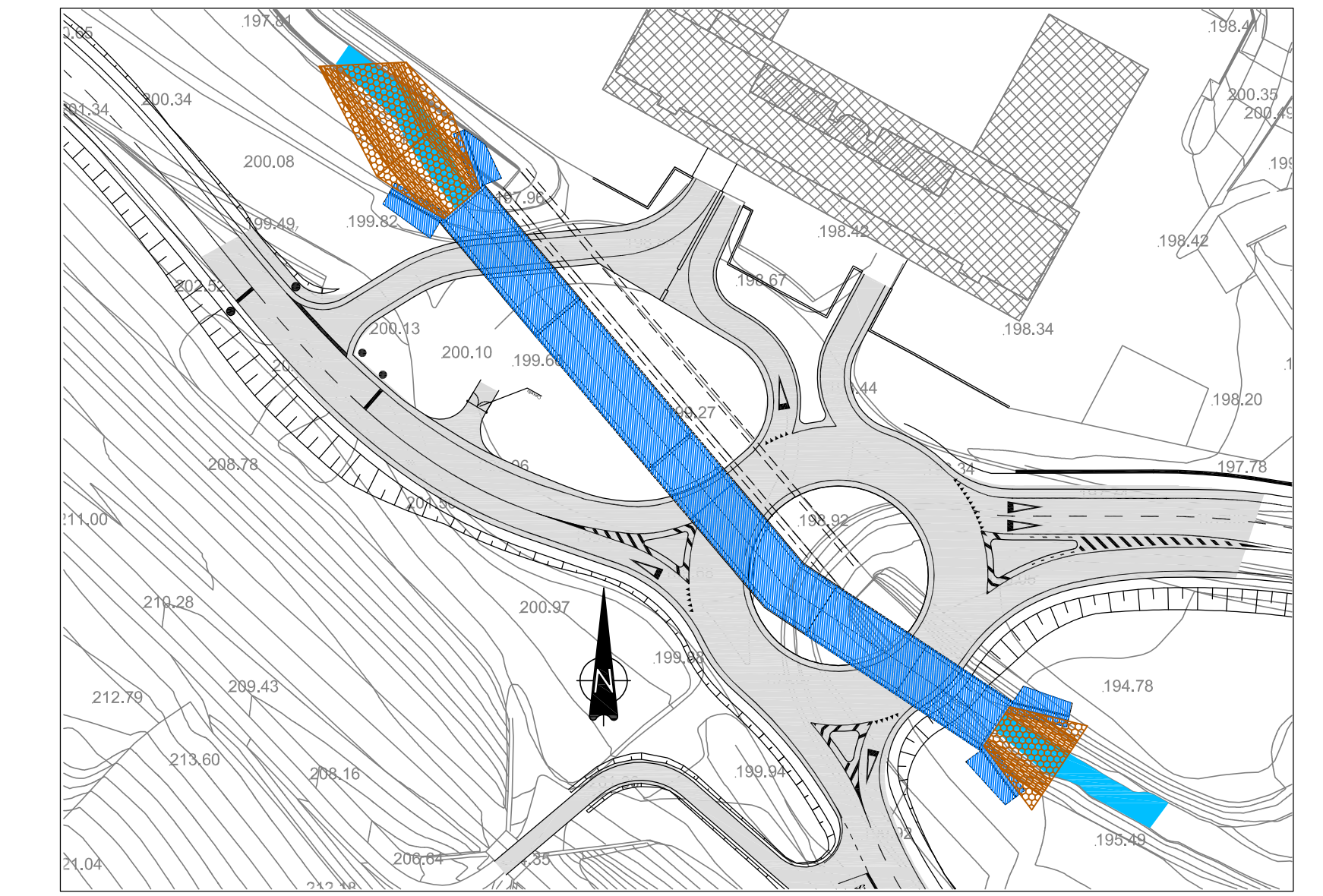
STRALCIO PLANIMETRICO SITUAZIONE DI PROGETTO SCALA 1:1000
