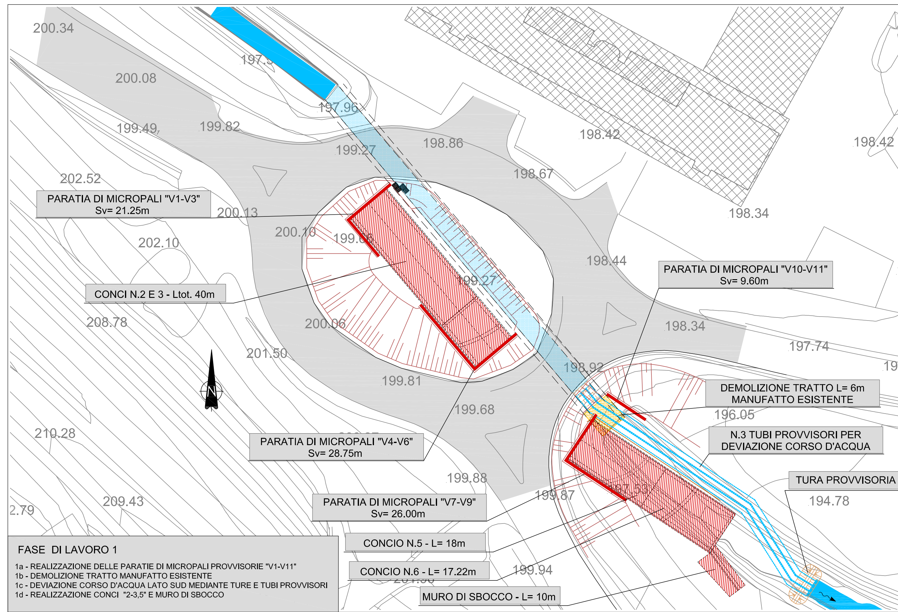
STRALCIO PLANIMETRICO FASE 1 SCALA 1:500
