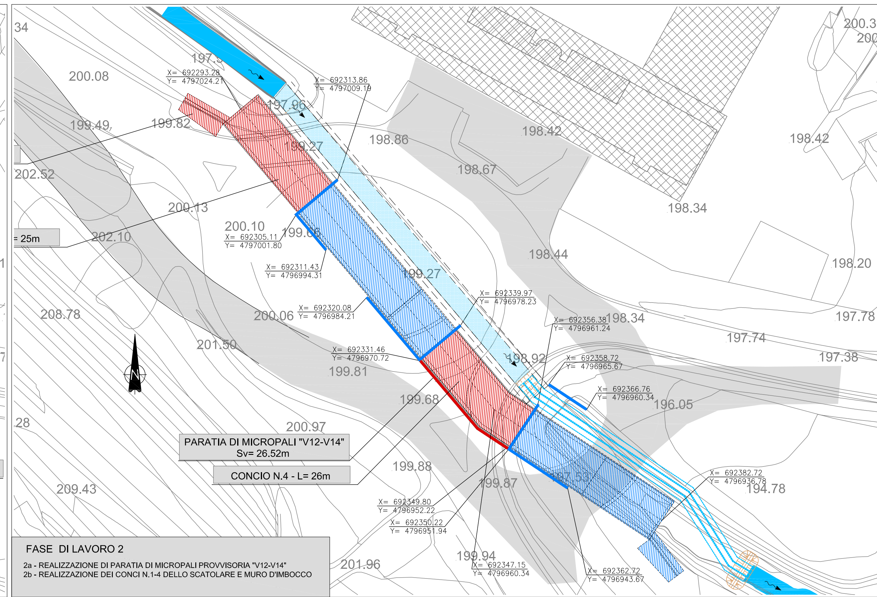
STRALCIO PLANIMETRICO FASE 2 SCALA 1:500
