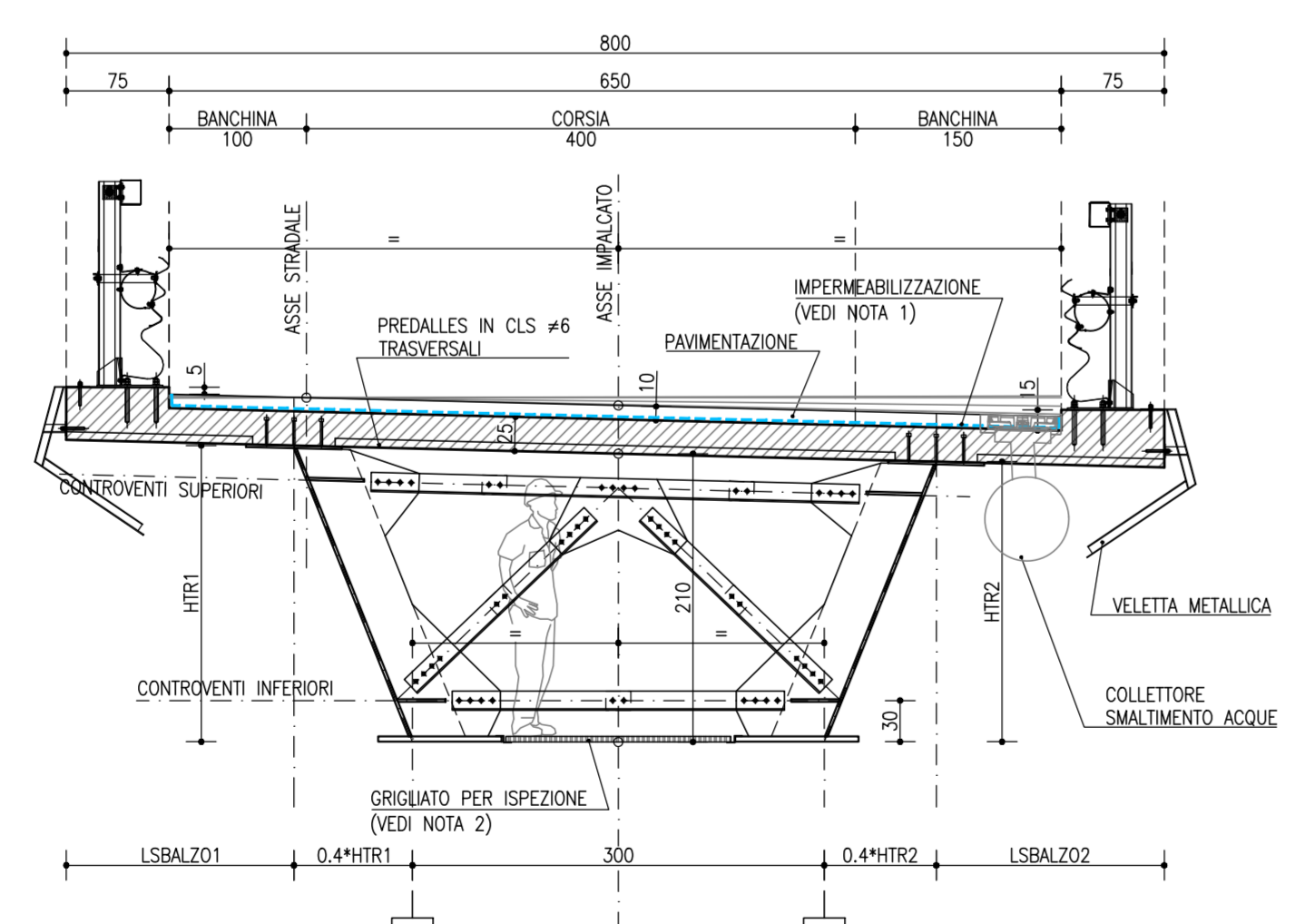
SEZIONE TIPO SCALA 1:50
