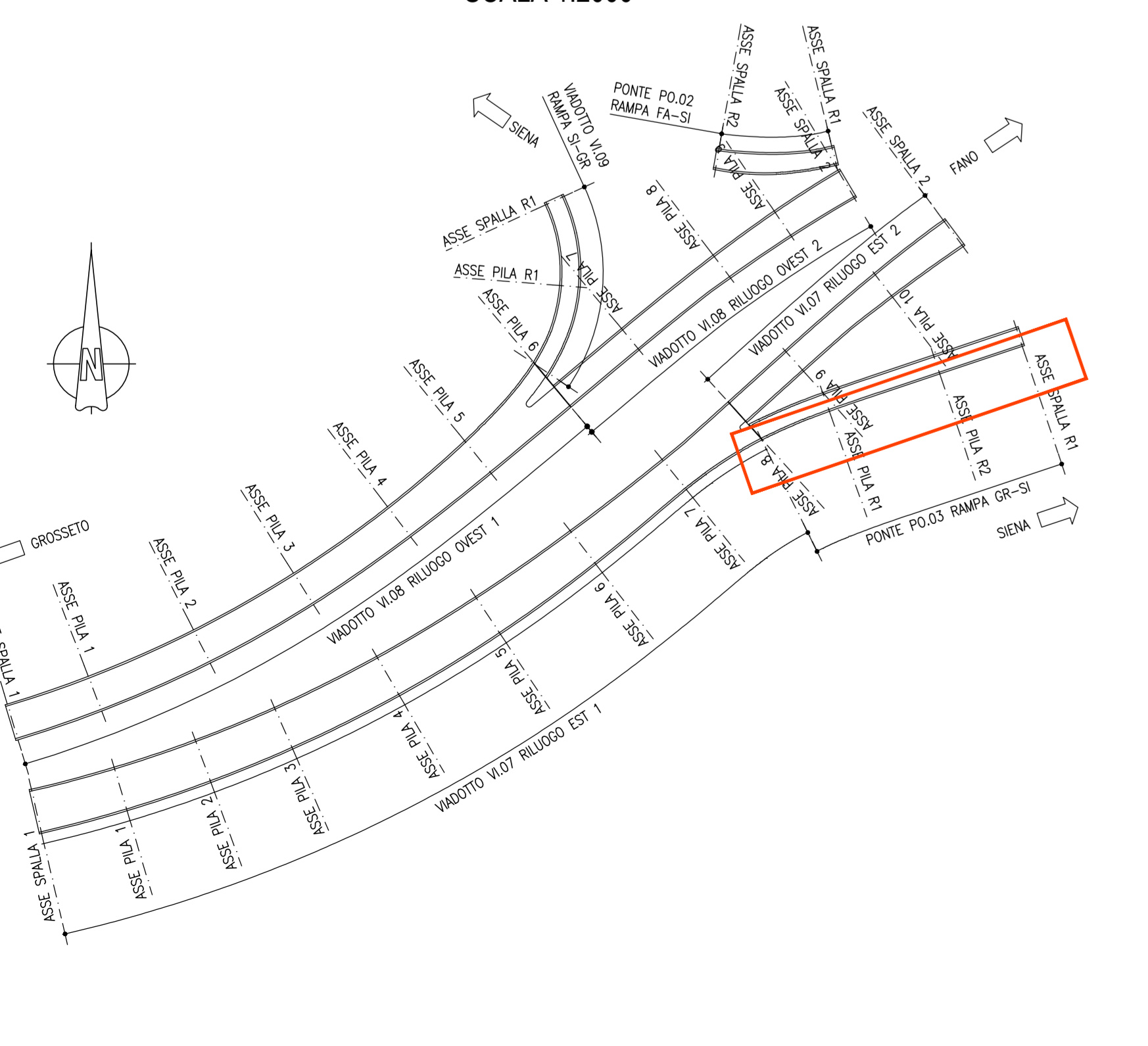
PIANTA CHIAVE SVINCOLO RUFFOLO SCALA 1:2000
