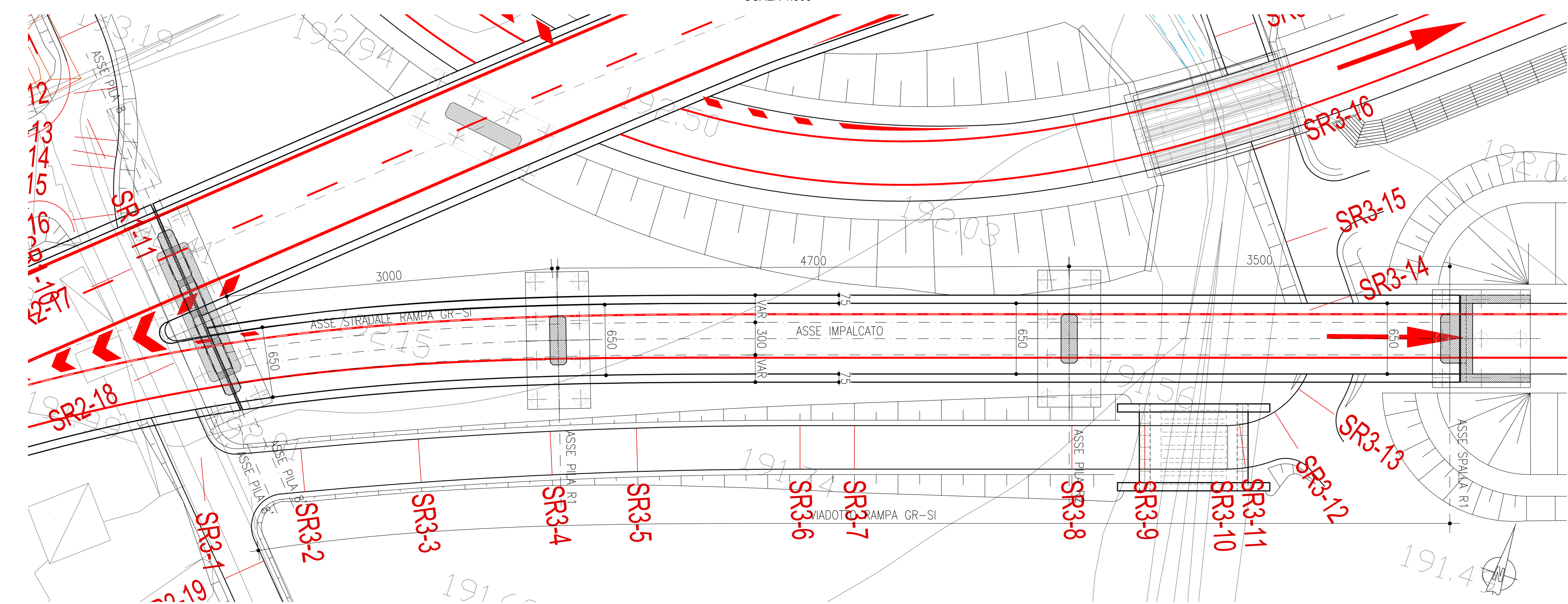
PIANTA GENERALE SCALA 1:500
