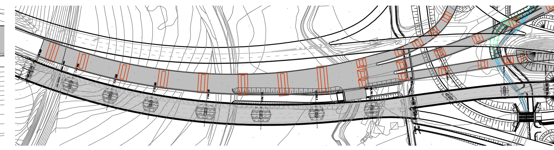
FASE 12 - REALIZZAZIONE SOLETTA E COMPLETAMENTO RILEVATI DI ACCESSO
