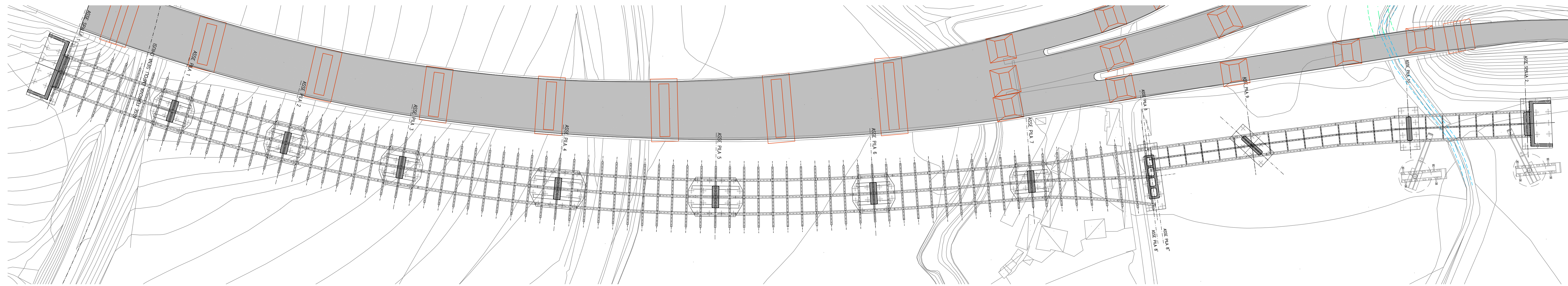
VIADOTTO VI.07 - RILUOGO EST 2 FASE 11 - MONTAGGIO CONCI 9-10-11-12 SCALA 1:500
