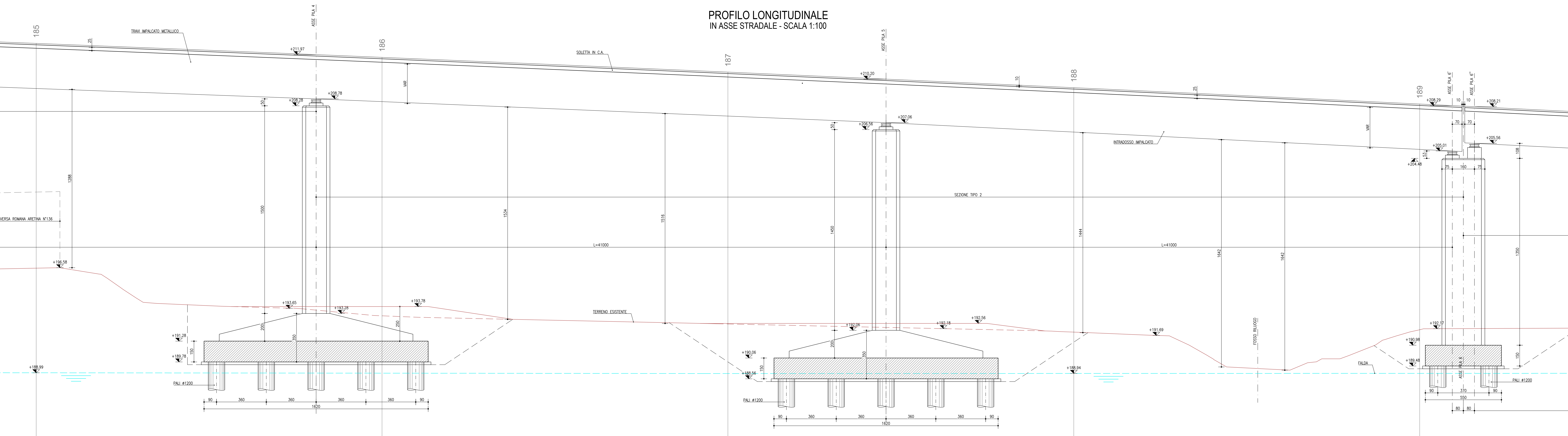
PIANTA GENERALE SCALA 1:500
