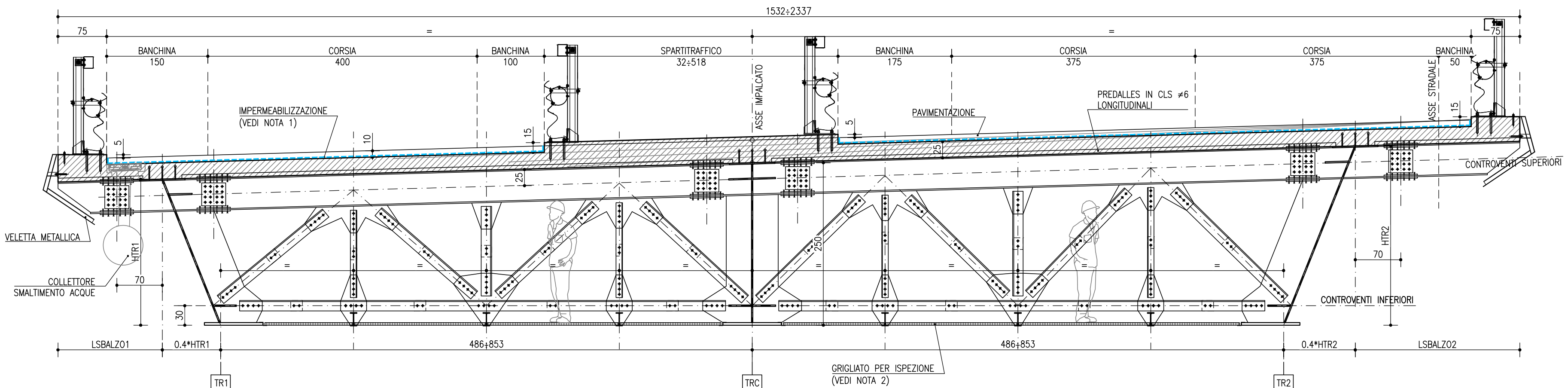
SEZIONE TIPO 3 SCALA 1:50
