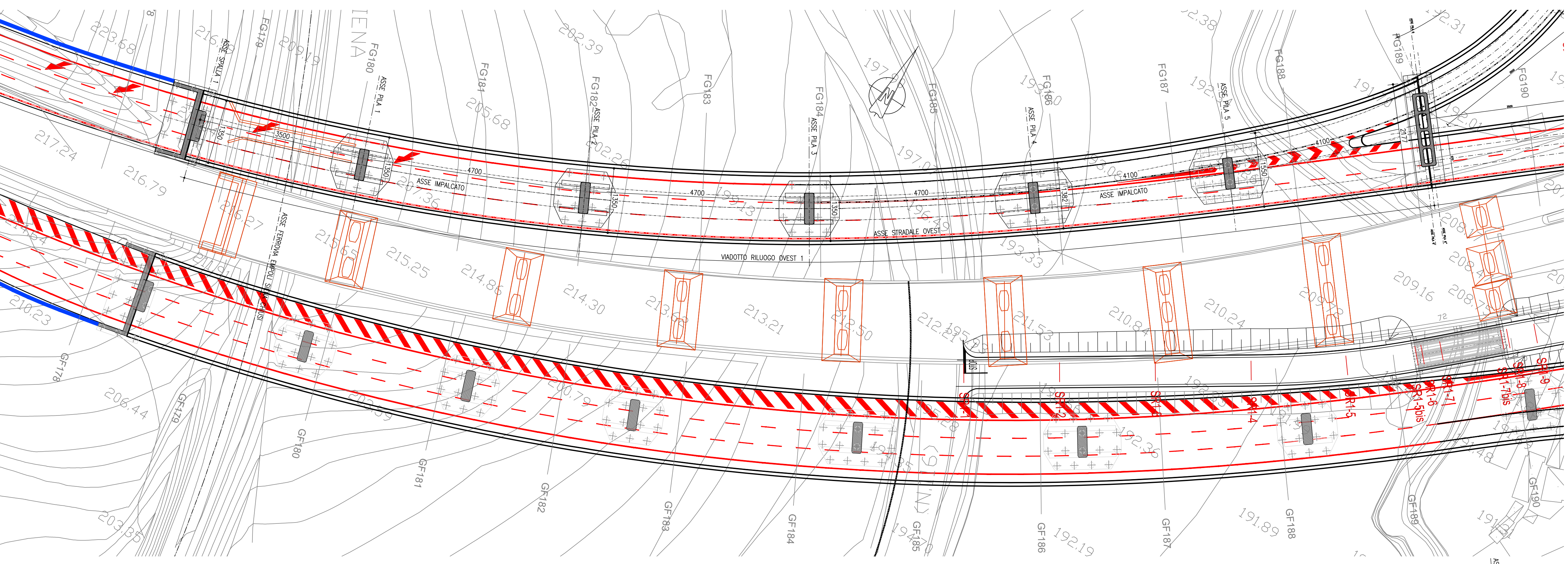
PIANTA SOTTOSTRUTTURE SCALA 1:100
