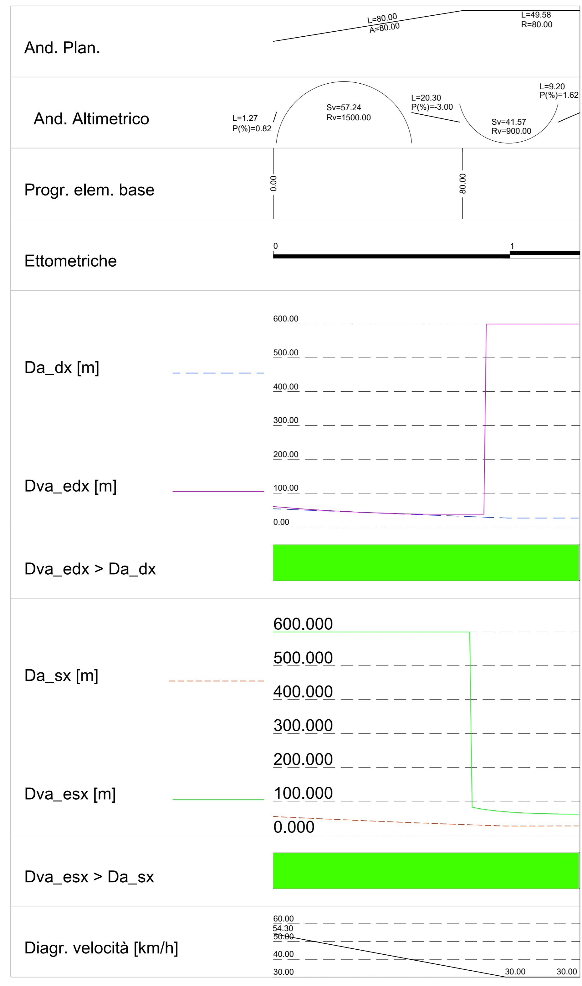
ROTATORIA - RAMO A - senza allargamenti Scala X 1:1000
