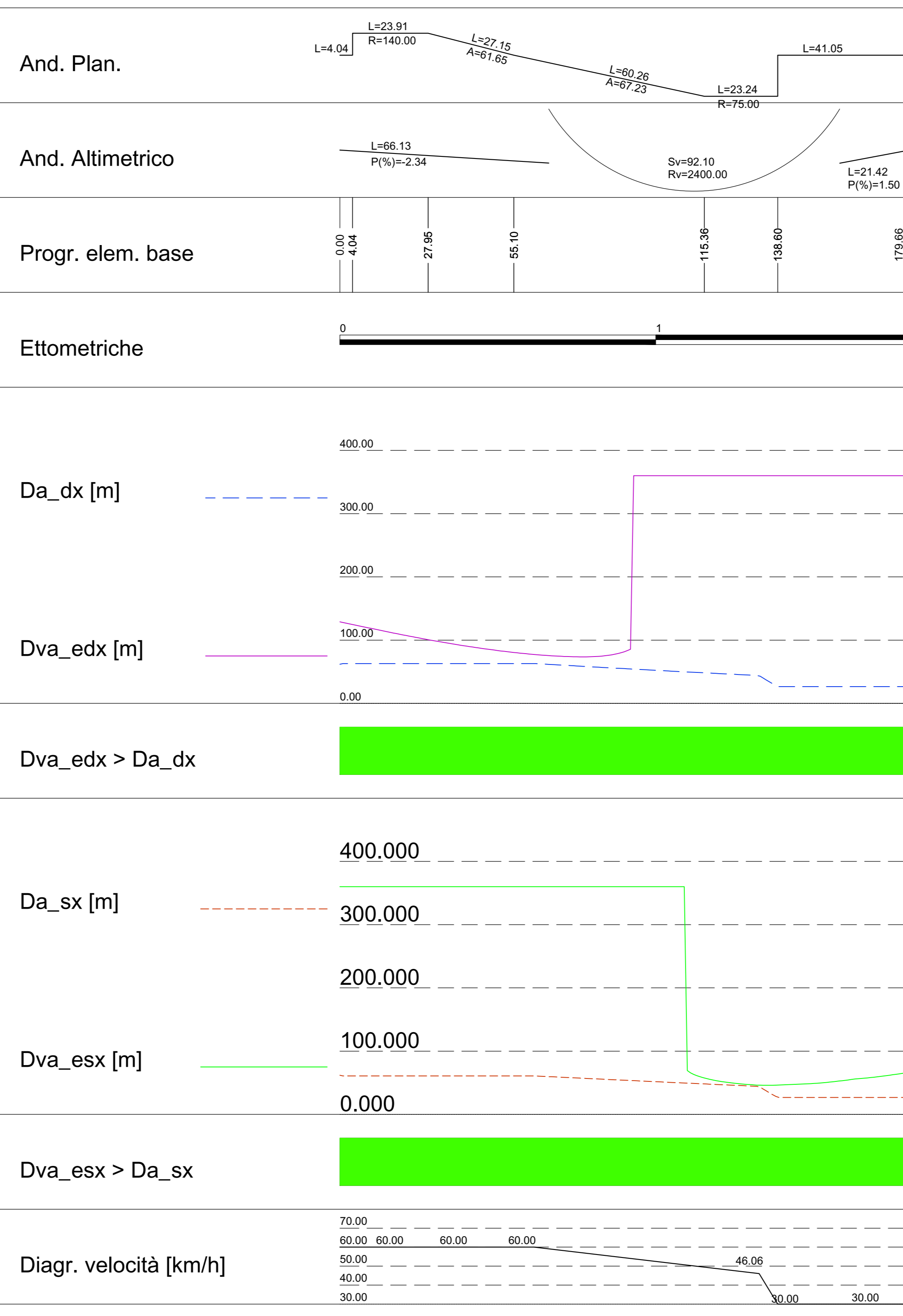
ROTATORIA - RAMO B - senza allargamenti Scala X 1:1000
