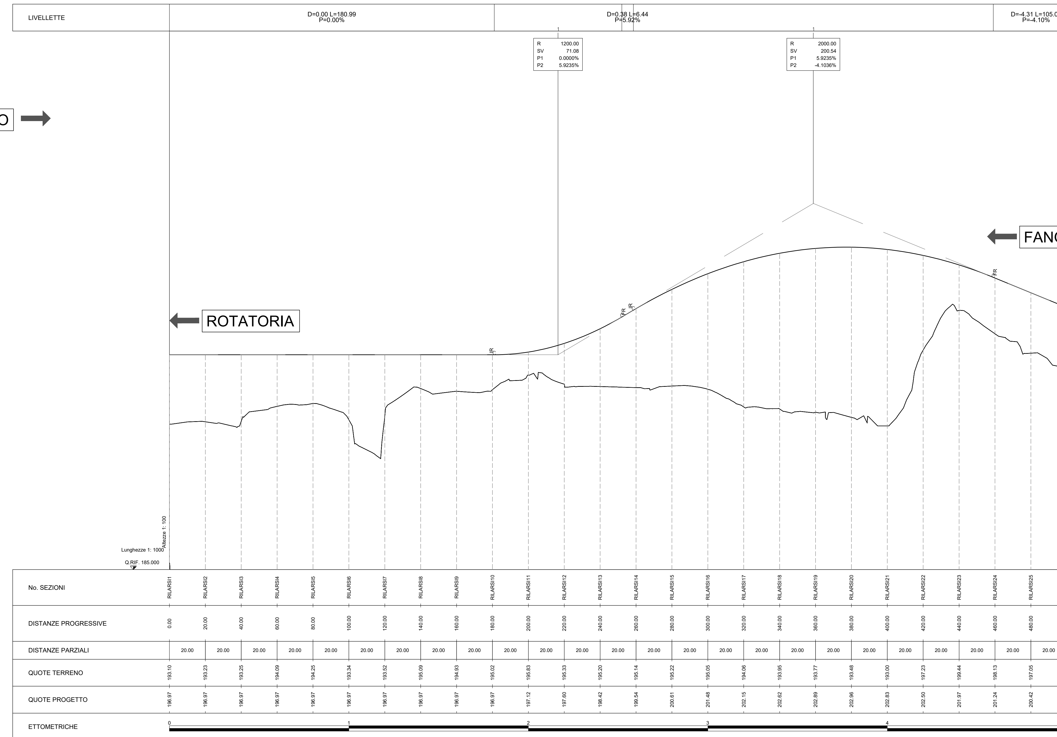
Svincolo di Ruffolo - Alternativa 3 - Profili Longitudinali Rampe Carreggiata Ovest
