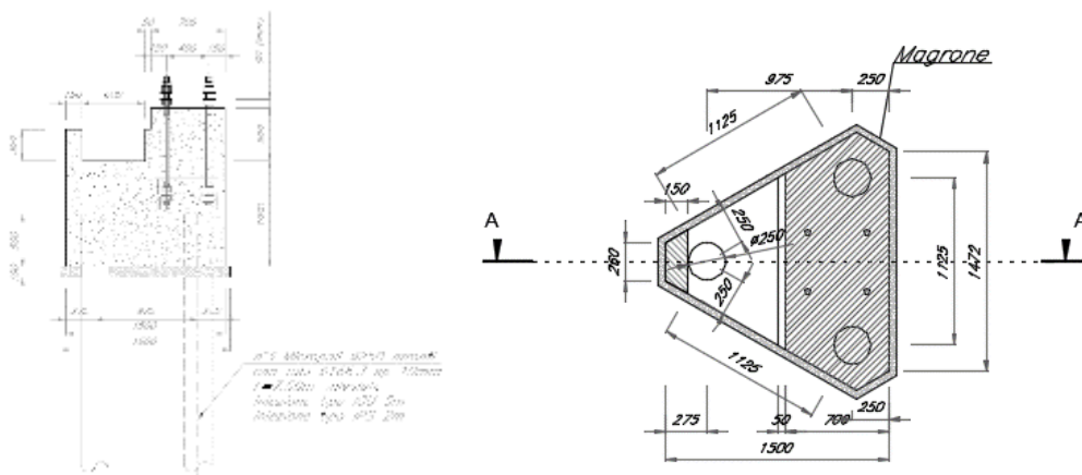
Figura 22 - Fondazioni per pali LSU – Sezione tipologica in trincea singolo binario – Carpenteria blocco
