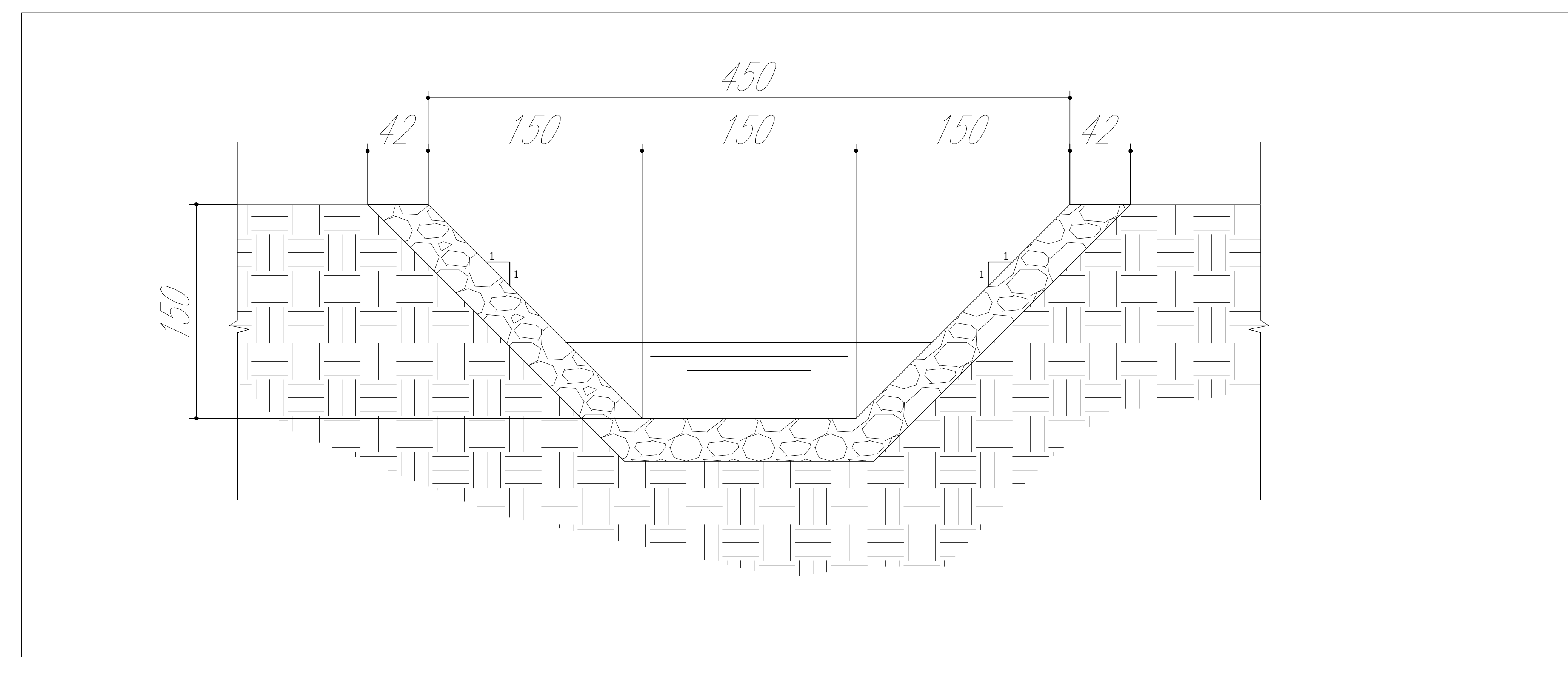
SEZIONE TIPO
