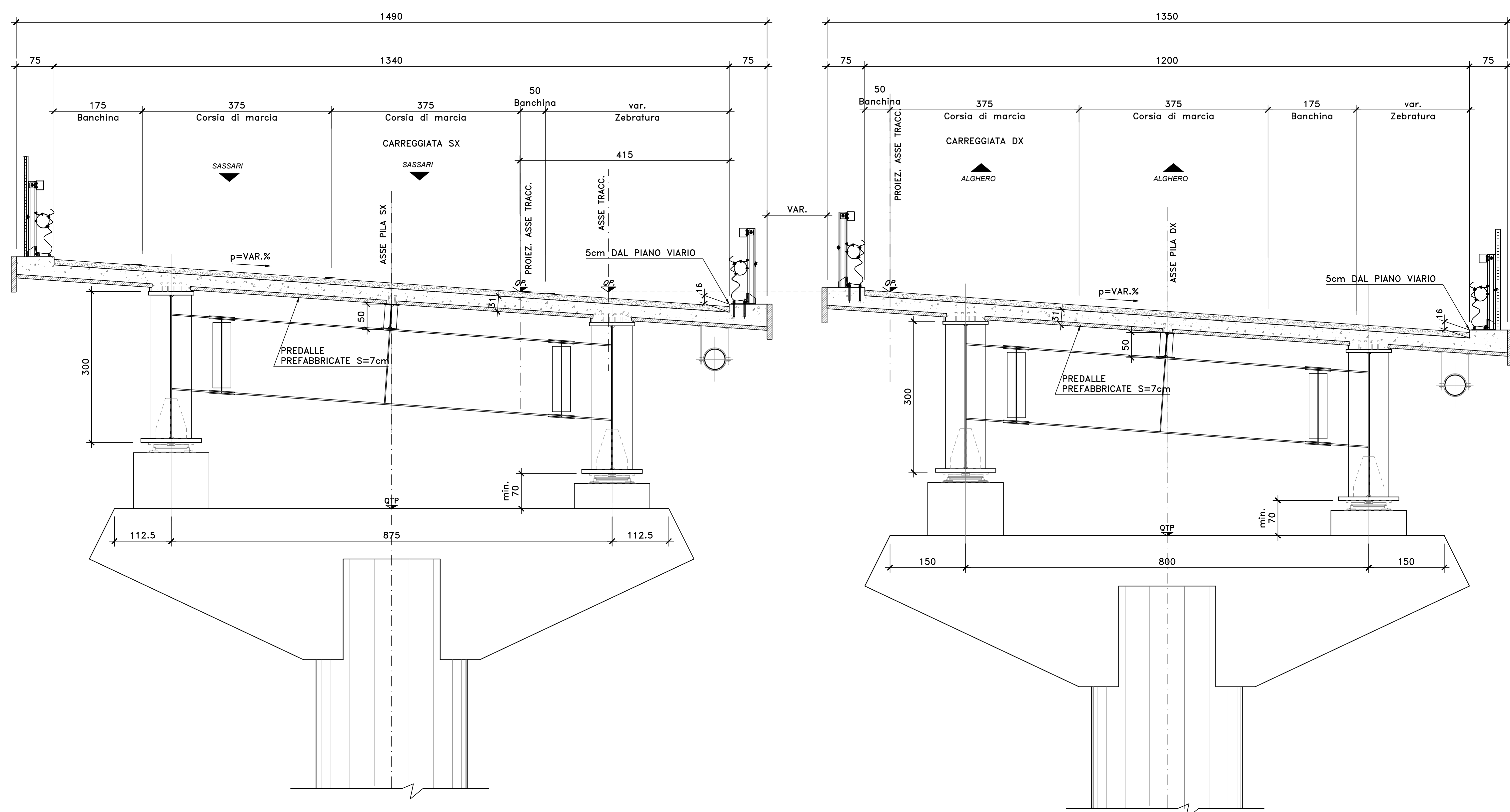
SEZIONE TRASVERSALE IN ASSE PILE (PONTE RIO CALVIA 1) SCALA 1:50
