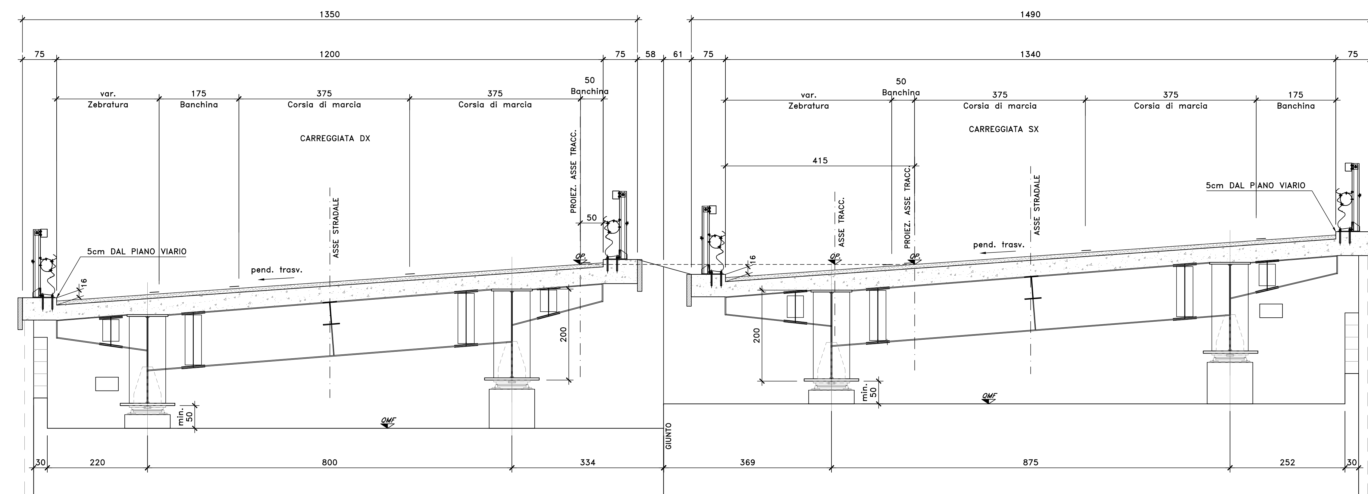
SEZIONE TRASVERSALE IN ASSE SPALLA A dx-sx SCALA 1:50
