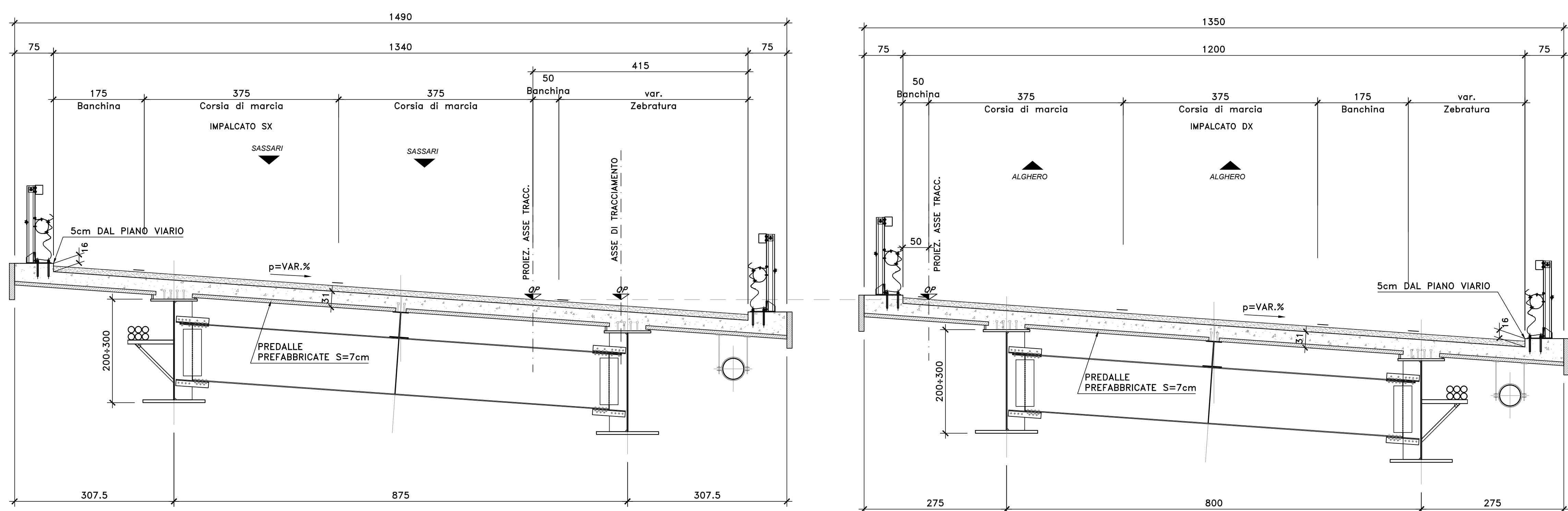
SEZIONE TRASVERSALE IN CAMPATA (PONTE RIO CALVIA 1) SCALA 1:50
