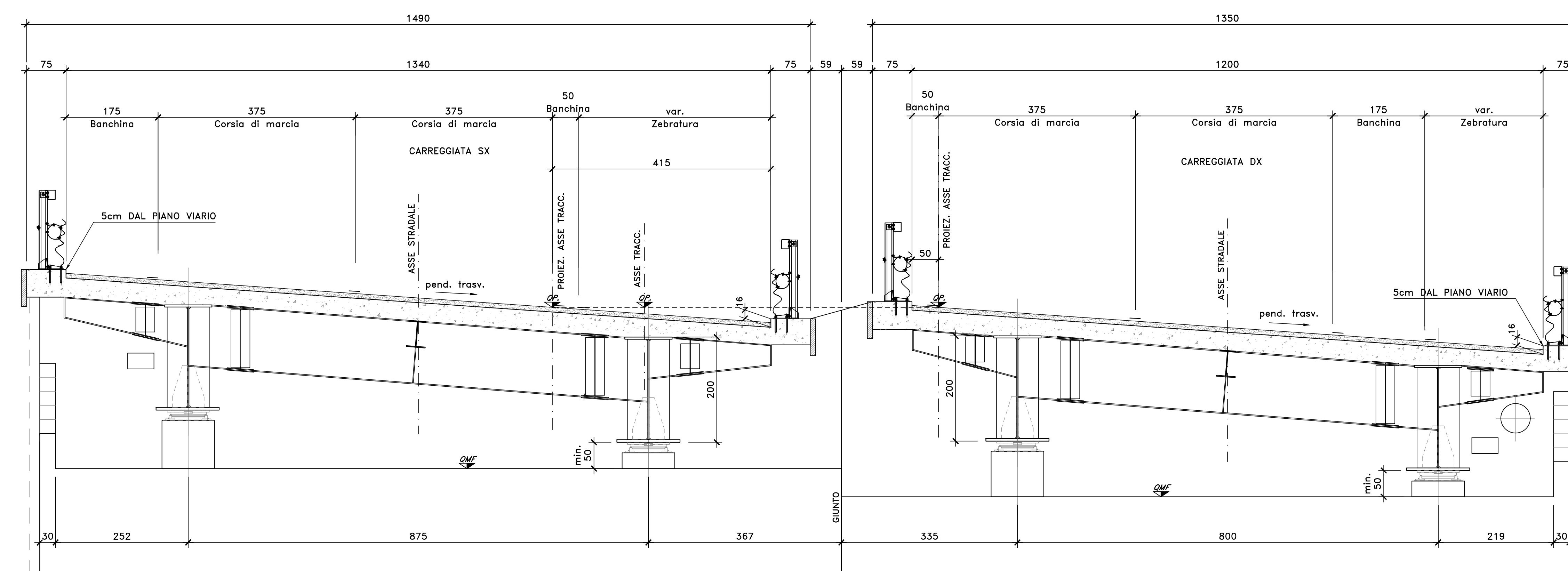
SEZIONE TRASVERSALE IN ASSE SPALLA B dx-sx SCALA 1:50
