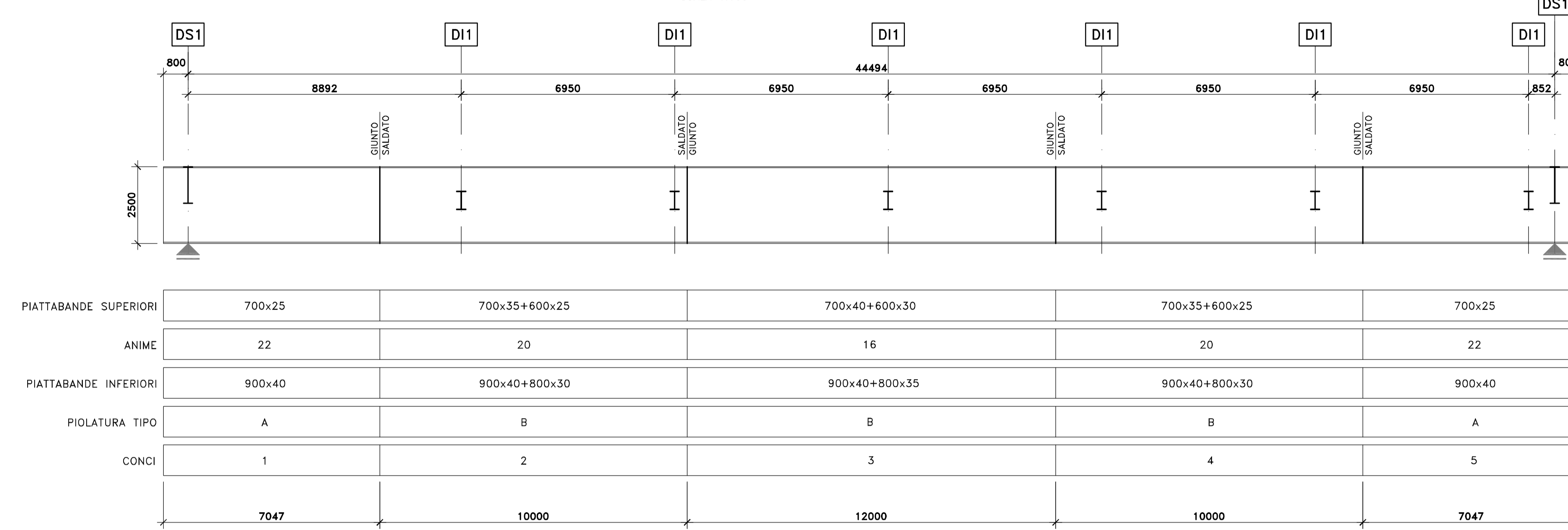
SEZIONE LONGITUDINALE TRAVI IMPALCATO DX SCALA 1:100
