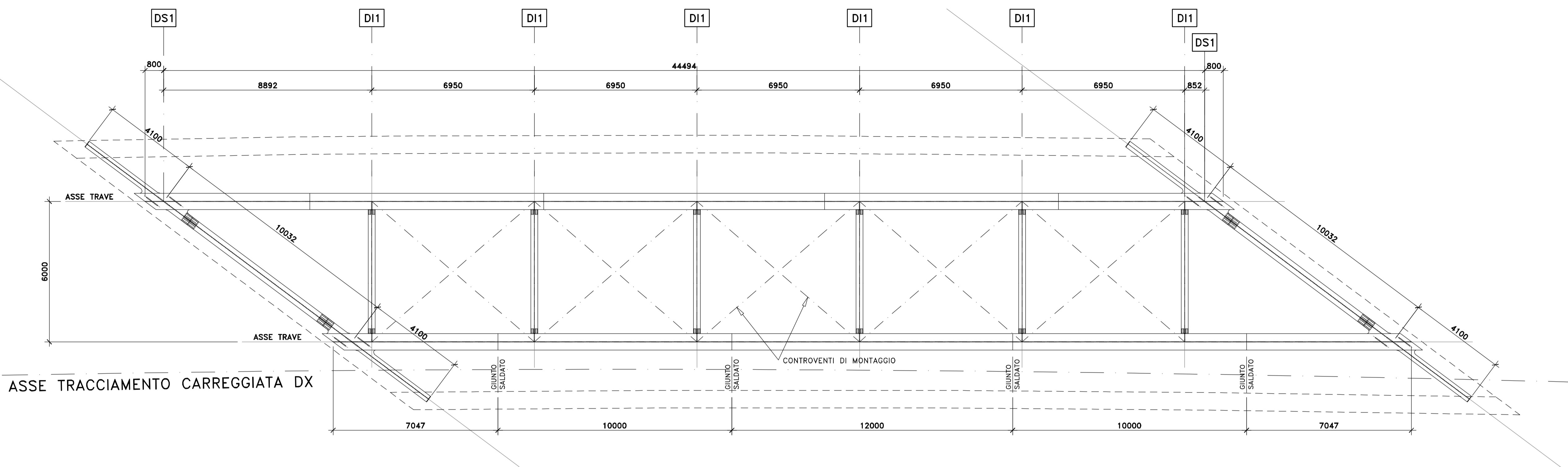
PIANTA IMPALCATO CARREGGIATA DX SCALA 1:100
