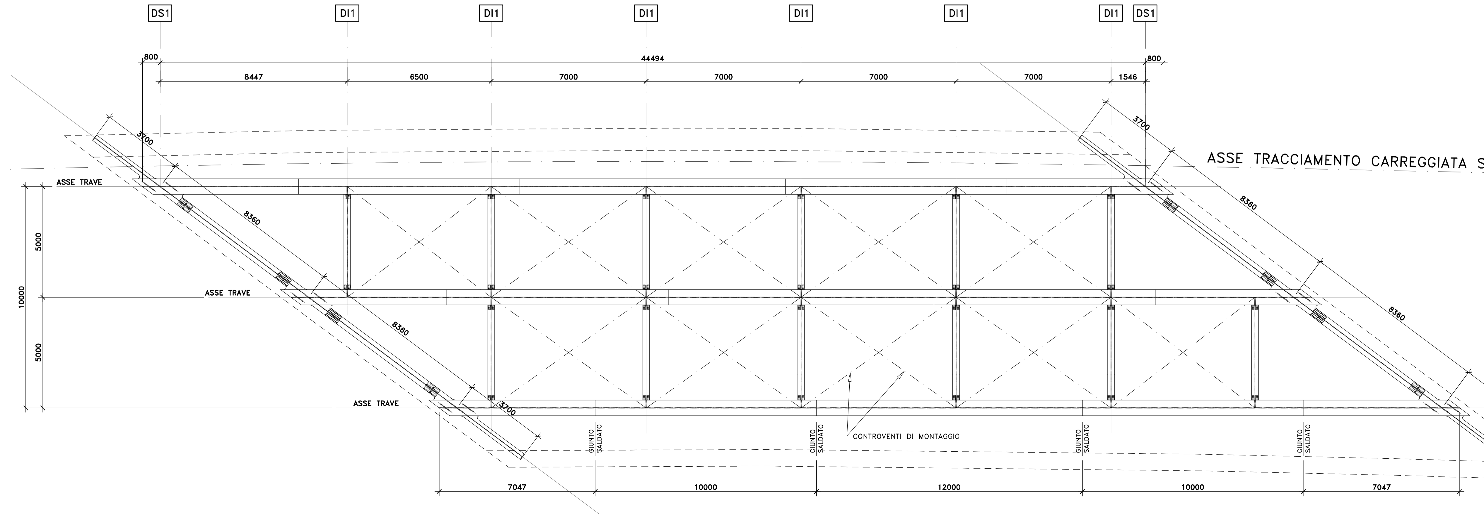
PIANTA IMPALCATO CARREGGIATA SX SCALA 1:100
