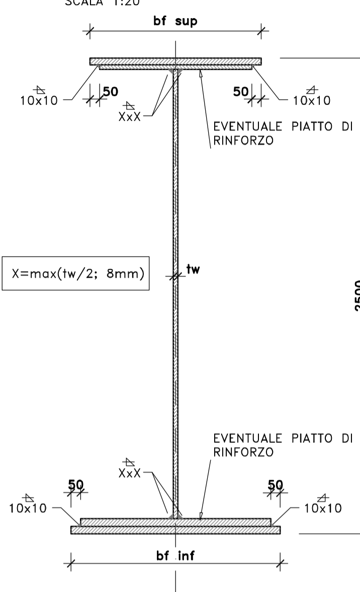
SCHEMA TRAVE COMPOSTA SALDATA SCALA 1:20
