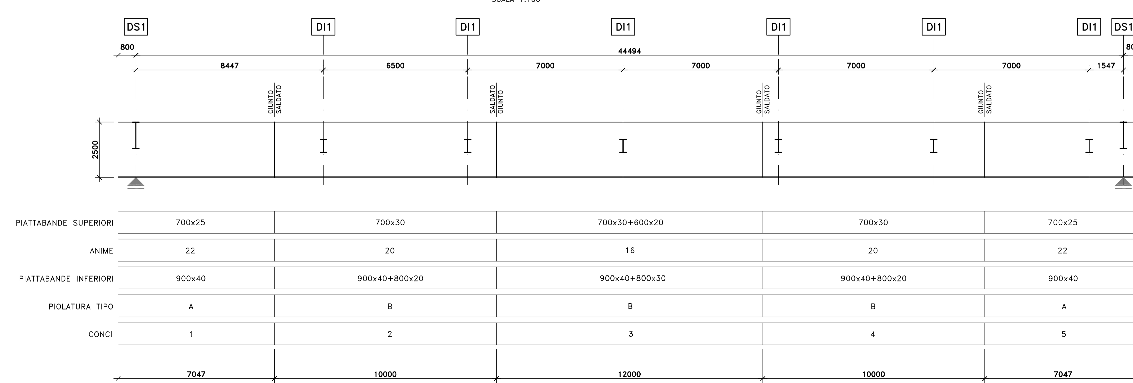
SEZIONE LONGITUDINALE TRAVI IMPALCATO SX SCALA 1:100
