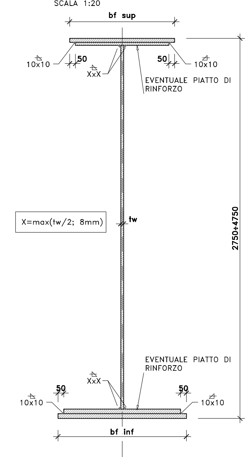
SCHEMA TRAVE COMPOSTA SALDATA SCALA 1:20
