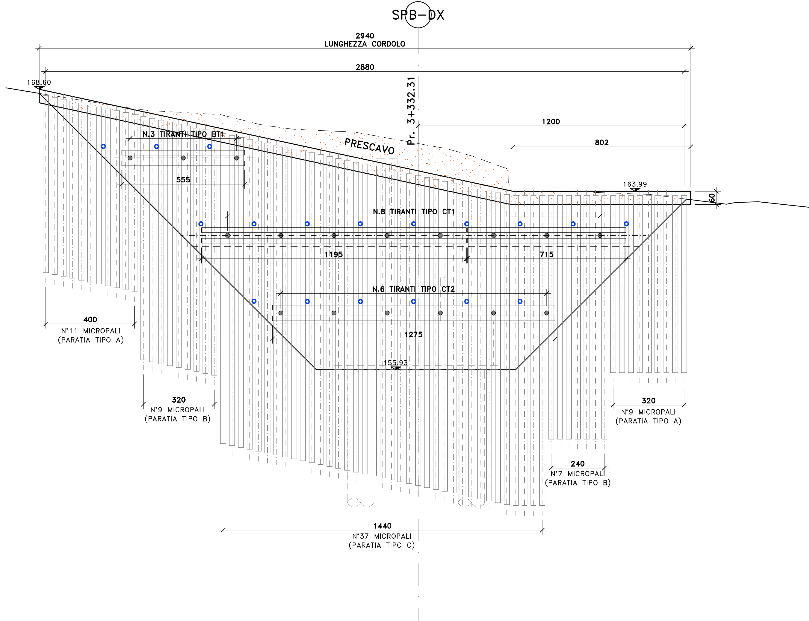
PROSPETTO PARATIA SPALLA B DX LATO SS-131 (1^FASE) SCALA 1:100
