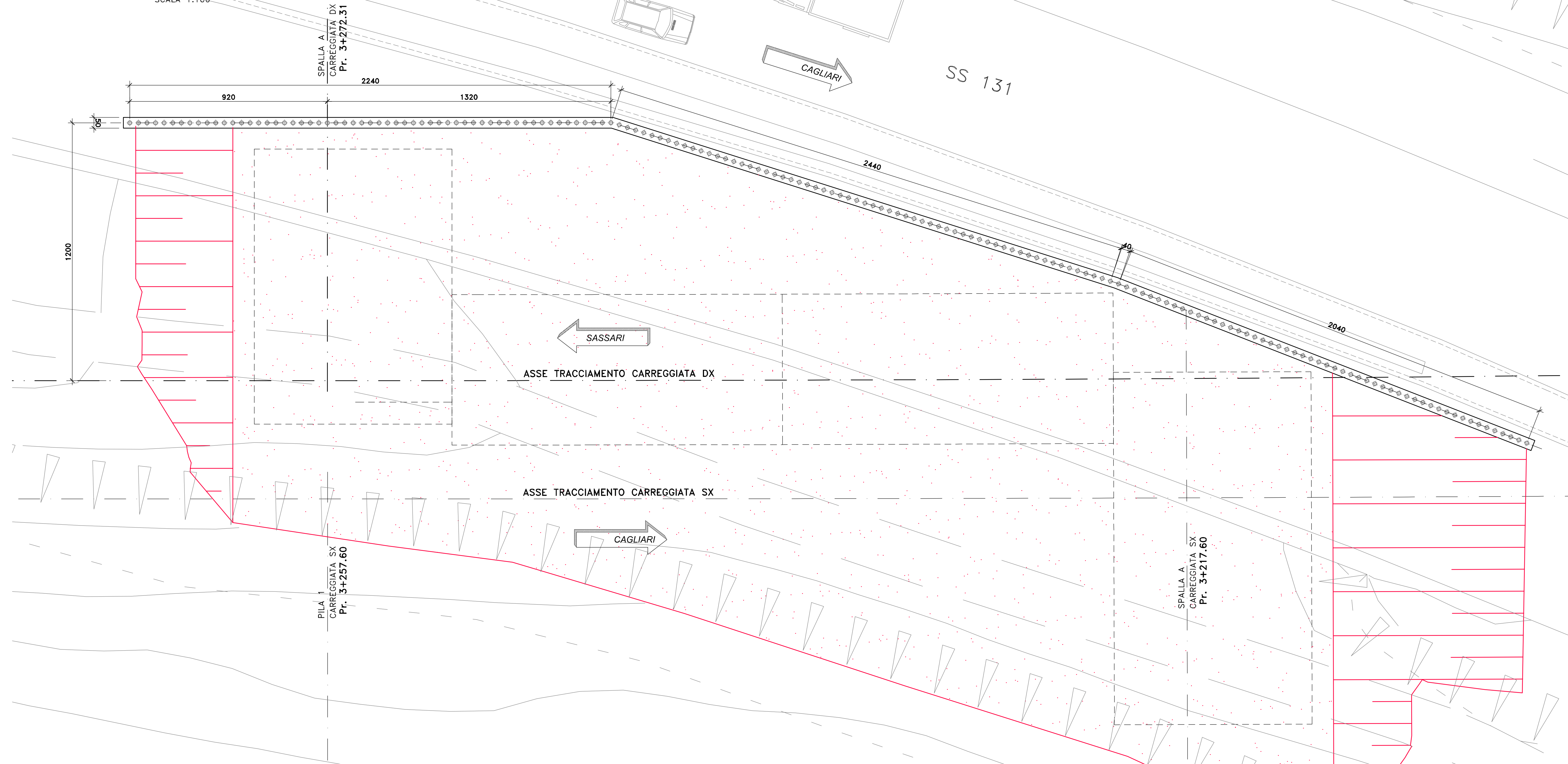
PIANTA PARATIA SPALLA A DX-SPALLA A SX LATO SS-131 (1^FASE) SCALA 1:100
