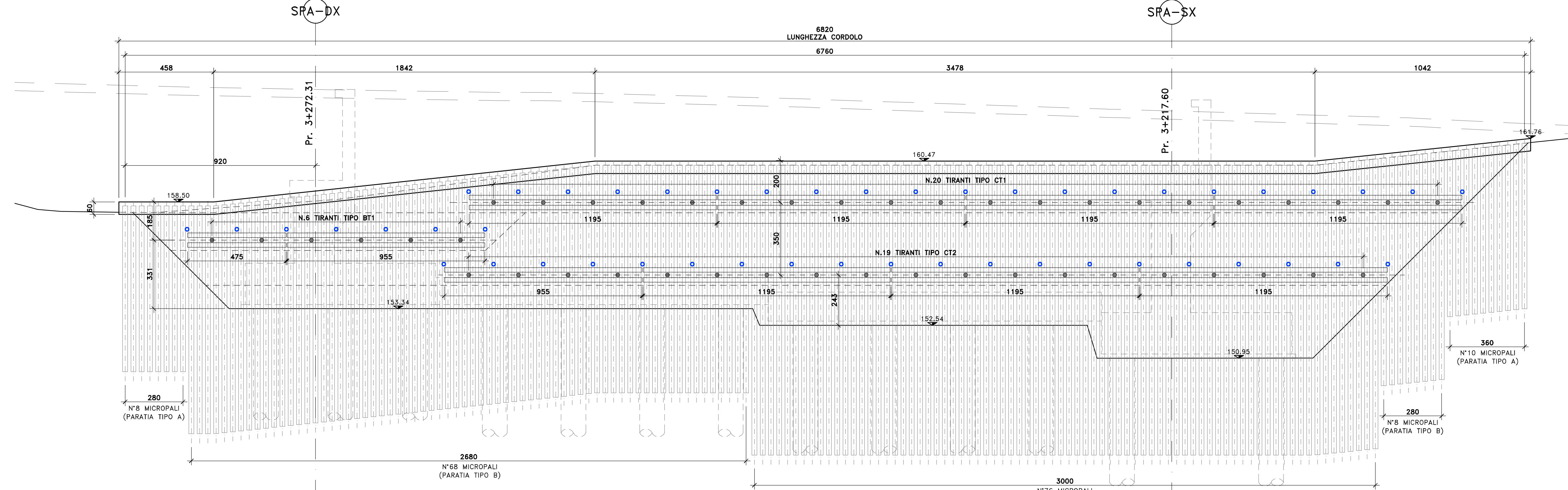
PROSPETTO PARATIA SPALLA A DX-SPALLA A SX LATO SS-131 (1^FASE) SCALA 1:100
