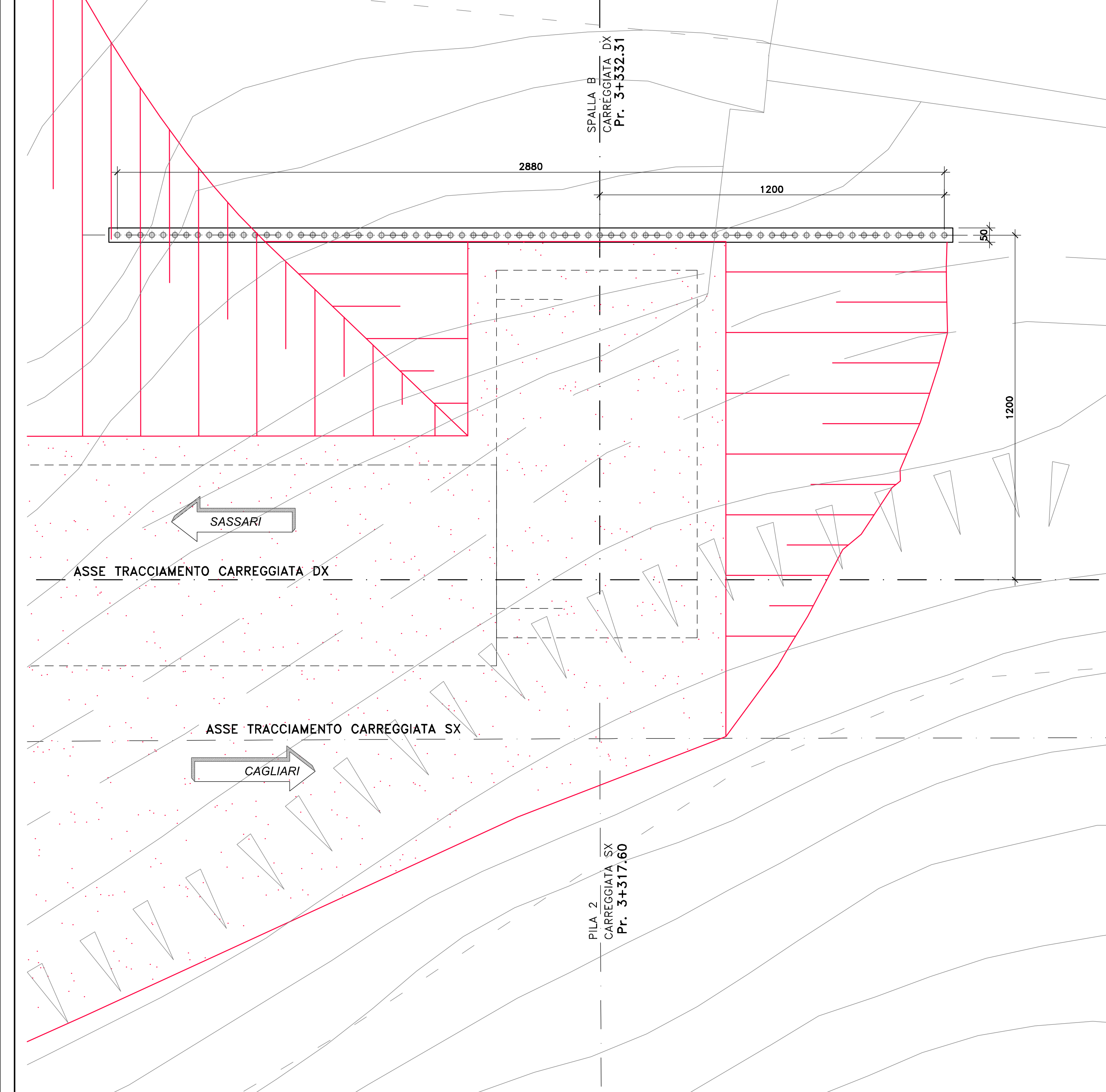
PIANTA PARATIA SPALLA B DX LATO SS-131 (1^FASE) SCALA 1:100
