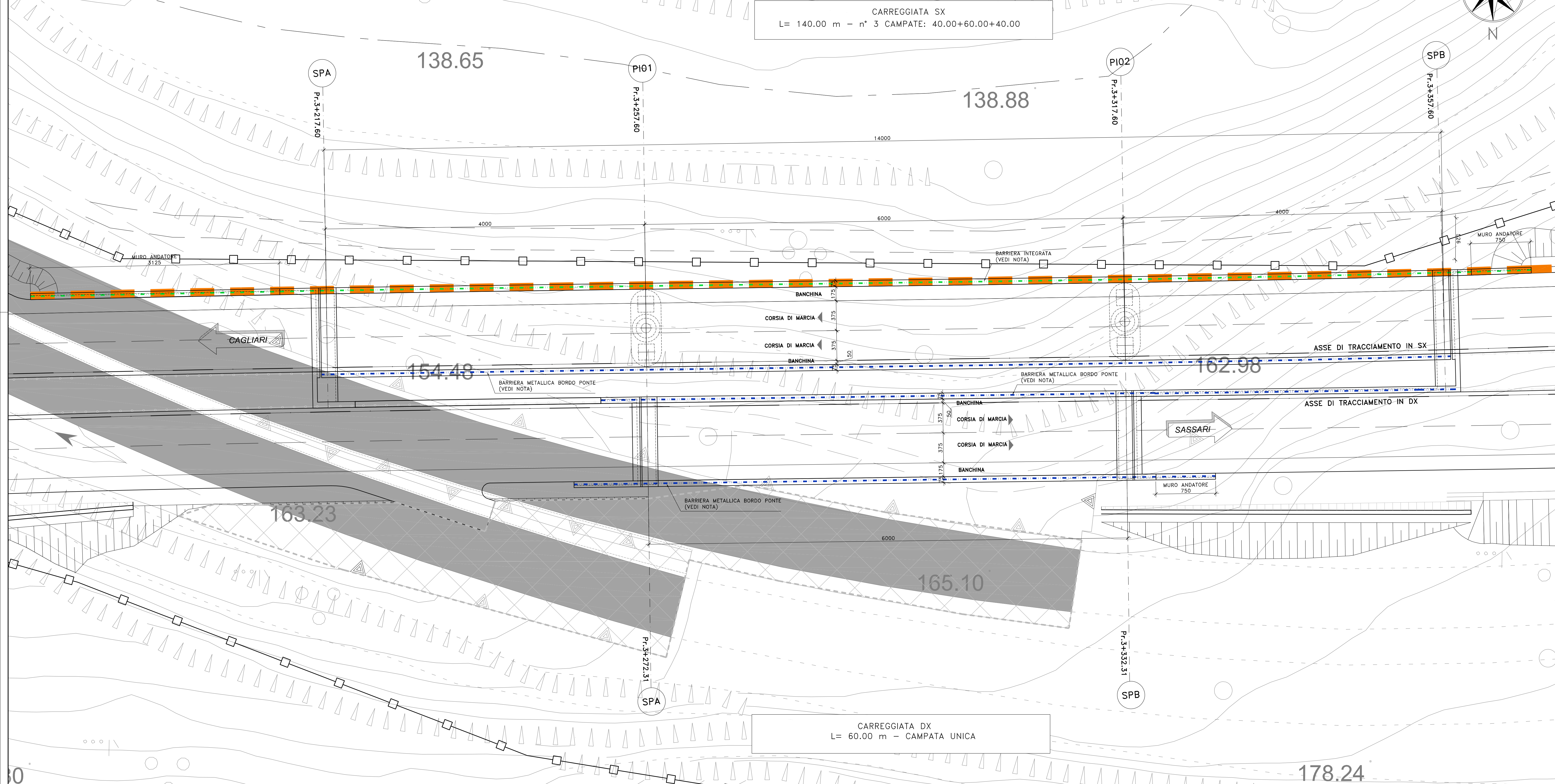
PROSPETTO CAREGGIATA SX scala 1:200
