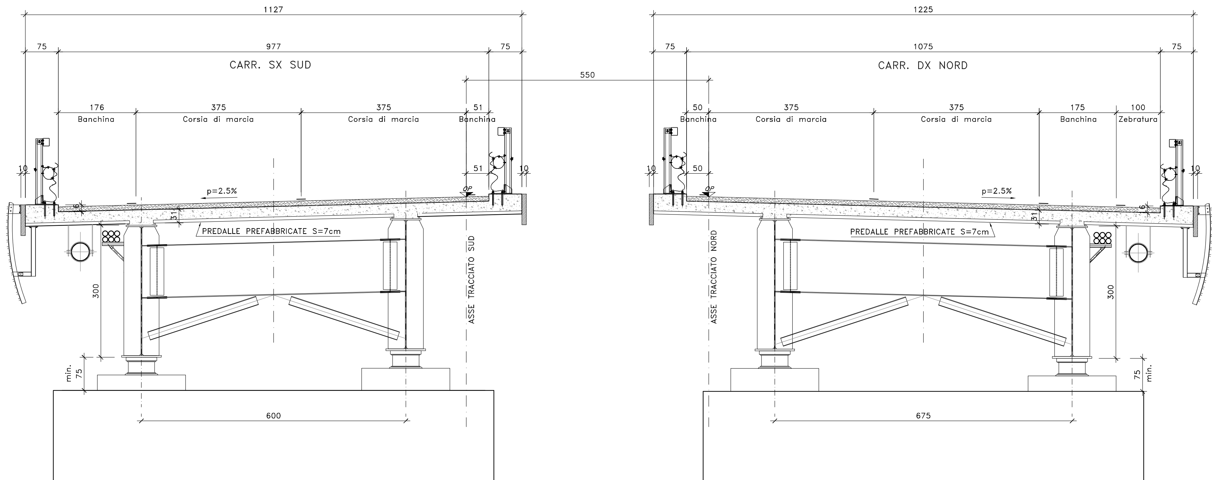
SEZIONE TRASVERSALE IN PILA (VI06) GIUNCHEDDU
