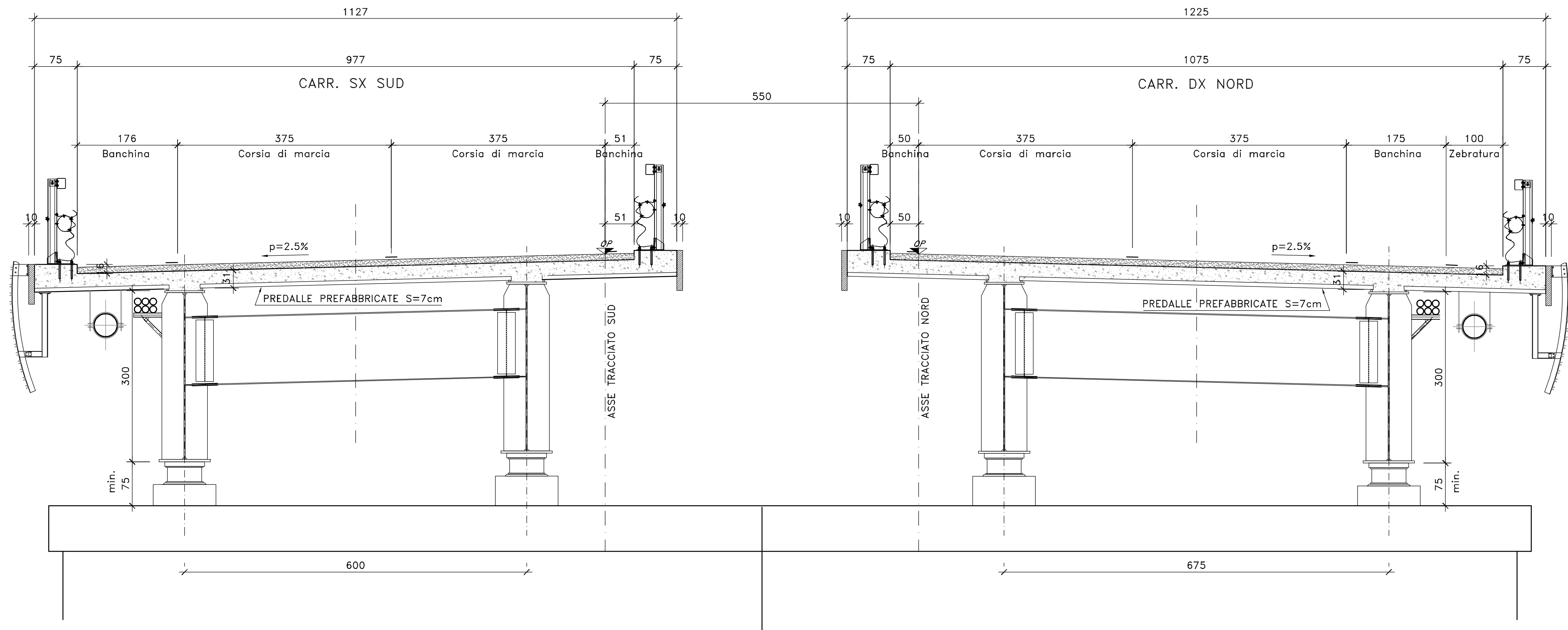
SEZIONE TRASVERSALE ASSE SPALLA (VI06) GIUNCHEDDU
