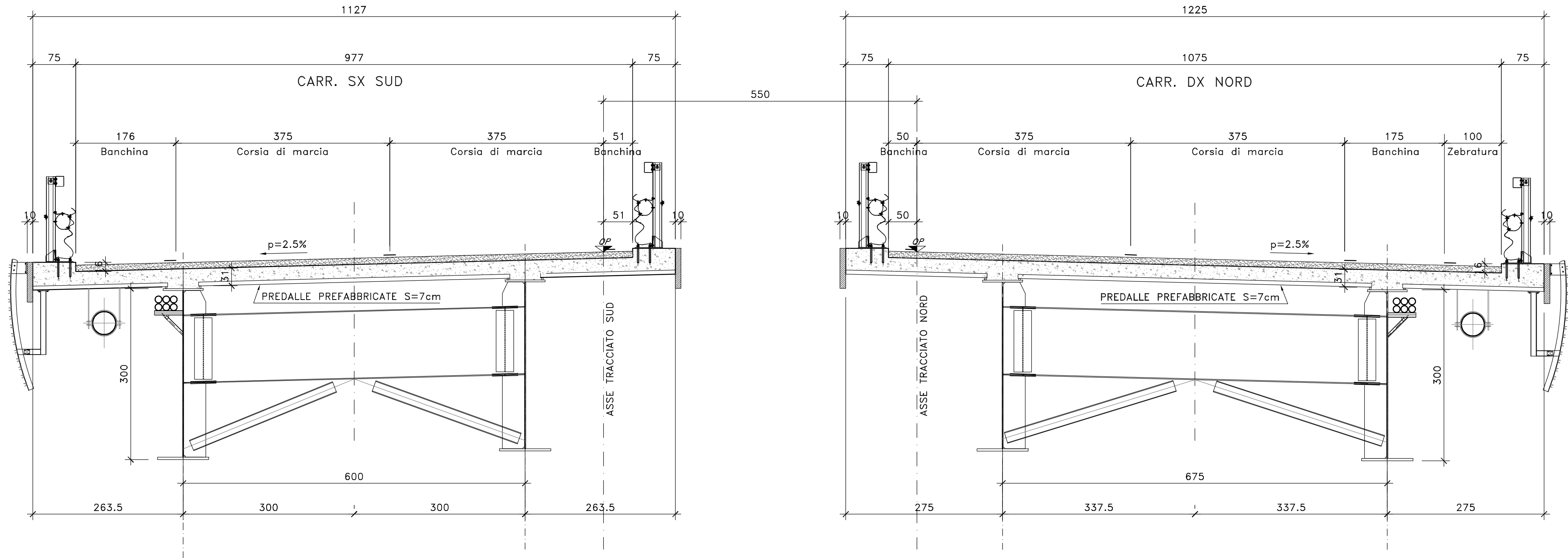
SEZIONE TRASVERSALE IN CAMPATA (VI06) GIUNCHEDDU
