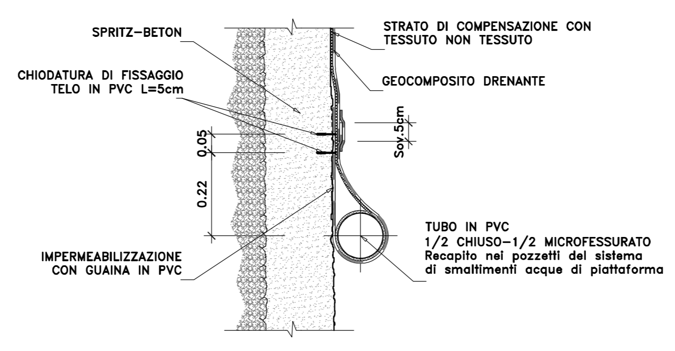
PARTICOLARE DRENAGGIO Scala 1:10
