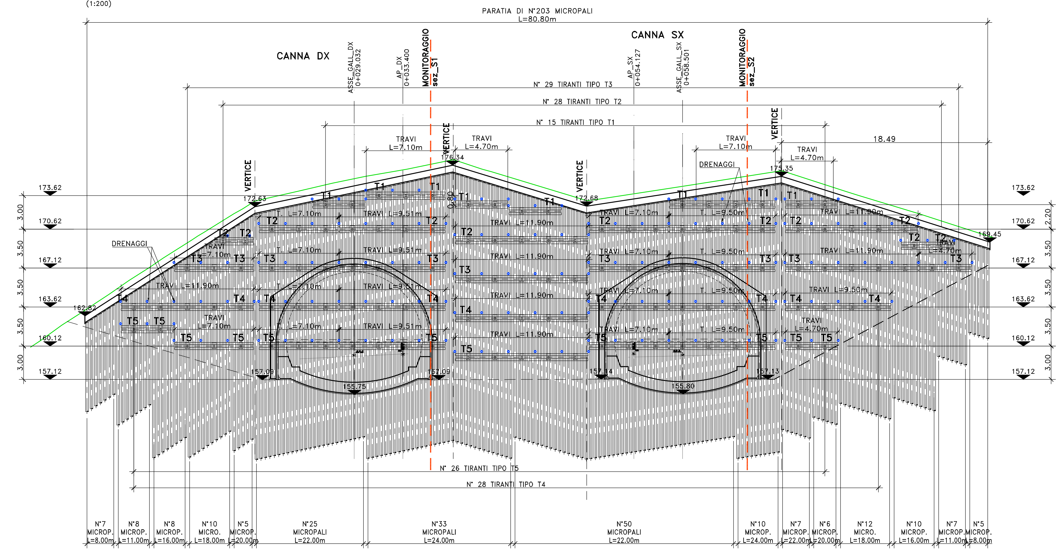
GALLERIA PALA SOLIANA – IMBOCCO LATO SASSARI PARATIA PROVVISORIALE DI MICROPALI SVILUPPATA (1:200)
