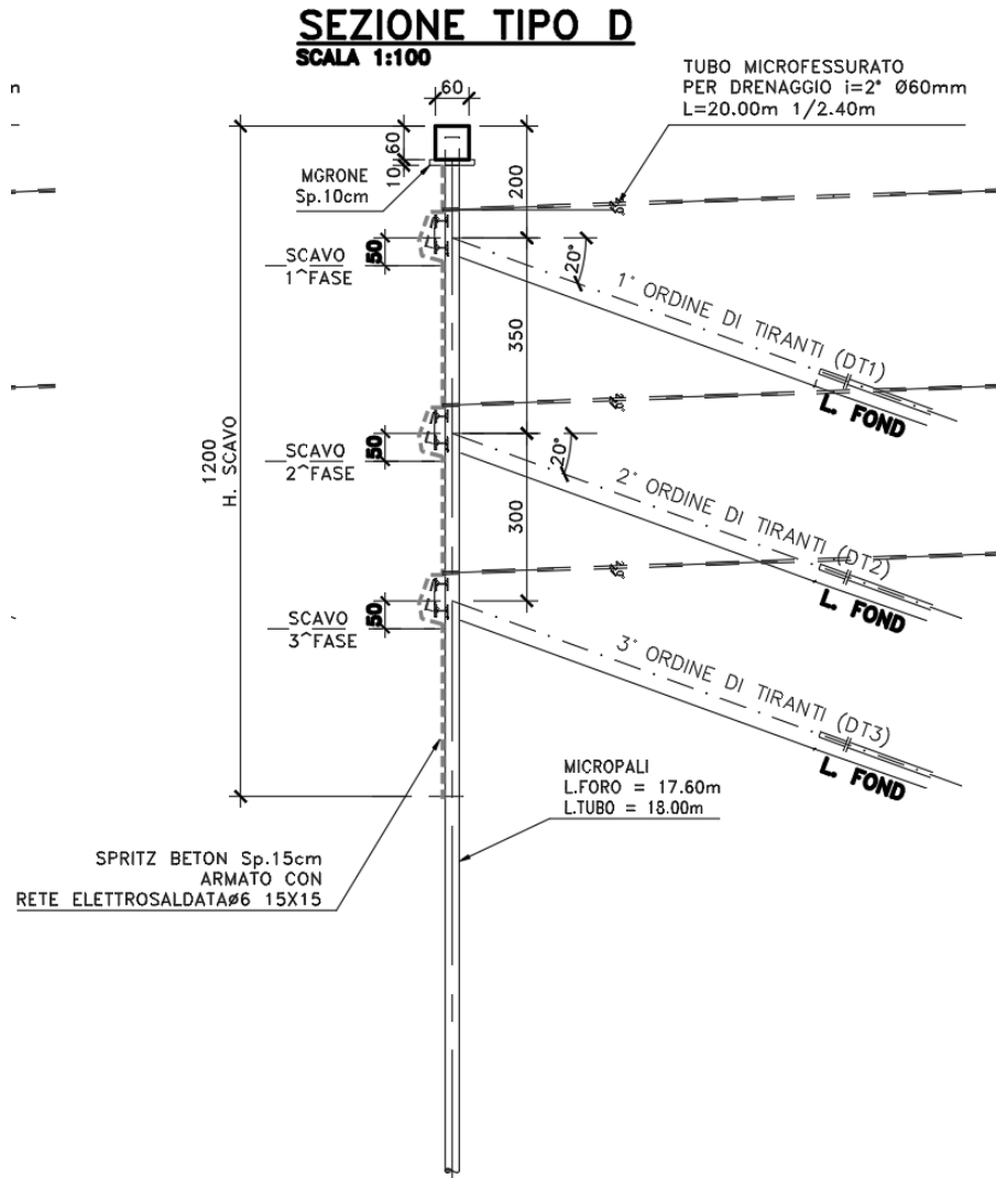
Figura 2.6 Sezione Paratia tipo D
