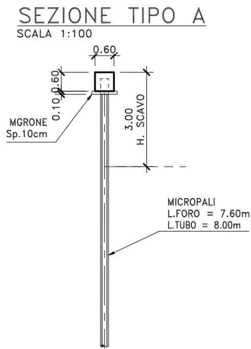
Figura 2.3 Sezione Paratia tipo A
