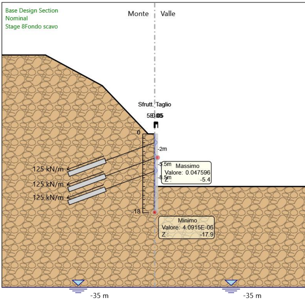
Involuppi Tasso di Sfruttamento a Taglio - SteelWorld
