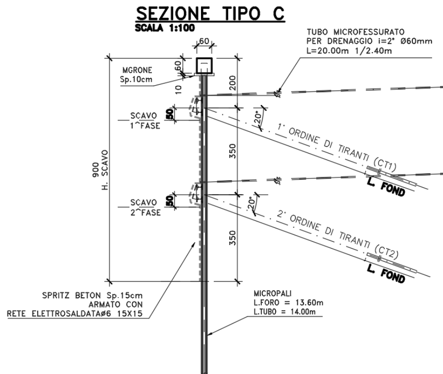
Figura 2.5 Sezione Paratia tipo C
