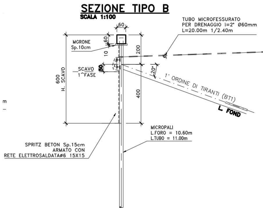
Figura 2.4 Sezione Paratia tipo B
