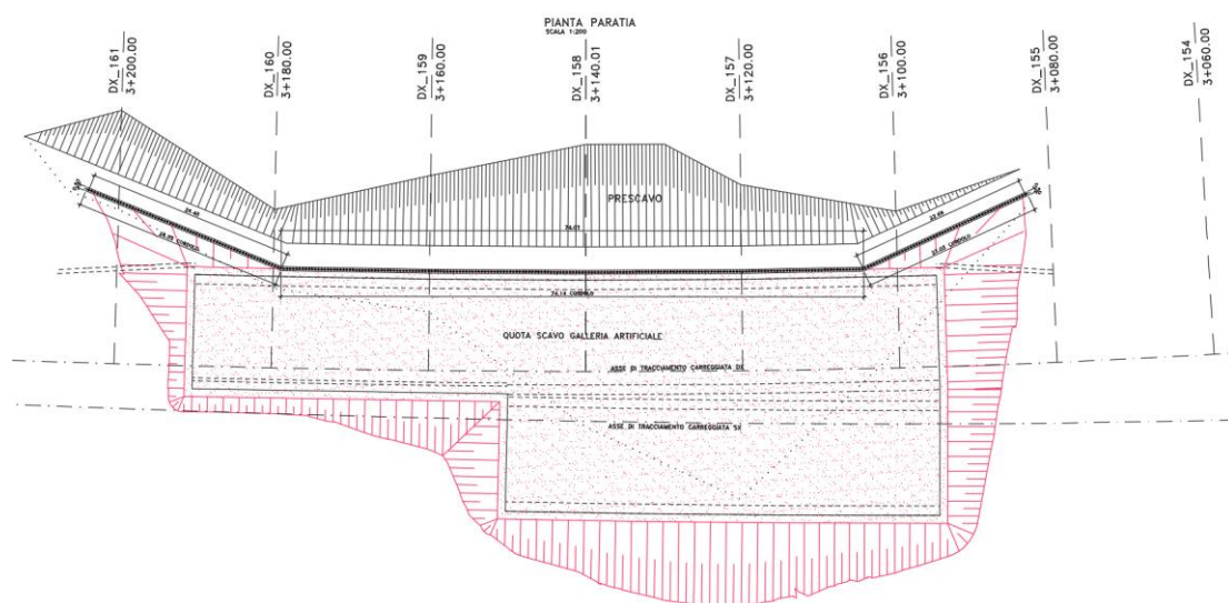
Figura 2.1 Pianta Paratia – Galleria artificiale GA01
