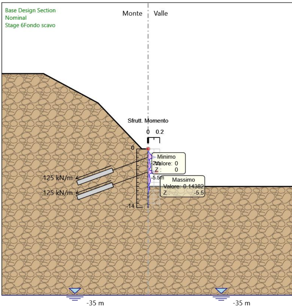
Grafico Inviluppi Tasso di Sfruttamento a Momento - SteelWorld
