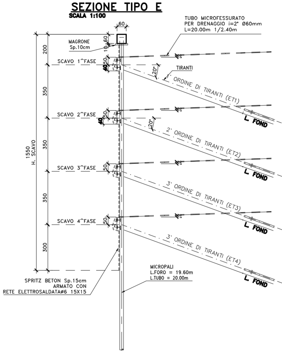
Figura 2.7 Sezione Paratia tipo E
