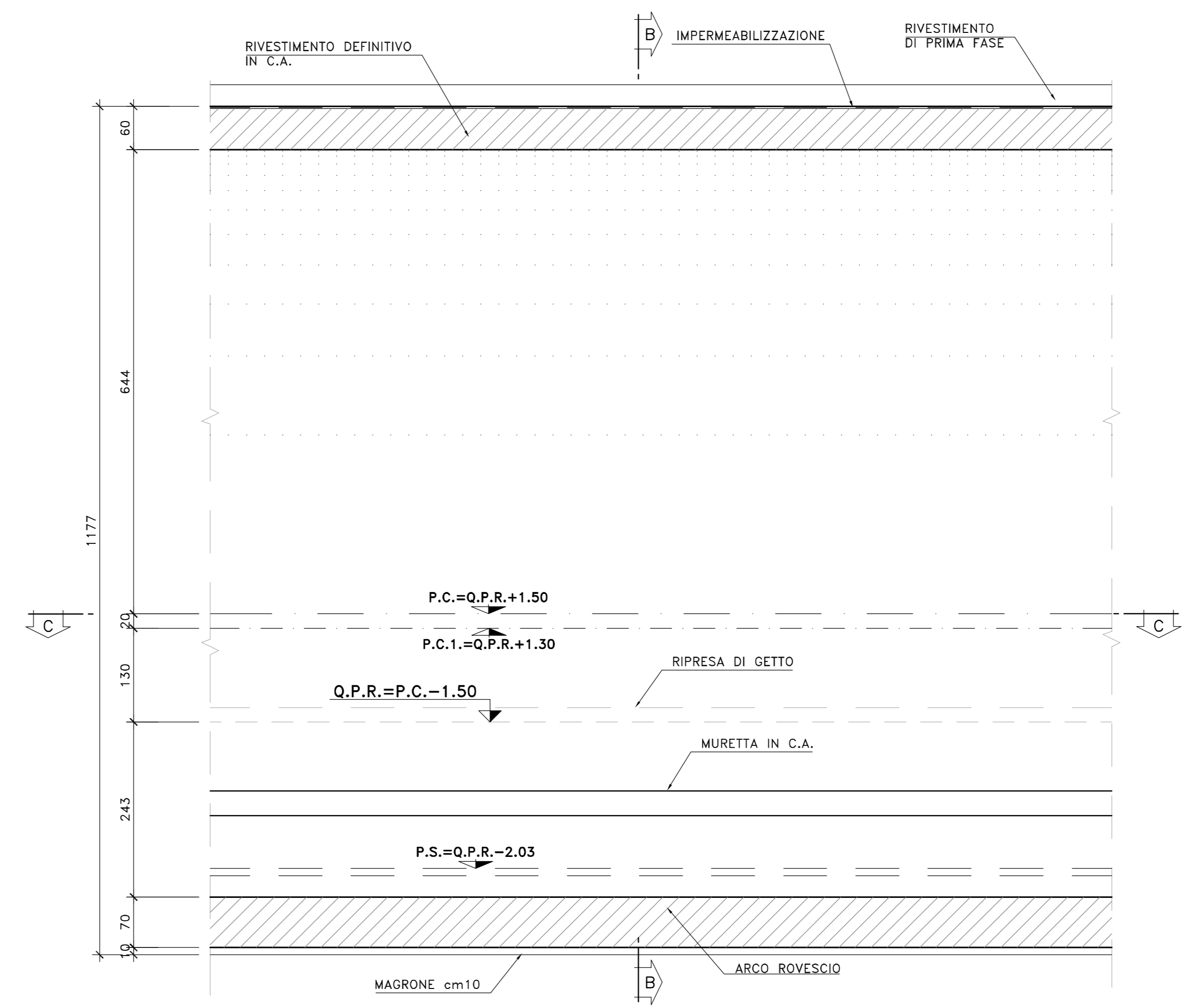
SEZIONE "A-A" PROFILO LONGITUDINALE Scala 1:50
