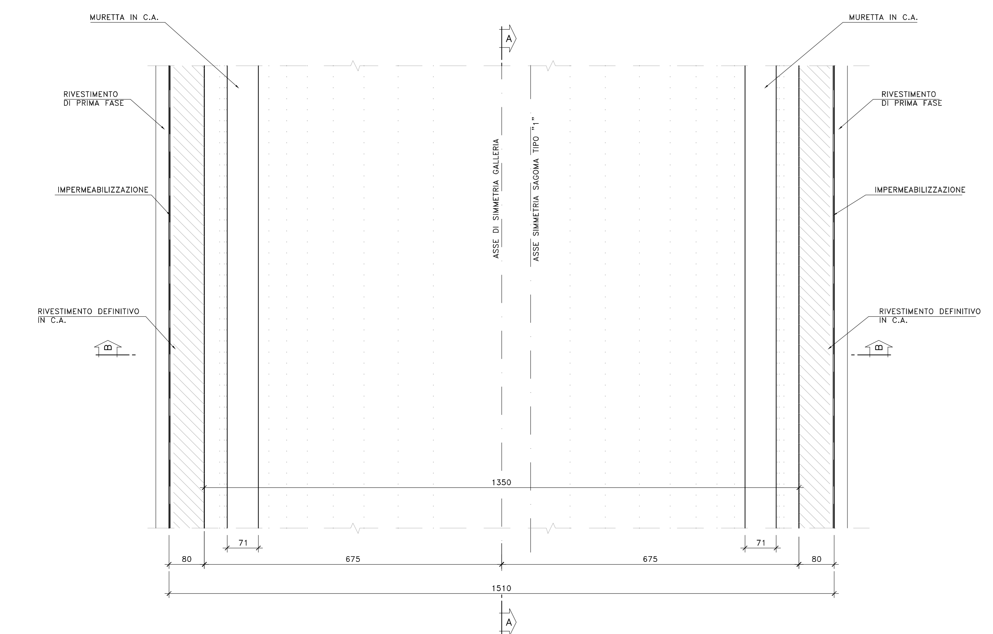
SEZIONE "C-C" PIANTA Scala 1:50
