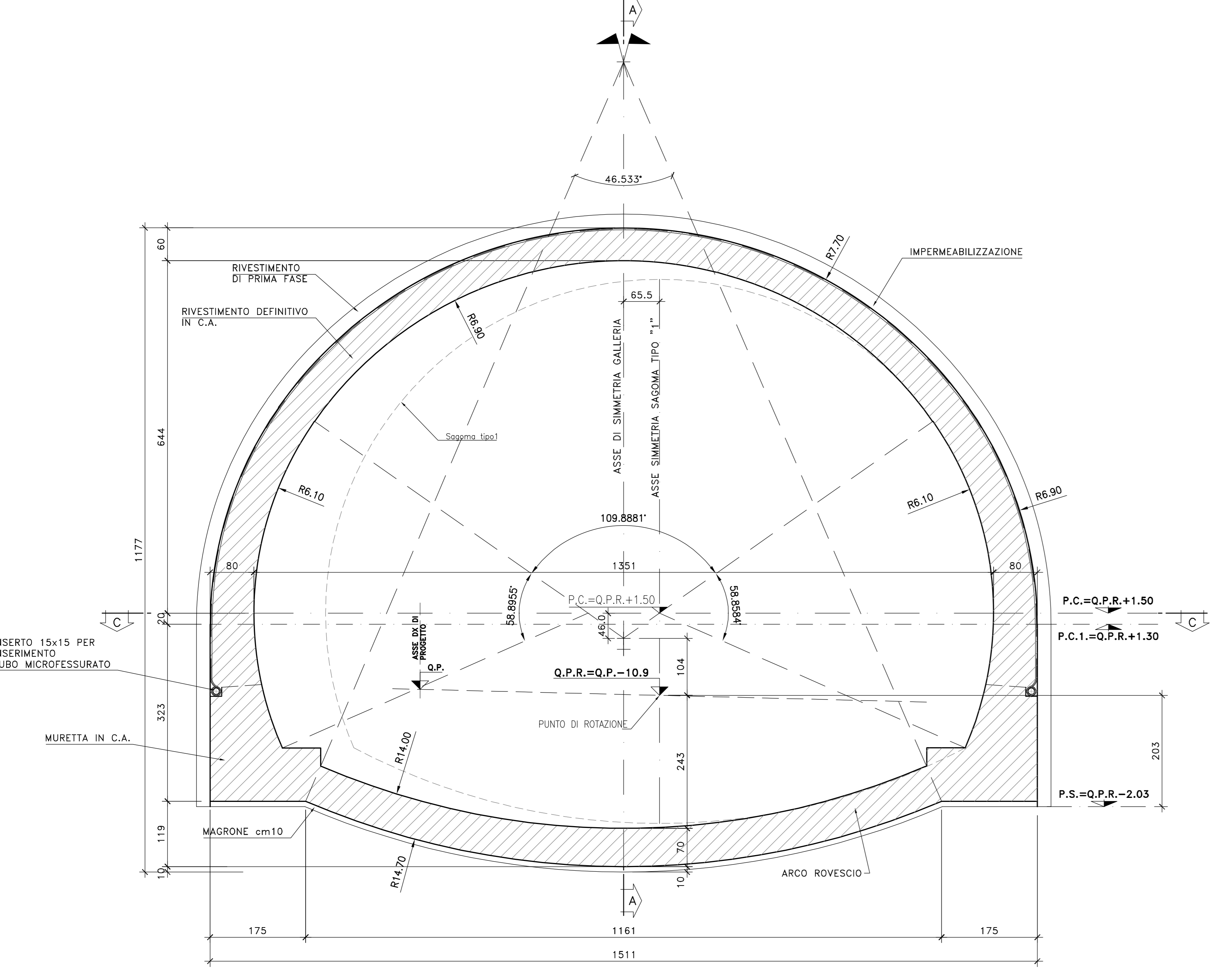
SEZIONE "B-B" Scala 1:50
