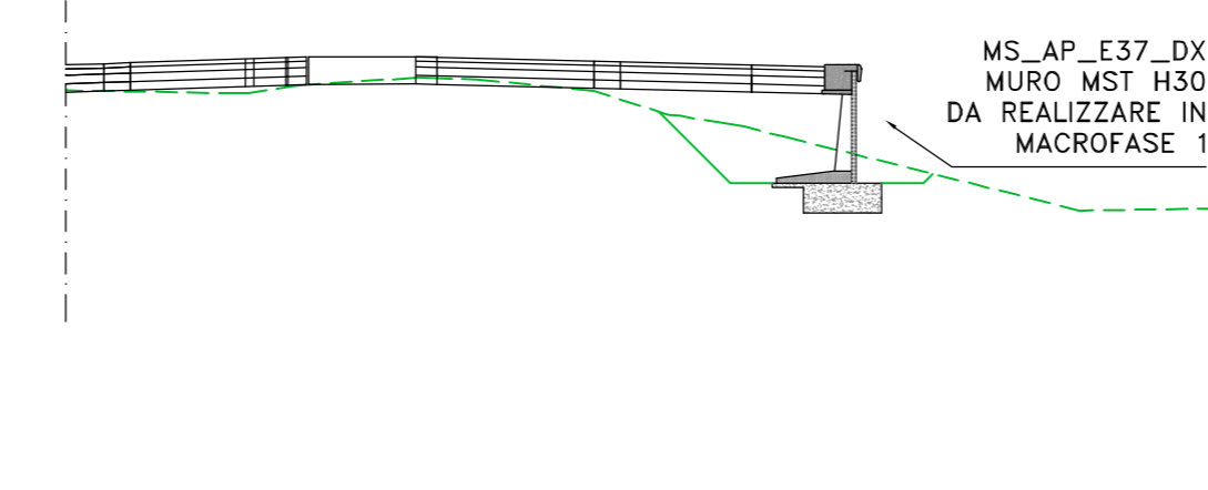
MS_AP_E37_DX Sez. DX_191 Progr.: 3+800,00 Scala : 1:200 Q.Rif. : 165,00
