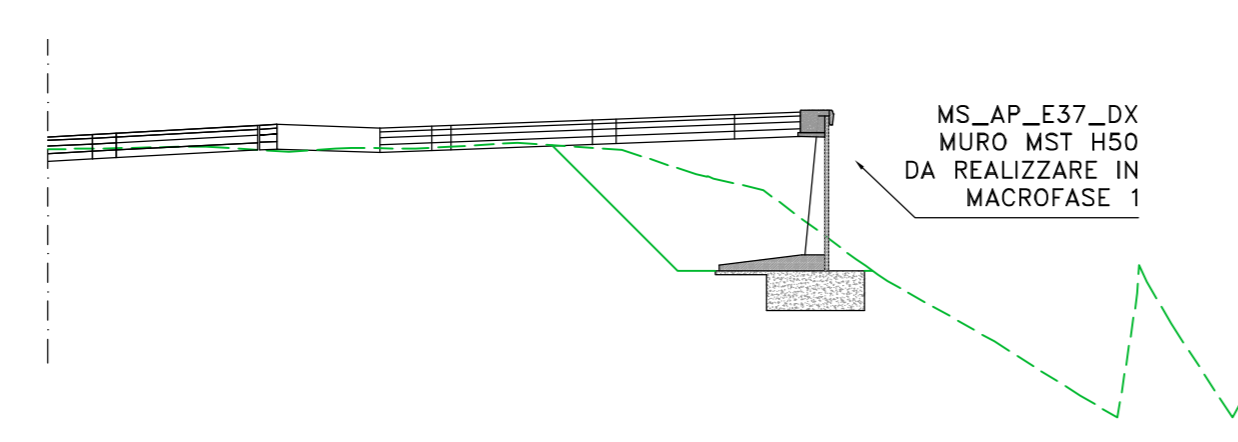
MS_AP_E37_DX Sez. DX_186 Progr.: 3+700,00 Scala : 1:200 Q.Rif. : 165,00
