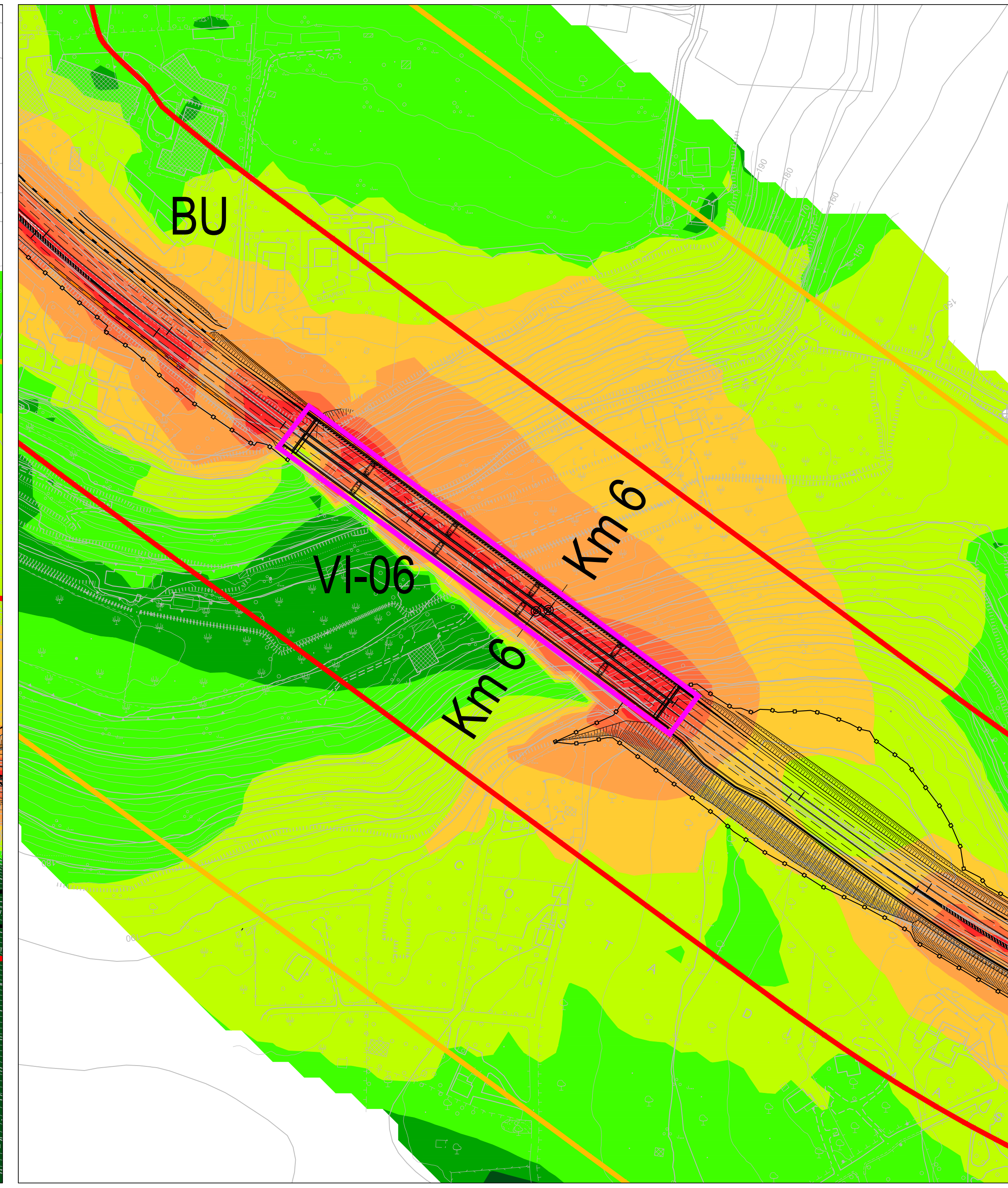
SIMULAZIONE ACUSTICA DEL CANTIERE LUNGOLINEA TIPOLOGICO VIADOTTO
