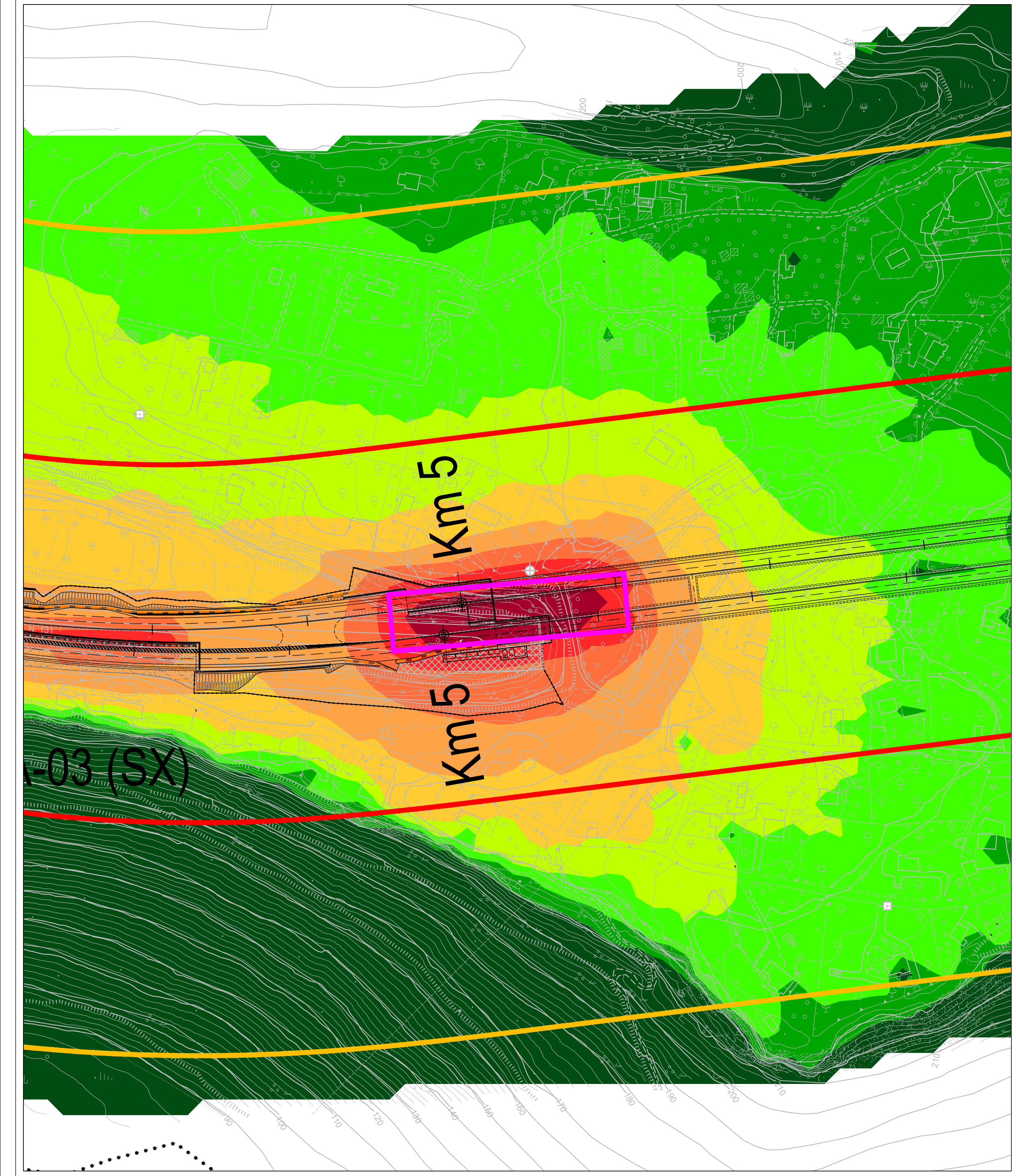
SIMULAZIONE ACUSTICA DEL CANTIERE LUNGOLINEA TIPOLOGICO GALLERIA
