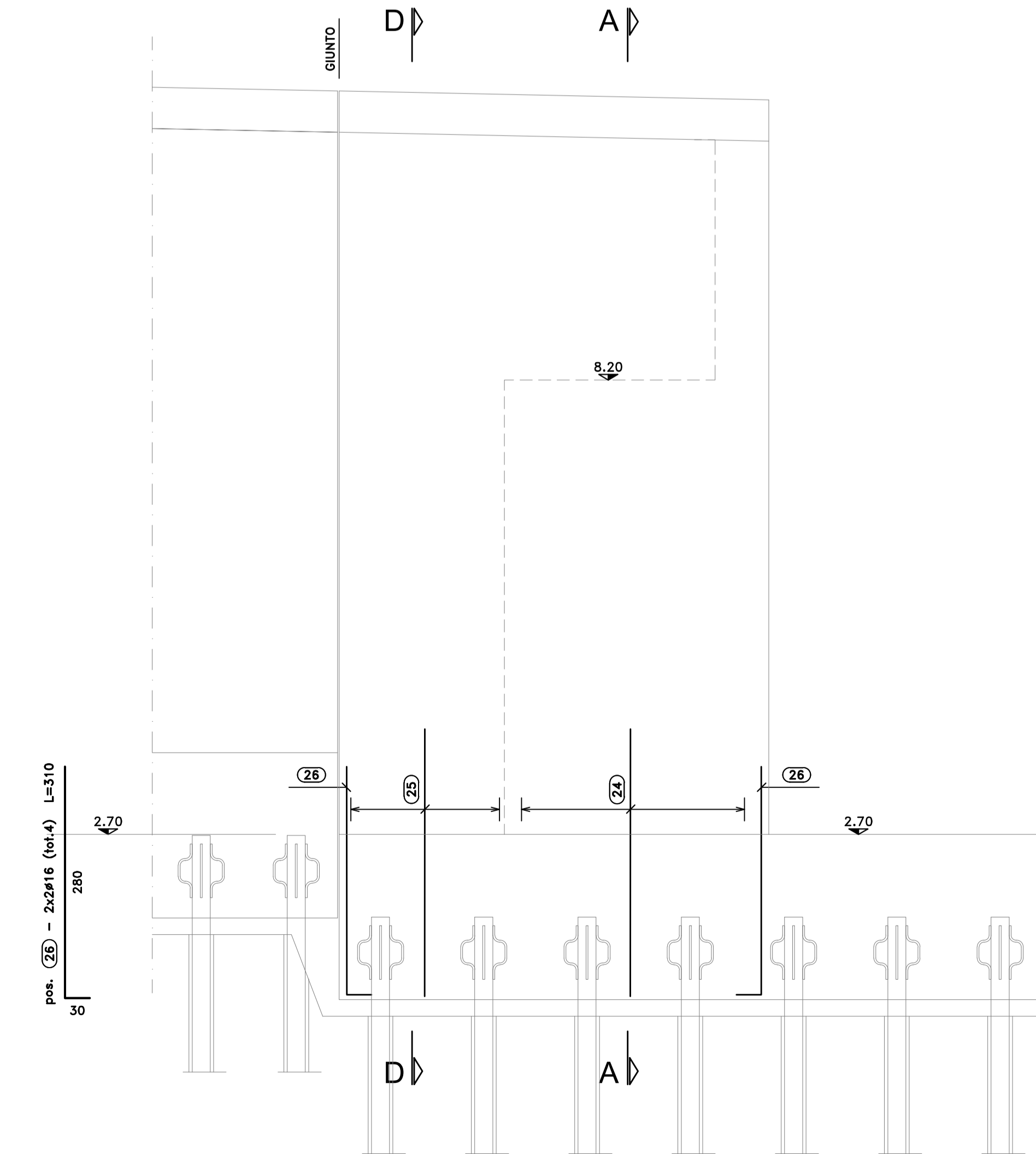
SEZIONE C-C SCALA 1:50
